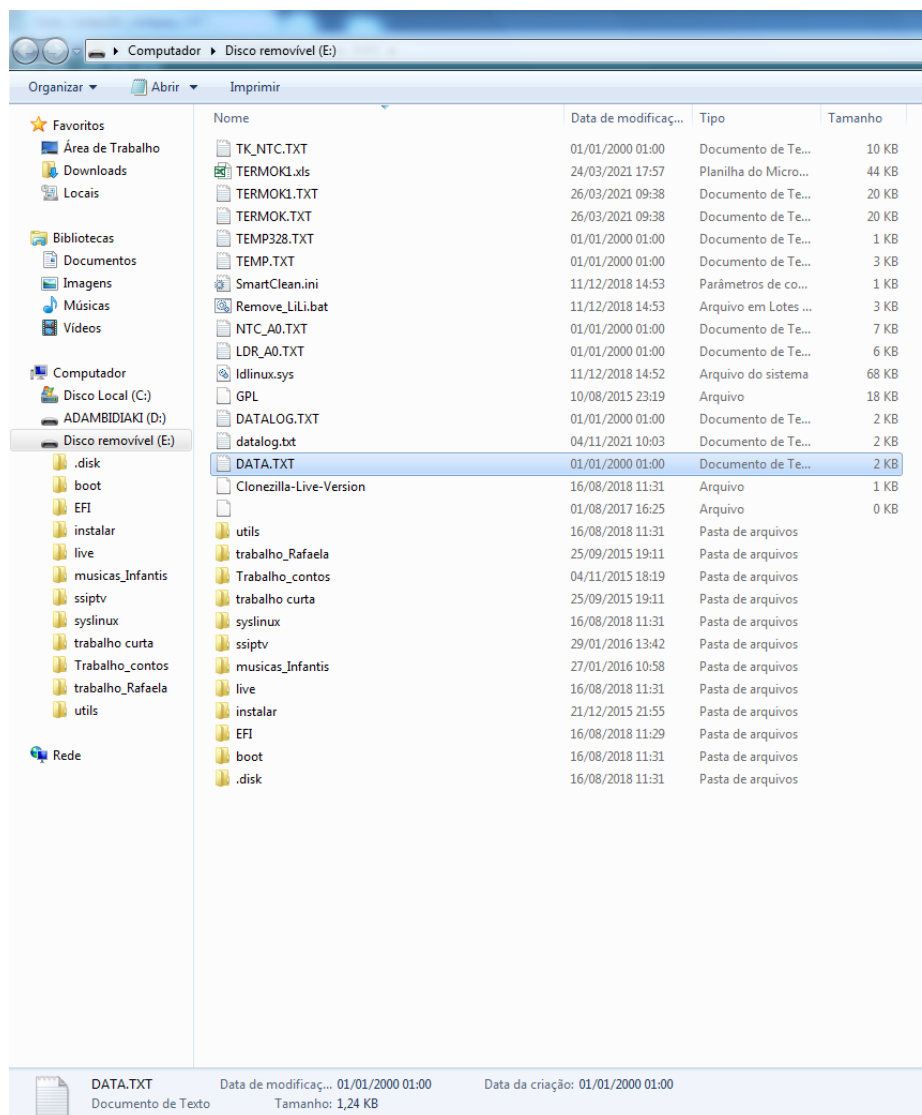
Figura 7: Arquivo DATA.TXT
