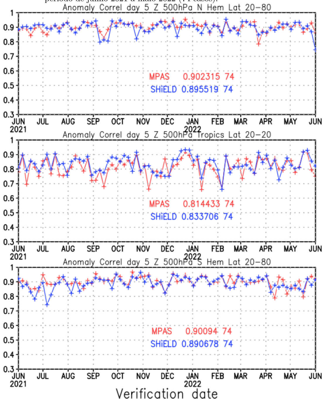
Figura 4.5 - Series temporais da ACC do geopotencial a 500 hPa dos modelos MPAS (vermelho) e SHiELD (azul), para o Hemisfério Norte (painel superior), trópicos (médio) e Hemisfério Sul (painel inferior). Previsões de 120 h (5 dias) para o período de junho 2021 a maio 2022 (74 casos).
