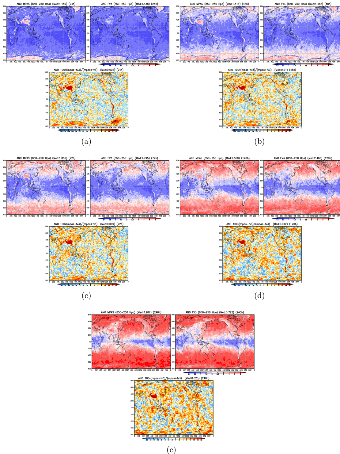
Figura 4.6 - Distância de MH para o MPAS e FV3 e diferença normalizada (DifMH) para os prazos de previsão de 24h (a), 48h (b), 72h (c), 120h (d) e 240h (e)
