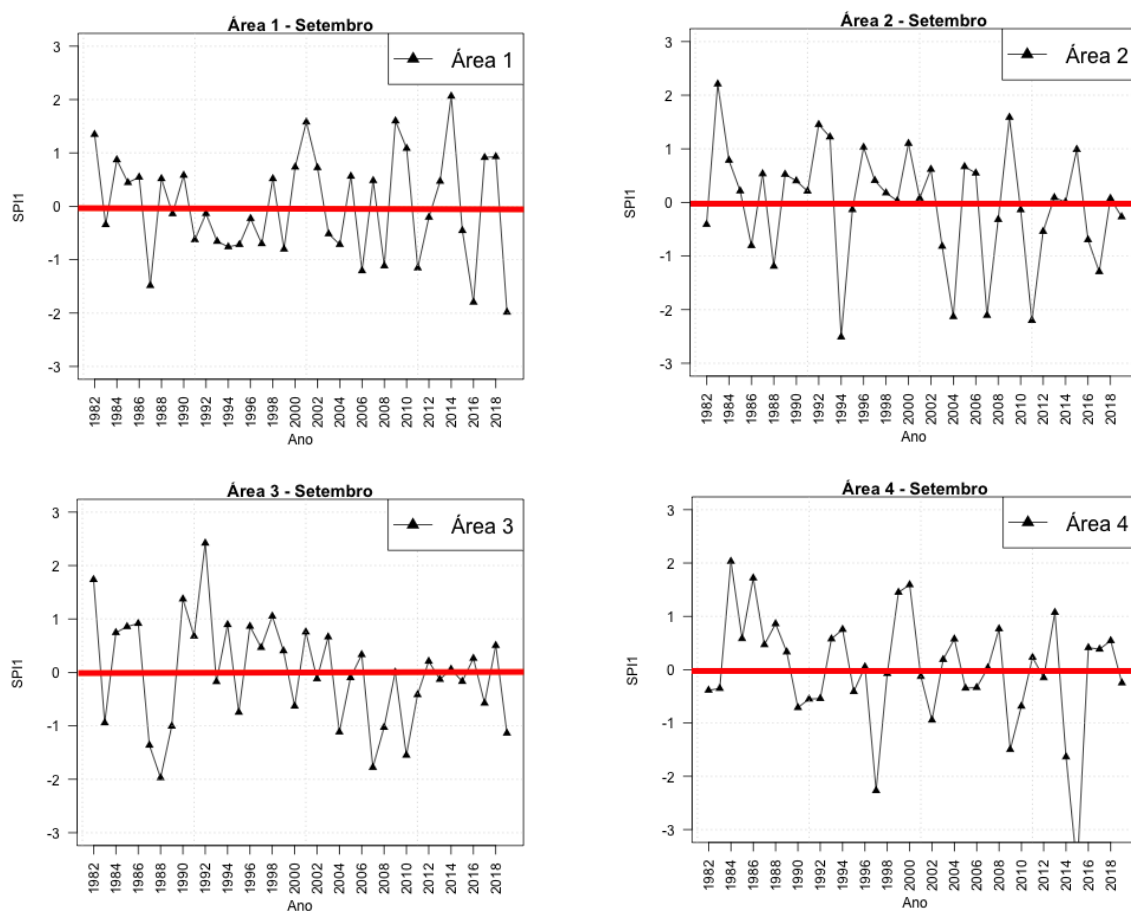
Figura 6.10 Séries temporais do SPI1 calculadas para o mês de setembro (1982-2019).
