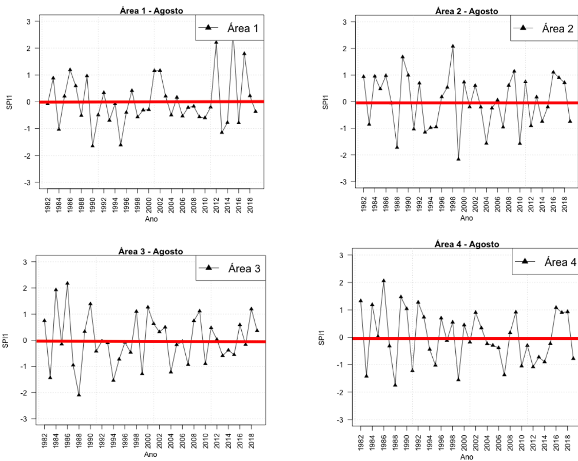
Figura 6.9 Séries temporais do SPI1 calculadas para o mês de agosto (1982-2019).
