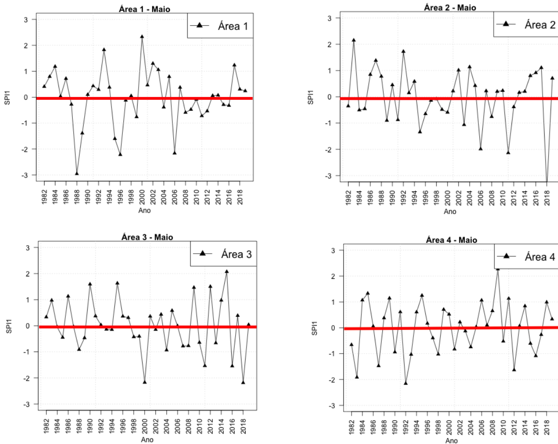
Figura 6.6 Séries temporais do SPI1 calculadas para o mês de maio (1982-2019).
