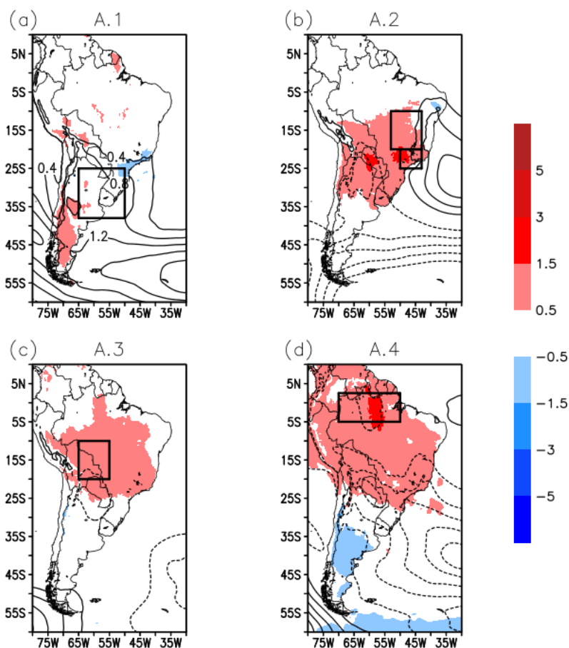
Compostos SON Anomalias Temperatura (°C) e PNMM (hPa)
