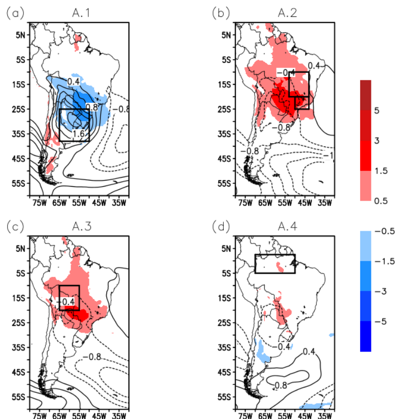
Figura 9.21 Compostos de anomalia de pressão a nível médio do mar (PNMM) e temperatura a 2 metros durante os meses de Setembro/Outubro/Novembro (SON), simulados pelo modelo HadGEM3 para os episódios de seca nas áreas homogêneas 1 (a), 2 (b), 3 (c) e 4 (d).
