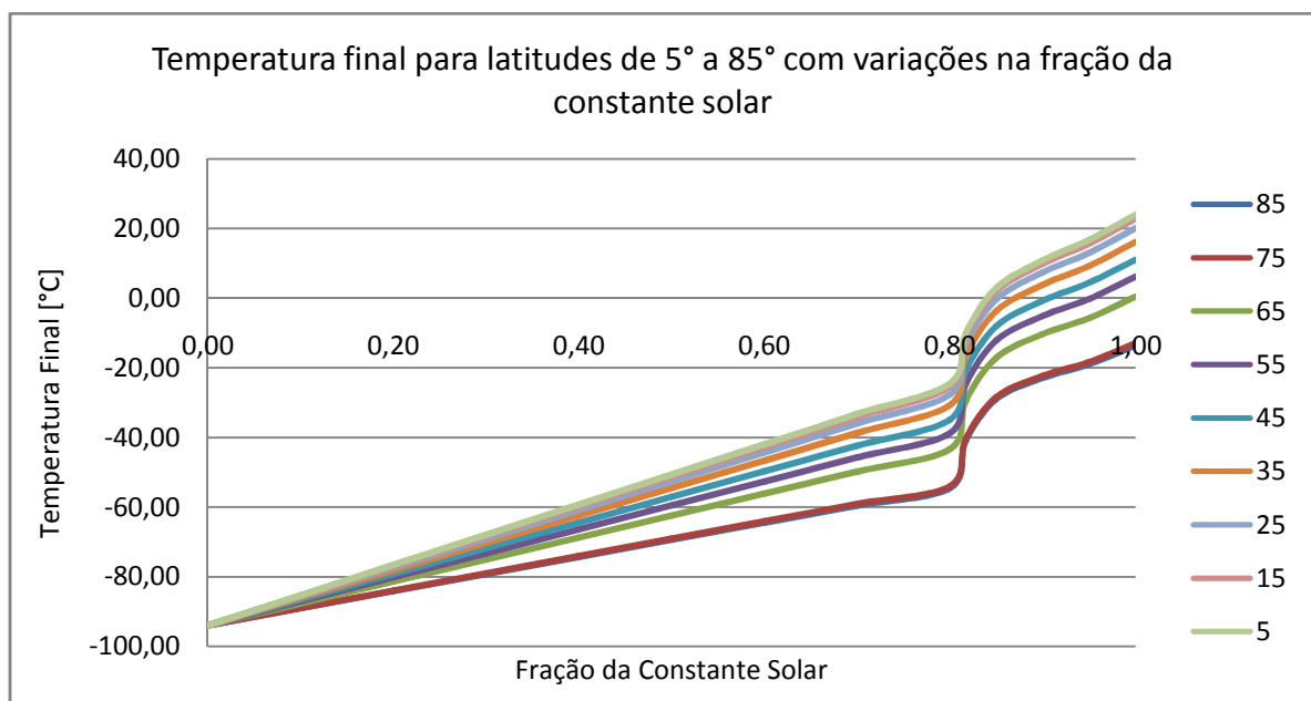
Figura 3: Temperatura final para latitudes de 5° a 85° com variações na fração da constante solar.
