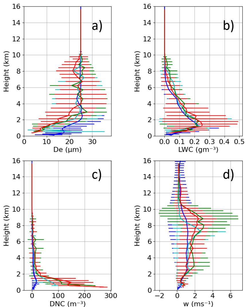
Figura 6.25 – Perfil vertical de De (a), LWC (b), DNC (c) e velocidade vertical (d) para nuvens associadas a diferentes concentrações de CCN em superfície. Curva azul CCN < 200 \text{ cm}^{-3} , curva ciano 200 \text{ cm}^{-3} < CCN < 450 \text{ cm}^{-3} , curva verde 450 \text{ cm}^{-3} < CCN < 800 \text{ cm}^{-3} e vermelho CCN > 800 \text{ cm}^{-3} .
