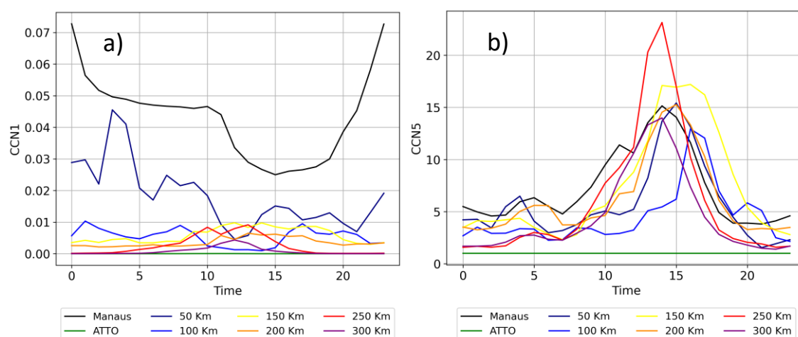
Figura 6.19 - Razão entre a concentração média de CCN para as distancias de 50, 100, 150, 200, 250 e 300 km de Manaus pela concentração de CCN no local ATTO em função da hora ao longo do dia 13/03 para a supersaturação de 0,02% (a) e 0,5% (b).
