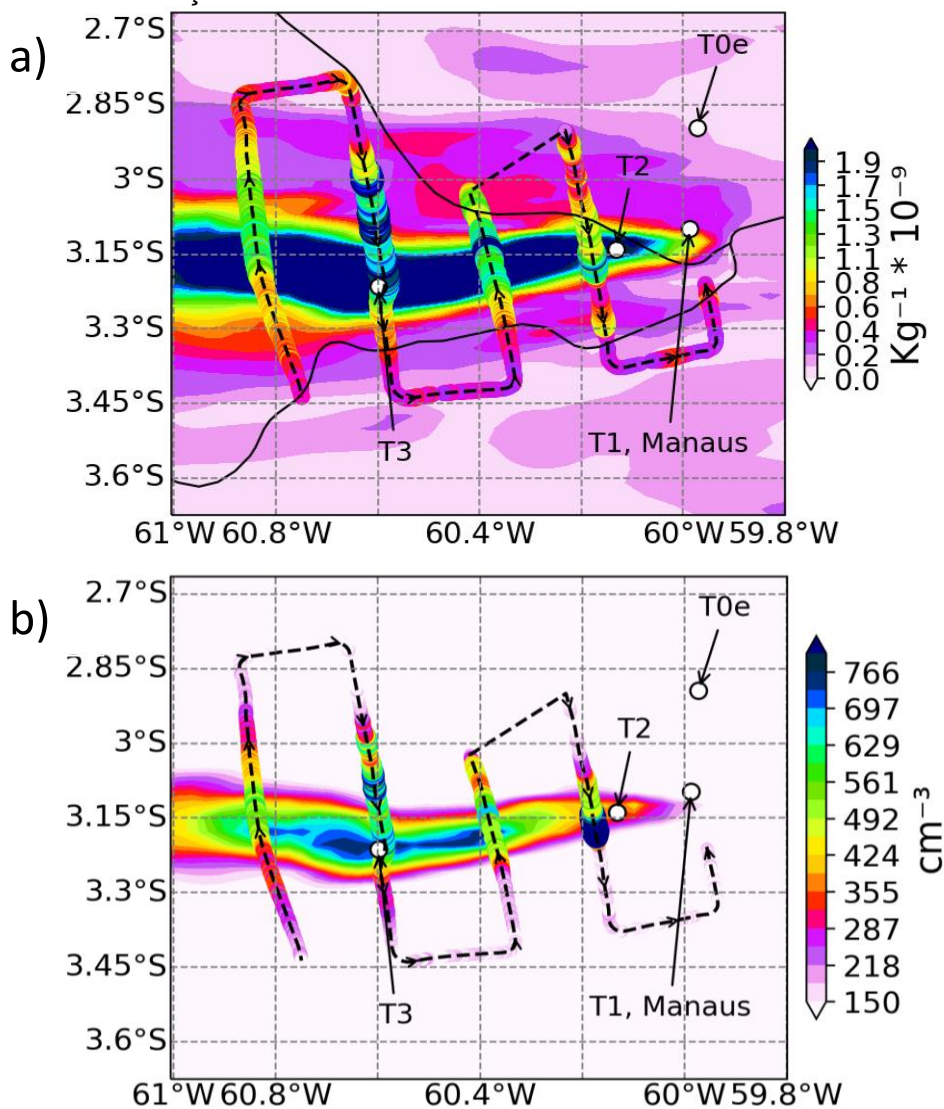
Figura 6.10 - Concentração de aerossol na moda de acumulação (a) e CCN (b). O mapa de fundo representa as concentrações observadas e os marcadores na mesma paleta de cor do mapa de fundo ao entorno da linha pontilhada representam as concentrações de aerossol e CCN extraídos das observações. As setas indicam o sentido do voo.
