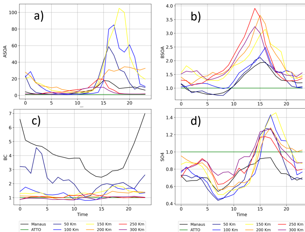
Figura 6.15 – Razão entre a concentração média de aerossol a) ASOA, b) BSOA, c) BC e d) \text{SO}_4^{2-} pela concentração média de aerossol no local ATTO em função da hora em Manaus, ao longo da pluma para as distancias de 50, 100, 150, 200, 250 e 300 km de Manaus e no ATTO.
