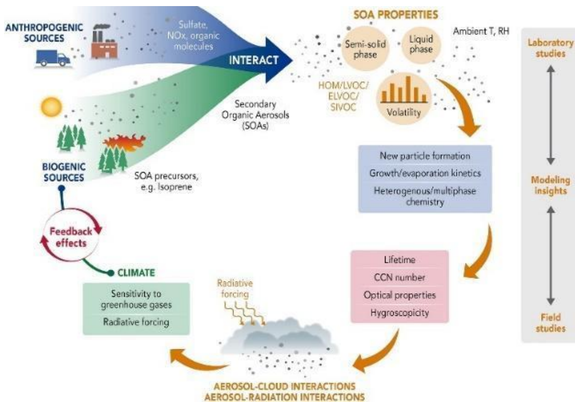
Figura 4.4- Ilustração dos processos que regem a importância climática de SOA. É mostrado as principais fontes de VOC, propriedades dos aerossóis relacionadas a formação e crescimento das partículas, nucleação de nuvens e uma possível resposta para o sistema climático.
