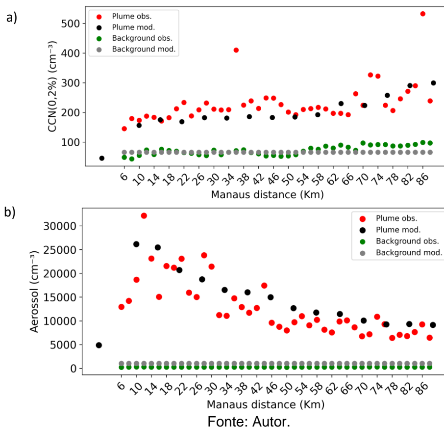
Figura 6.12 - Concentrações médias de a) aerossóis e b) CCN observado (background – verde e na pluma - vermelho) e modelado (background – cinza e na pluma - preto). O CCN observado corresponde a SS de 0,23 % e o modelado a SS de 0,2 %. As concentrações foram calculadas em relação à distância de Manaus.
