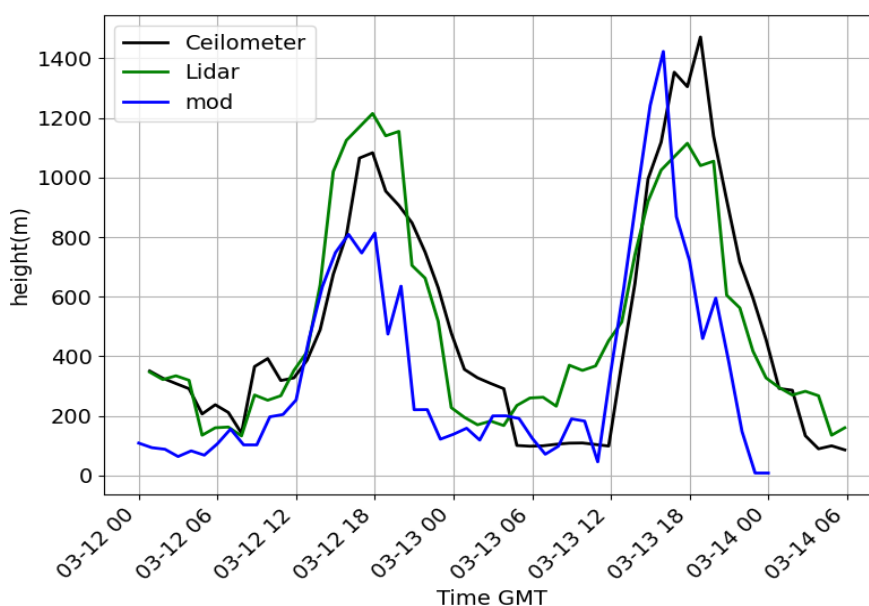
Figura 6.5 - CLP observada e modelada ao longo dos dias 12 e 13 de março de 2014.
