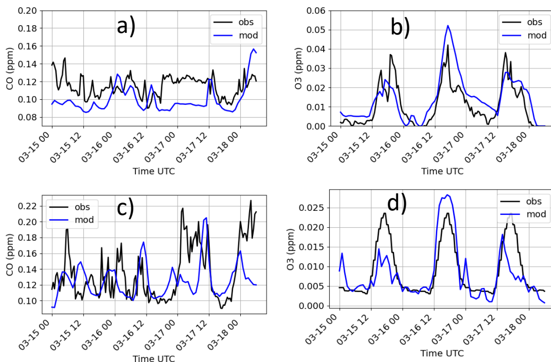
Figura A.3 – Comparação entre os dados observados e modelados. Os gráficos a) e b) são referentes a concentração de CO e O3 respectivamente para o local e os gráficos c) e d) para CO e O3 no local.
