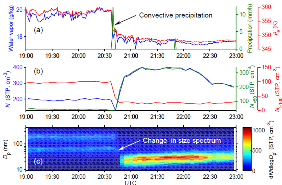
Figura 4.11 - Dados do experimento GoAmazon mostrando o efeito da convecção na concentração de aerossol.
