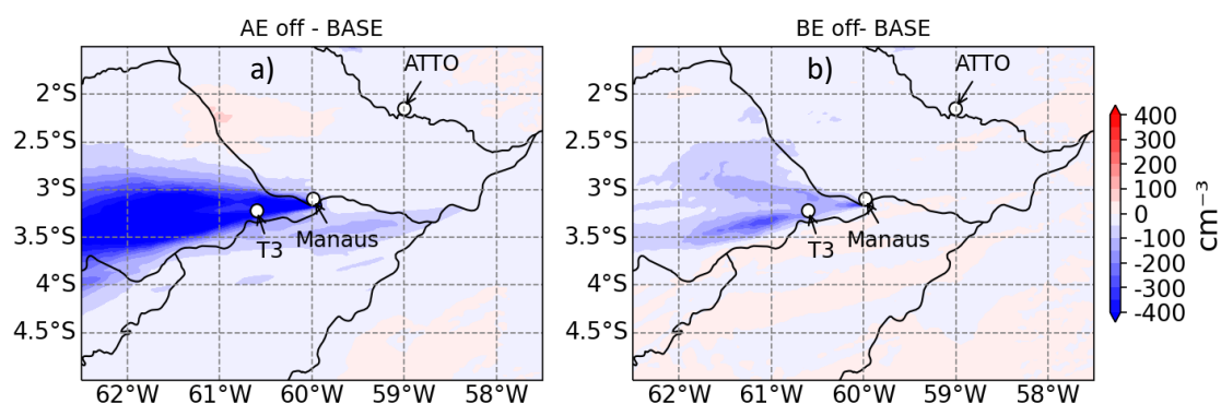
Figura 6.27 - diferença entre a concentração de CCN média entre os dias 16 e 17 de março a) AE off – Base, b) BE off – Base.
