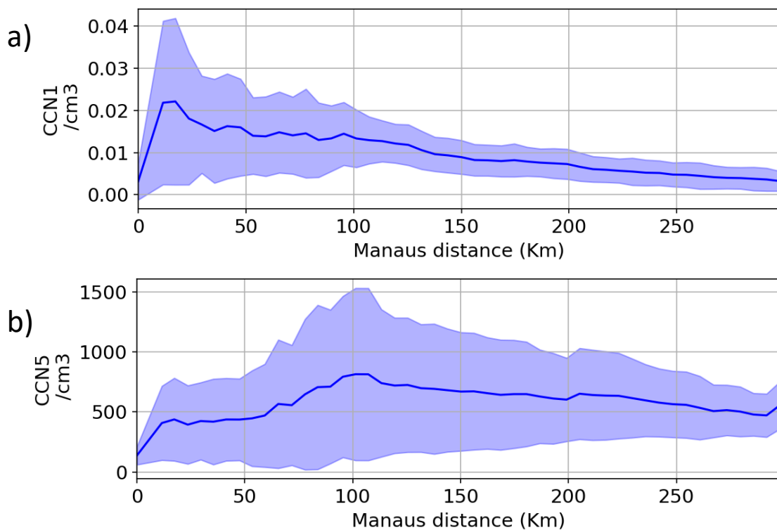
Figura 6.18 - Concentração de CCN simulada média em função da distância de Manaus para o dia 13/03 e supersaturação de 0,01% (a) e 0,5% (b). A região hachurada em cada figura representa o intervalo de + ou - 1 desvio padrão.
