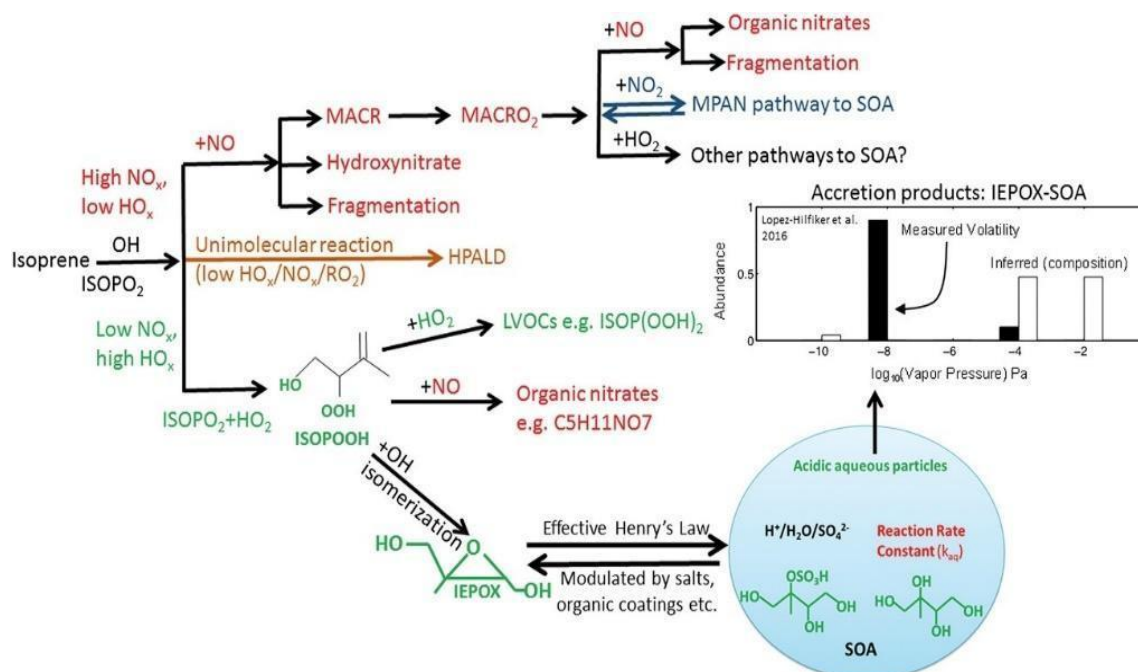
Figura 4.2 - Destino dos radicais de isopreno (ISOPO) e as diferentes vias químicas que dependem dos regimes de NO, HO e RO.
