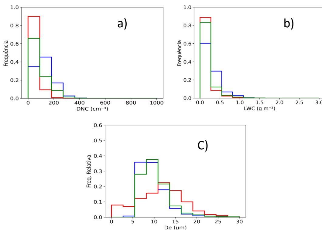
Figura 6.29 - Histograma de frequência para o a) DNC, b) LWC e c) De derivado dos experimentos AE off (linha vermelha), BE off (linha verde) e Base (linha azul) entre os dias 16 e 17 de março.
