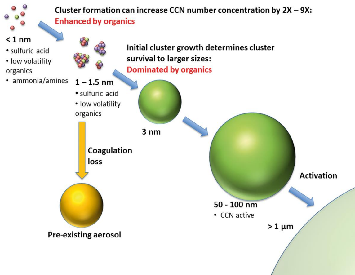
Figura 4.3 - Esquema ilustrando a partição de produtos de oxidação e o crescimento dos aglomerados recém-formados para tamanhos CCN-ativos ou a coagulação com o aerossol preexistente.
