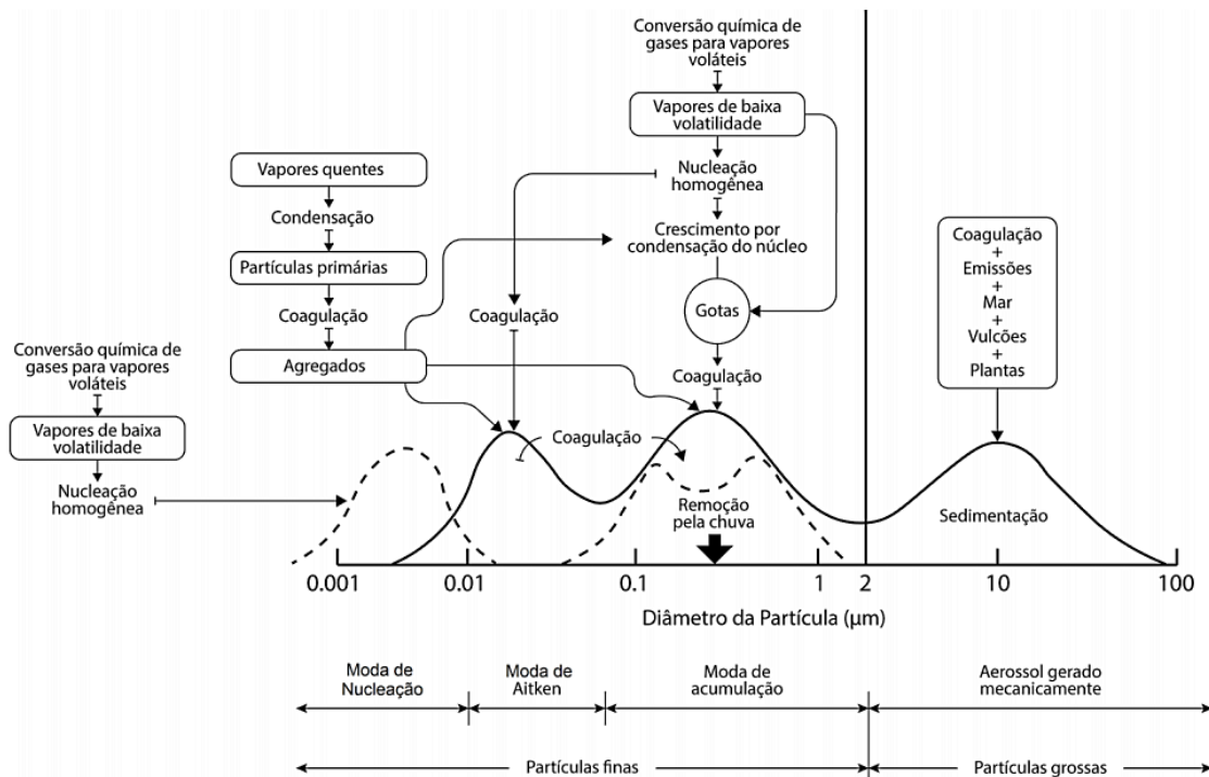
Figura 4.1 - Esquema da distribuição de tamanhos dos aerossóis atmosféricos e os processos que influenciam cada fração de tamanho das partículas. A linha sólida é a clássica hipótese de Whitby e colaboradores, e a moda mais à esquerda representada pela linha pontilhada é referente à moda de nucleação.
