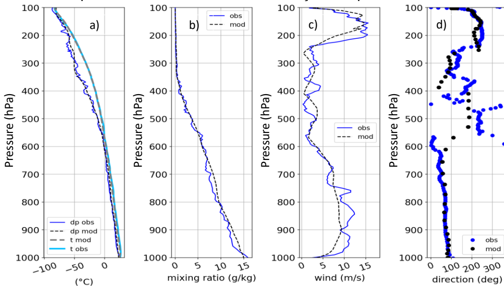
Figura 6.4 - Variação de a) temperatura (Temperatura do ponto de orvalho e temperatura do ar) b) razão de mistura e c) intensidade e d) direção do vento modelado (linha tracejada preta) e observado (linha contínua azul). As observações são provenientes das radiossondas lançadas a partir do site T3.
