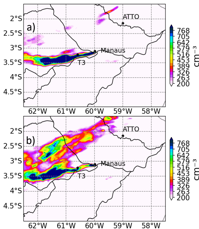
Figura 6.21 - Concentração de CCN a) às 12:00 e b) as 15:00 do dia 17 de março para o nível do modelo.
