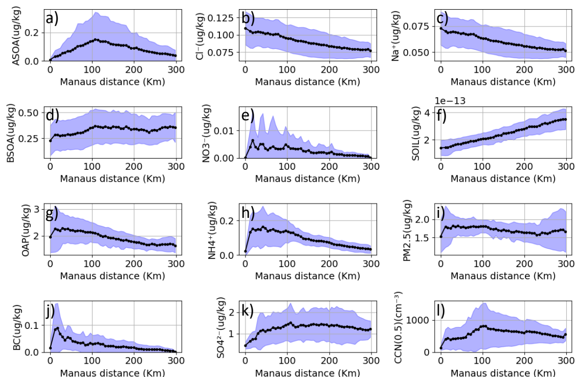
Figura 6.14 - Concentração média de a) ASOA, b) aerossol de cloreto ( \text{Cl}^- ), c) sódio ( \text{Na}^+ ), d) BSOA, e) nitrato ( \text{NO}_3^- ), f) SOIL, g) aerossol orgânico primário (OAP), h) amônia ( \text{NH}_4^+ ), i) \text{PM}_{2.5} não especificado, j) Black Carbon (BC), k) sulfato ( \text{SO}_4^{2-} ) e l) CCN ( \text{SS}=0,5\% ), no dia 13/03 ao longo da pluma. A região hachurada em cada figura representa o intervalo de + ou - 1 desvio padrão.
