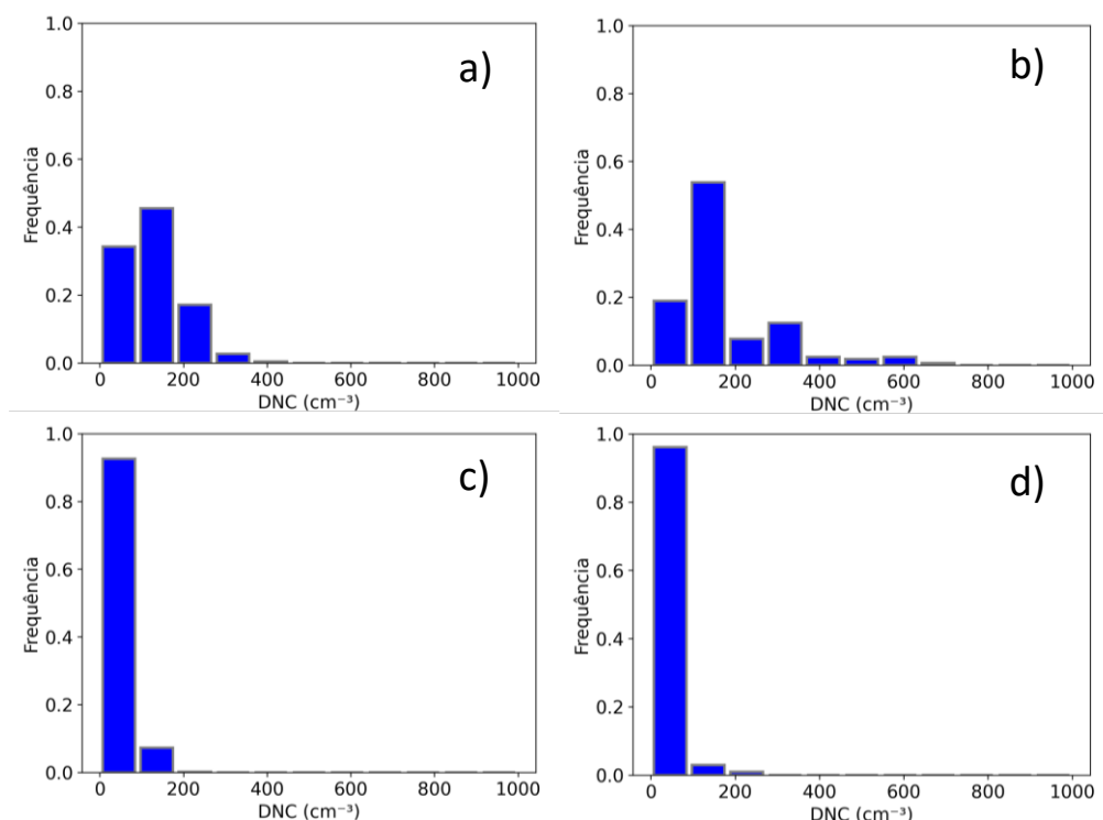
Figura 6.22 - Histograma de frequência do DNC derivado dos dados do modelo, sob ação da pluma (a) e condição de background (c), abaixo da isoterma de 0°C entre os dias 16 e 17 de março (coluna a esquerda) e extraídos dos dados observados (coluna a direita), sob ação da pluma (b) e condição de background (d).
