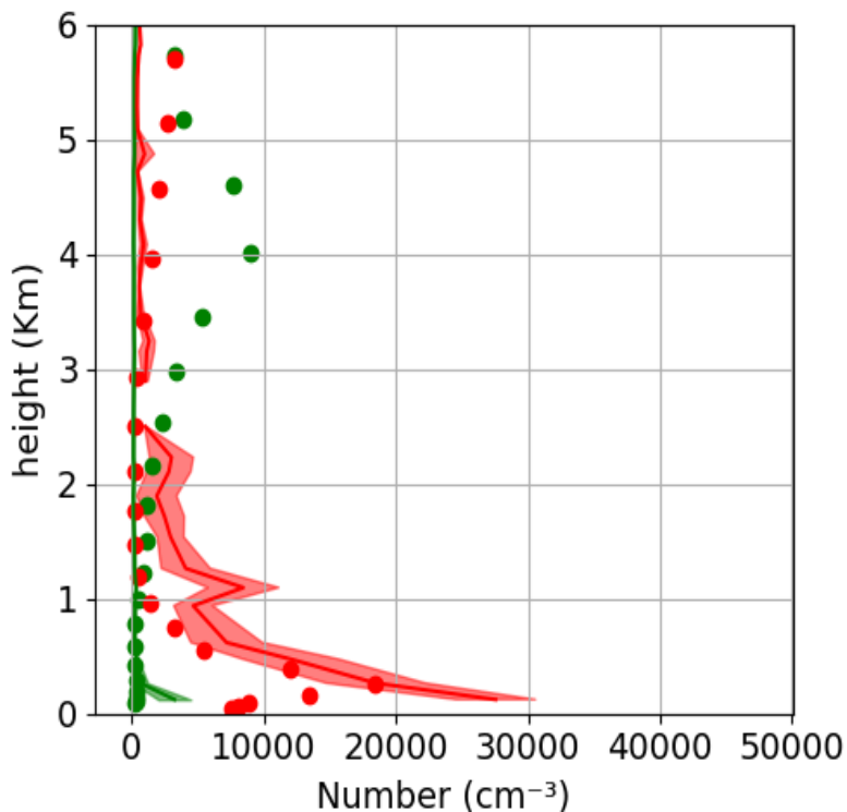
Figura 6.9 - Perfil médio de aerossol extraídos de todos os voos realizados no mês de março de 2014 e modelados (média dos dias 12 e 13 de março). Em cada gráfico as cores vermelhas (verdes) representam as concentrações associadas à pluma (fora da pluma). Os pontos vermelhos (verde) são os dados do modelo extraídos no local T3 (ATTO).
