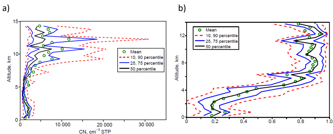
Figura 4.9 - Perfil vertical médio da concentração de aerossol de todos os voos realizados com o avião HALO durante o experimento GoAmazon e b) Partículas com diâmetro menor que 90 nm.
