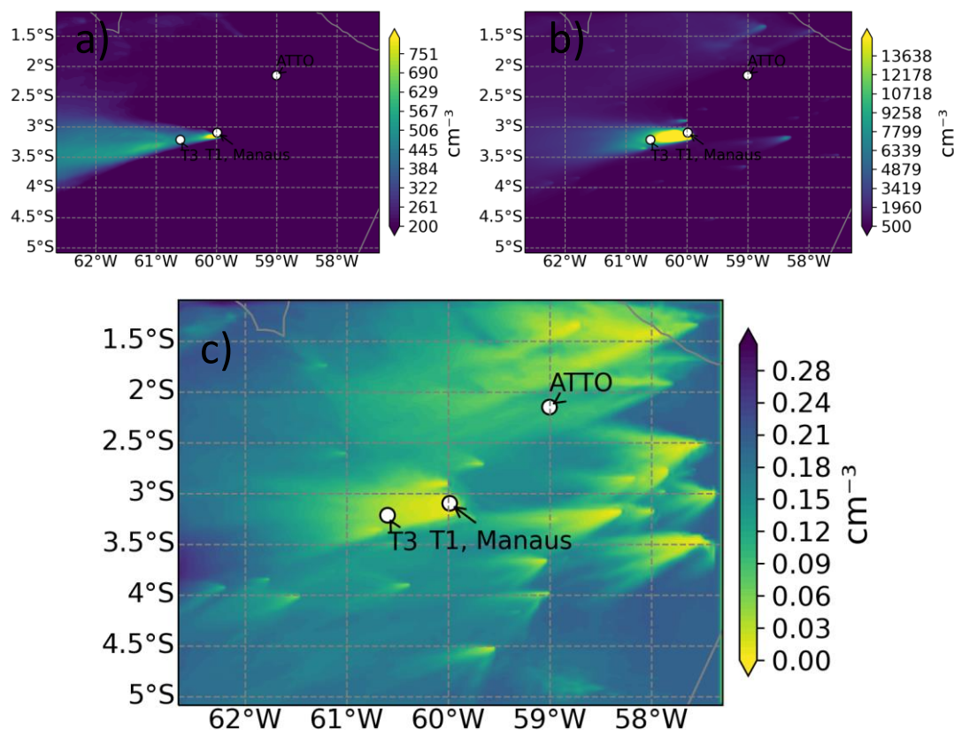
Figura 6.20 - Concentração média (entre os dias 16 e 17) dos primeiros 8 níveis do modelo para as concentrações de a) CCN, b) Aerossol e c) relação CCN/aerossol.
