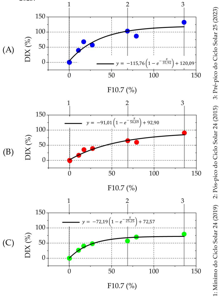
Figura 6.2 – Gráficos de dispersão que ilustram a relação entre as taxas de variação percentual das médias anuais do F10.7 e do DIX durante EPBs em relação ao mínimo solar ocorrido entre os ciclos solares 24 e 25, para os meridianos oeste (A), central (B) e leste (C). As linhas verticais indicam etapas específicas dos ciclos solares: ‘1’ representa o mínimo de atividade solar em 2019, ‘2’ representa a fase pós-pico do ciclo solar 24 em 2015 e ‘3’ representa a fase pré-pico do ciclo solar 25 em 2023.
