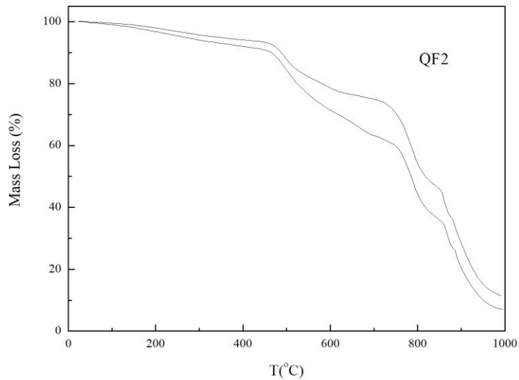
Figura 6 – TG da amostra QF2
