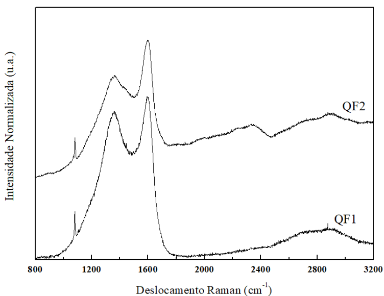
Figura 4 – Deslocamento de Raman do QF1 e QF2
