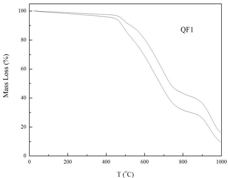
Figura 5 – TG da amostra QF1
