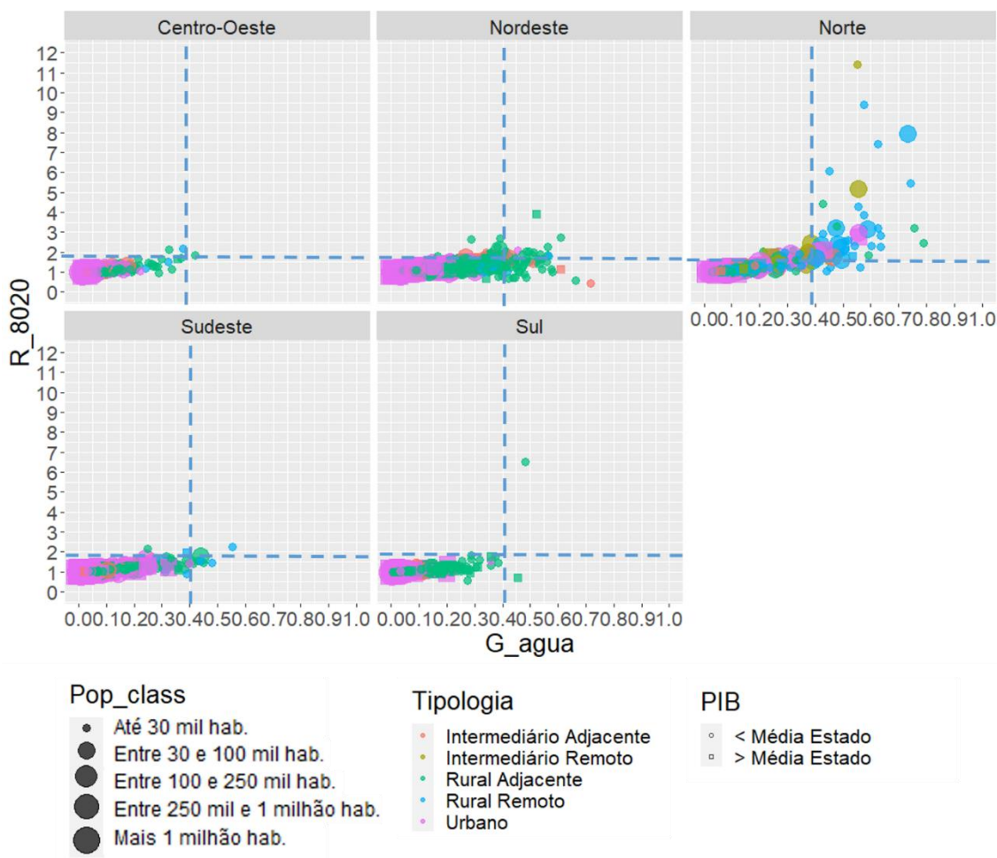
Figura 4.30 – Relações gráficas entre os resultados de G_{\text{água}} e R_{80/20} dos municípios por Região do Brasil, considerando população, tipologia e PIB per capita .
