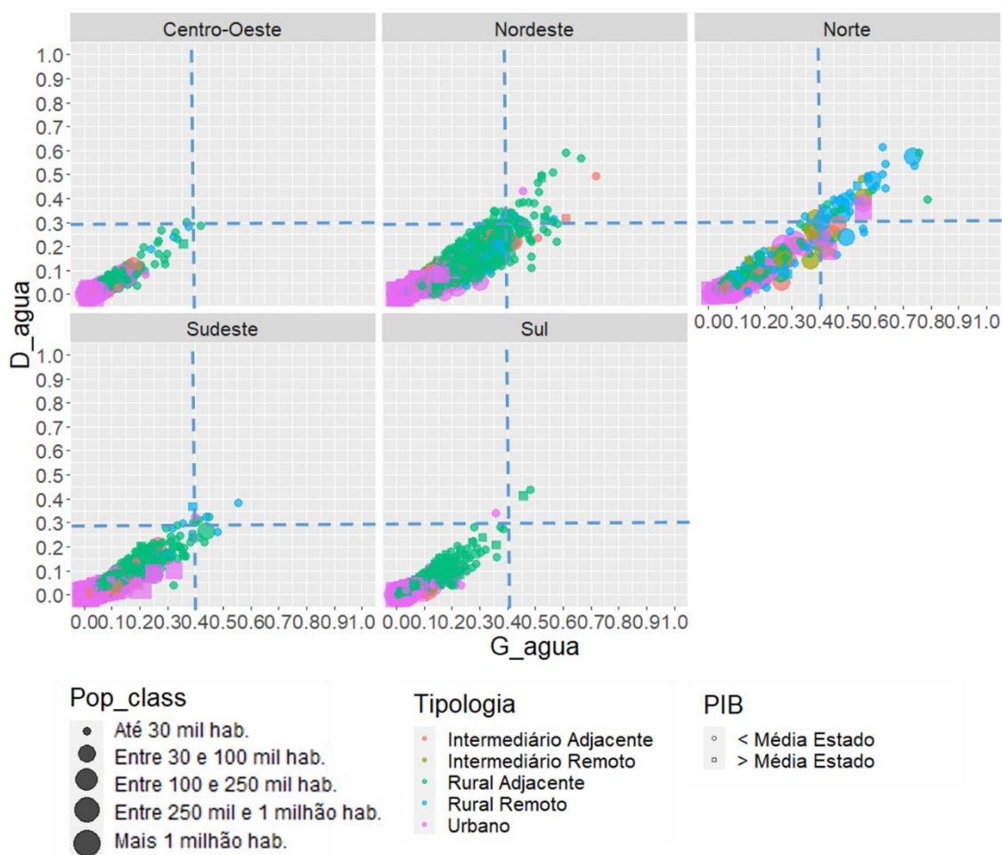
Figura 4.28 – Relações gráficas entre os resultados de G_{\text{água}} e D_{\text{água}} dos municípios por Região do Brasil, considerando população, tipologia e PIB per capita .
