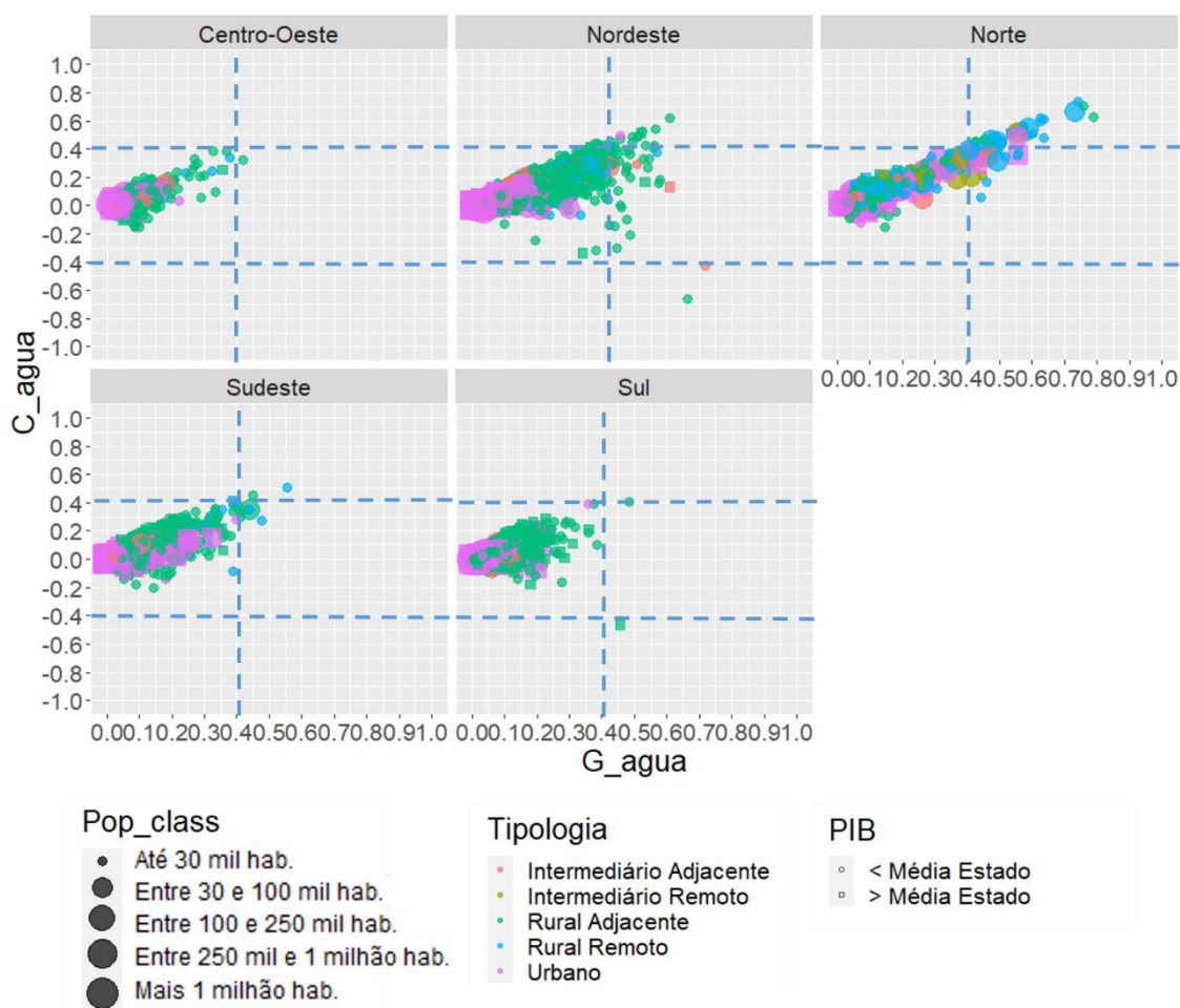
Figura 4.29 – Relações gráficas entre os resultados de G_{\text{água}} e C_{\text{água}} dos municípios por Região do Brasil, considerando população, tipologia e PIB per capita .
