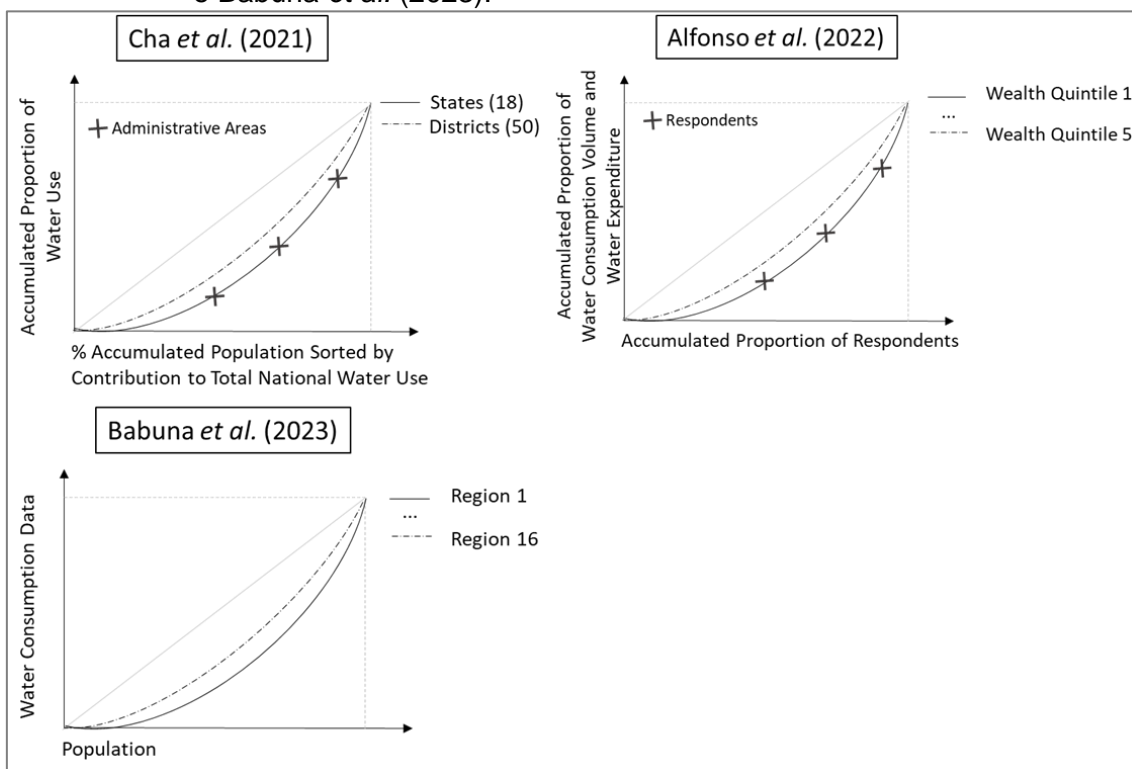
Figura 2.10 – Curvas de Lorenz adaptadas por Cha et al. (2021), Alfonso et al. (2022) e Babuna et al. (2023).
