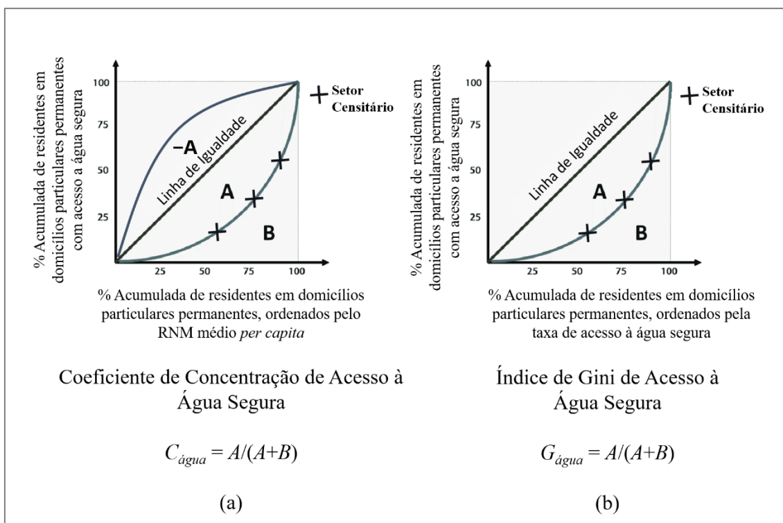
Figura 3.4. Curvas de Lorenz adaptadas para obtenção do Coeficiente de Concentração de Acesso à Água Segura (a) e do Índice de Gini de Acesso à Água Segura (b).
