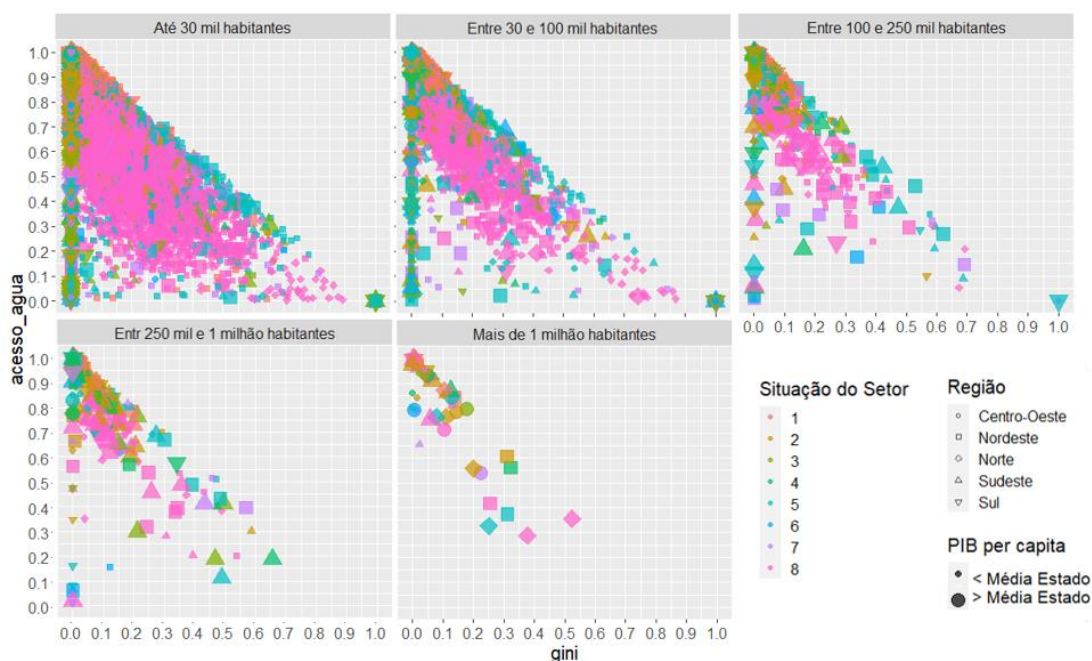
Figura 4.40 – Relações gráficas entre os resultados de G_{\text{água}} e IAAS dos municípios com os setores censitários discriminados em função da situação desses conforme Tabela 4.3.
