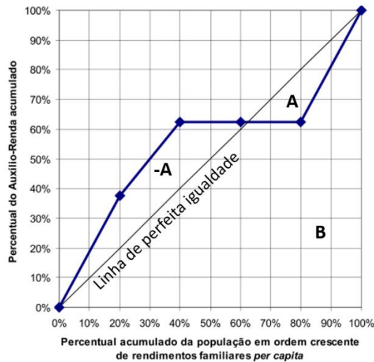
Figura 2.7 – Curva de Concentração segundo rendimentos da população.
