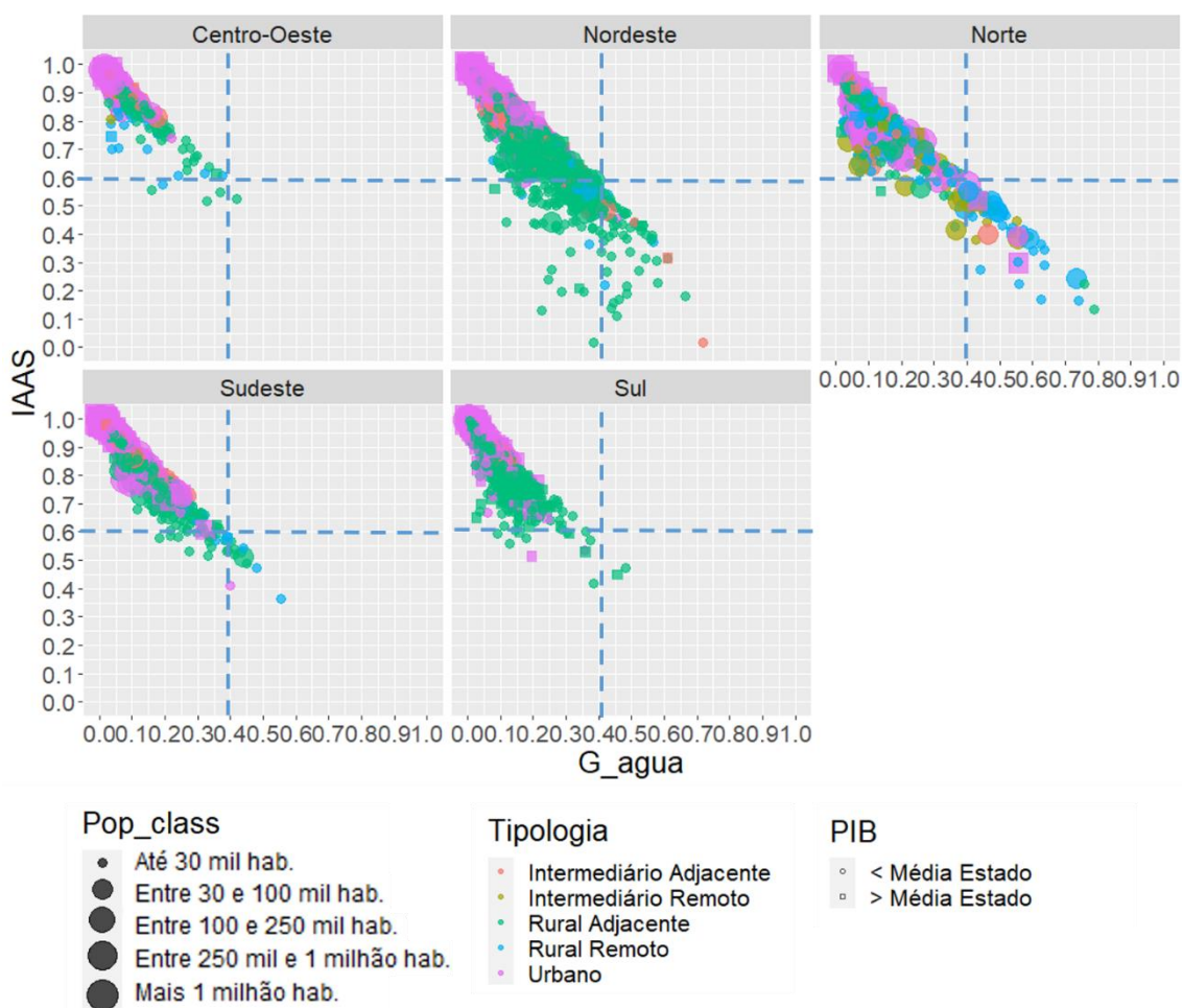
Figura 4.20 – Relações gráficas entre os resultados de G_{\text{água}} e IAAS dos municípios por Região do Brasil, considerando população, tipologia e PIB per capita .
