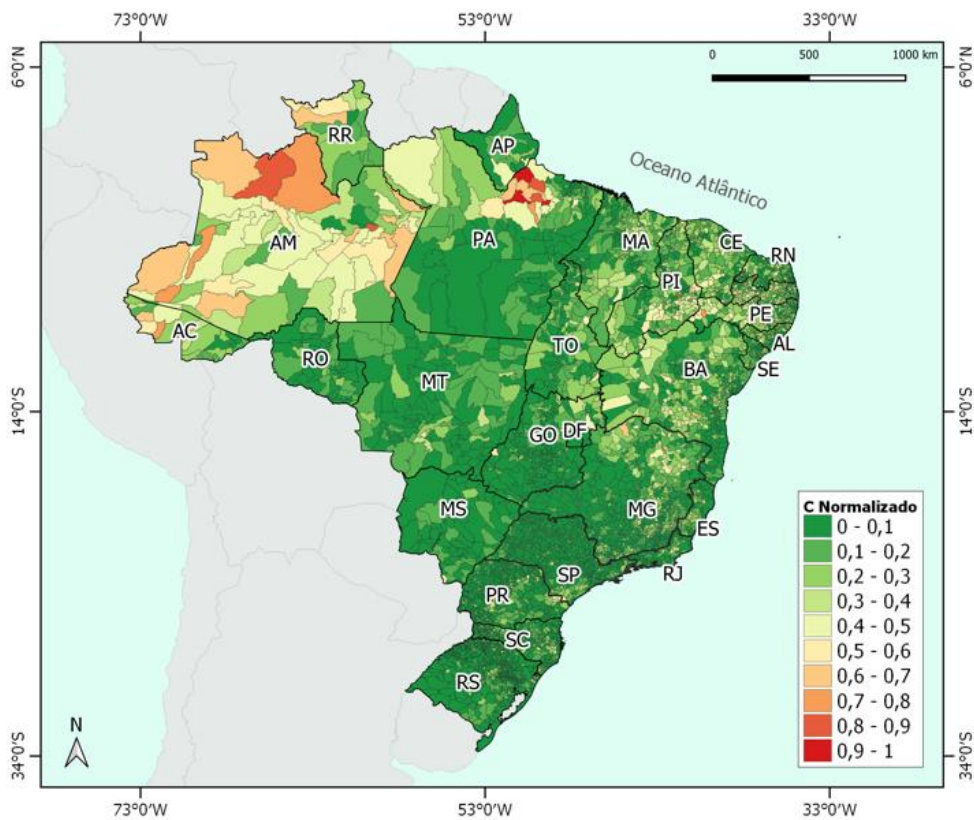
Figura 4.35 - Resultados de C_{\text{água}} normalizados.
