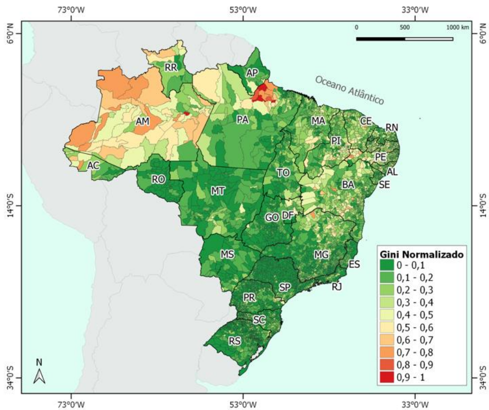
Figura 4.34 - Resultados de G_{\text{água}} normalizados.
