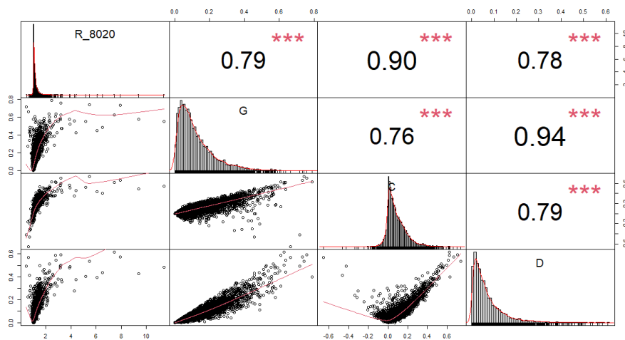
Figura 4.38 - Correlograma dos resultados dos índices de desigualdades adaptados para acesso à água segura.
