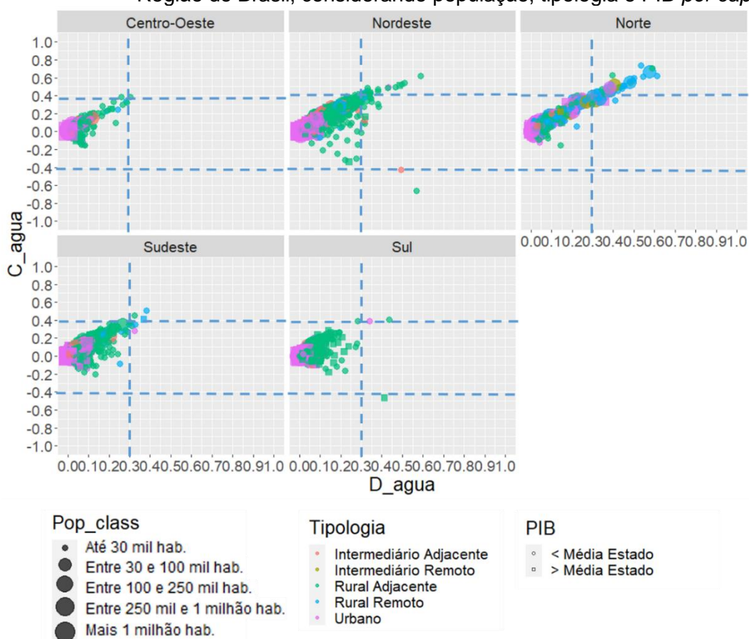
Figura 4.31 – Relações gráficas entre os resultados de C_{\text{água}} e D_{\text{água}} dos municípios por Região do Brasil, considerando população, tipologia e PIB per capita .
