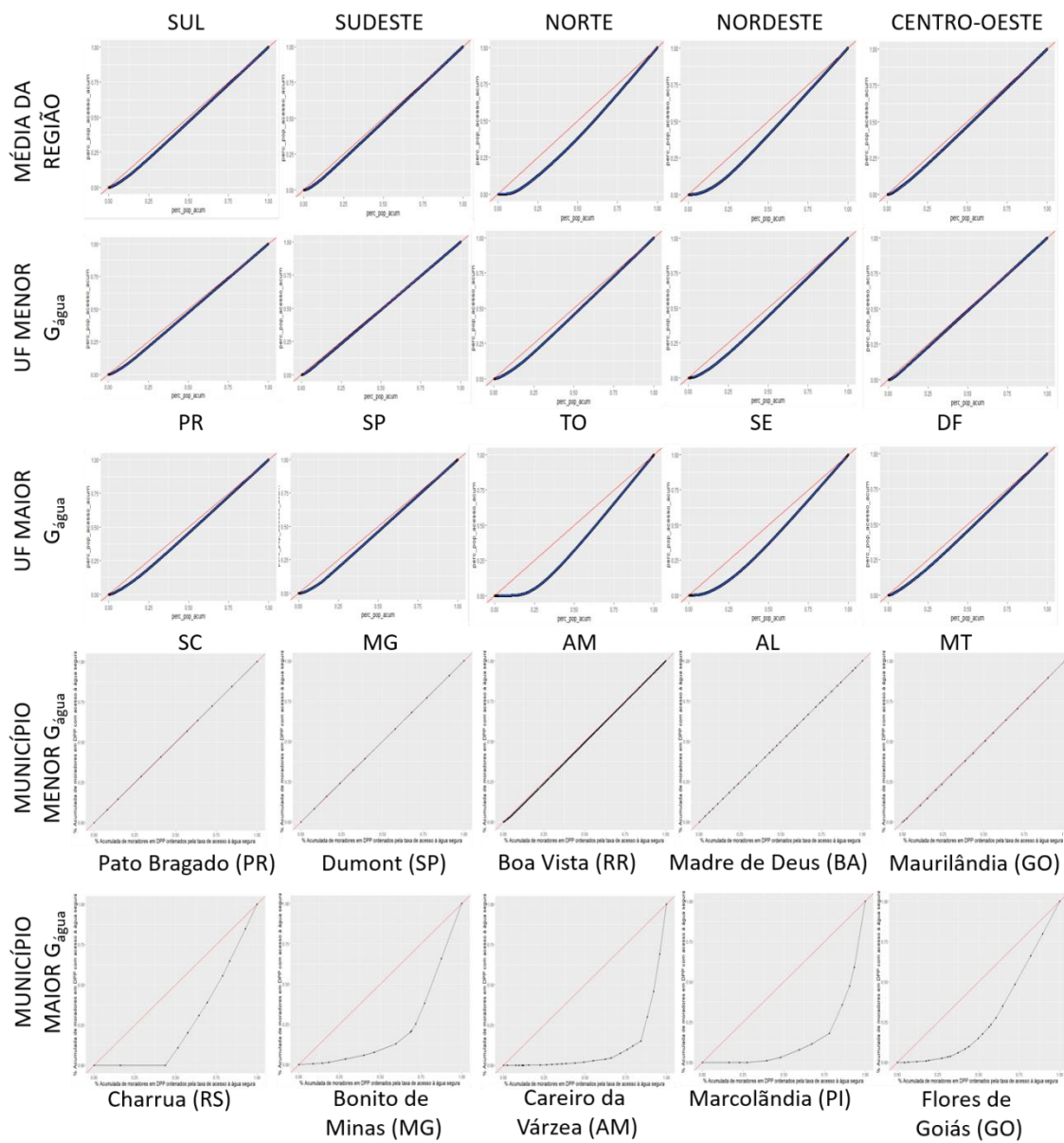
Figura 4.23 – Curvas de Lorenz para as Regiões do Brasil, e respectivos estados e municípios menores e maiores resultados de G_{\text{água}} .
