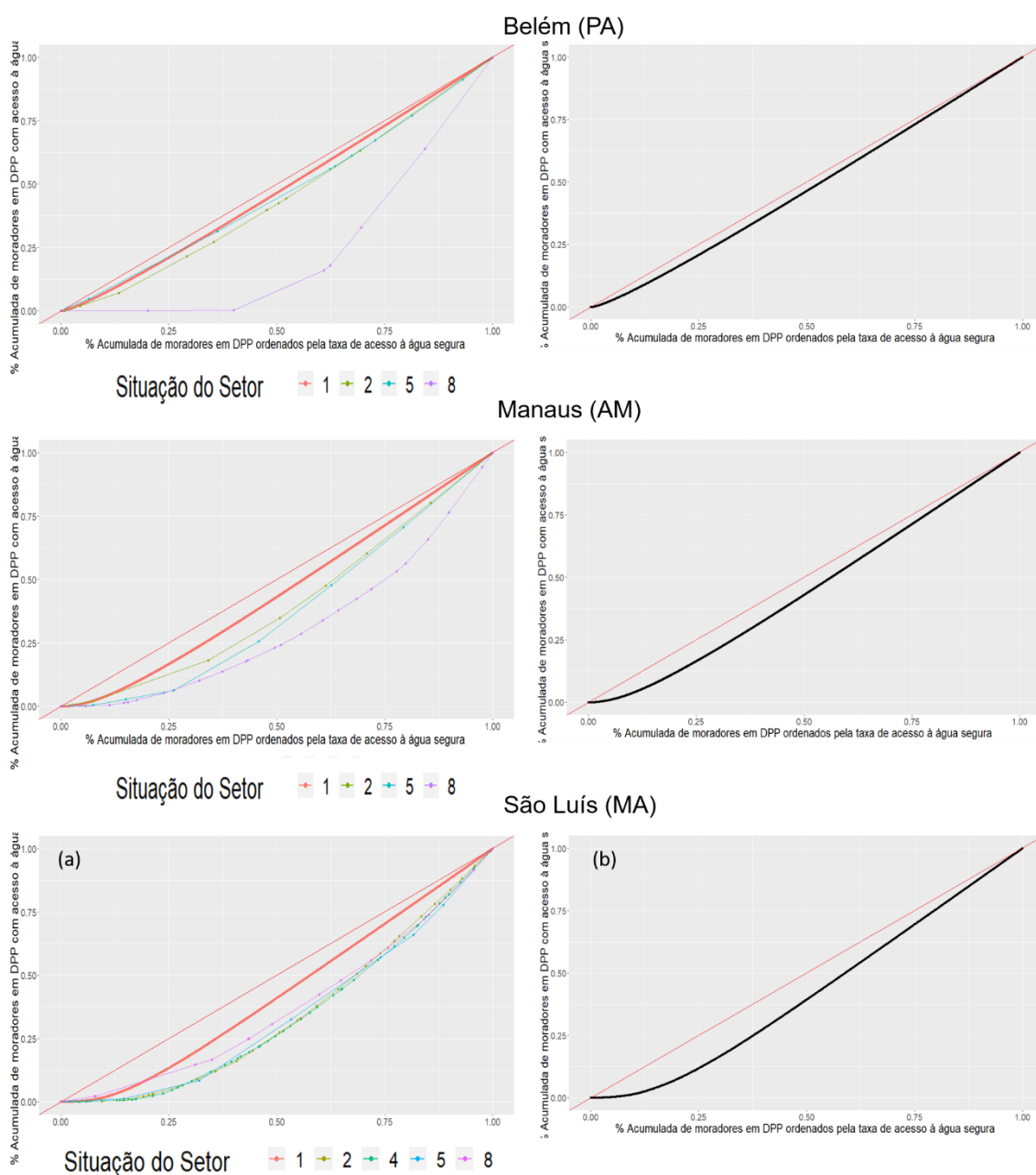
Figura 4.41 – Curvas de Lorenz para alguns municípios com mais de 1 milhão de moradores em DPP discriminadas em função da situação dos setores censitários (a) e para todo o município (b).
