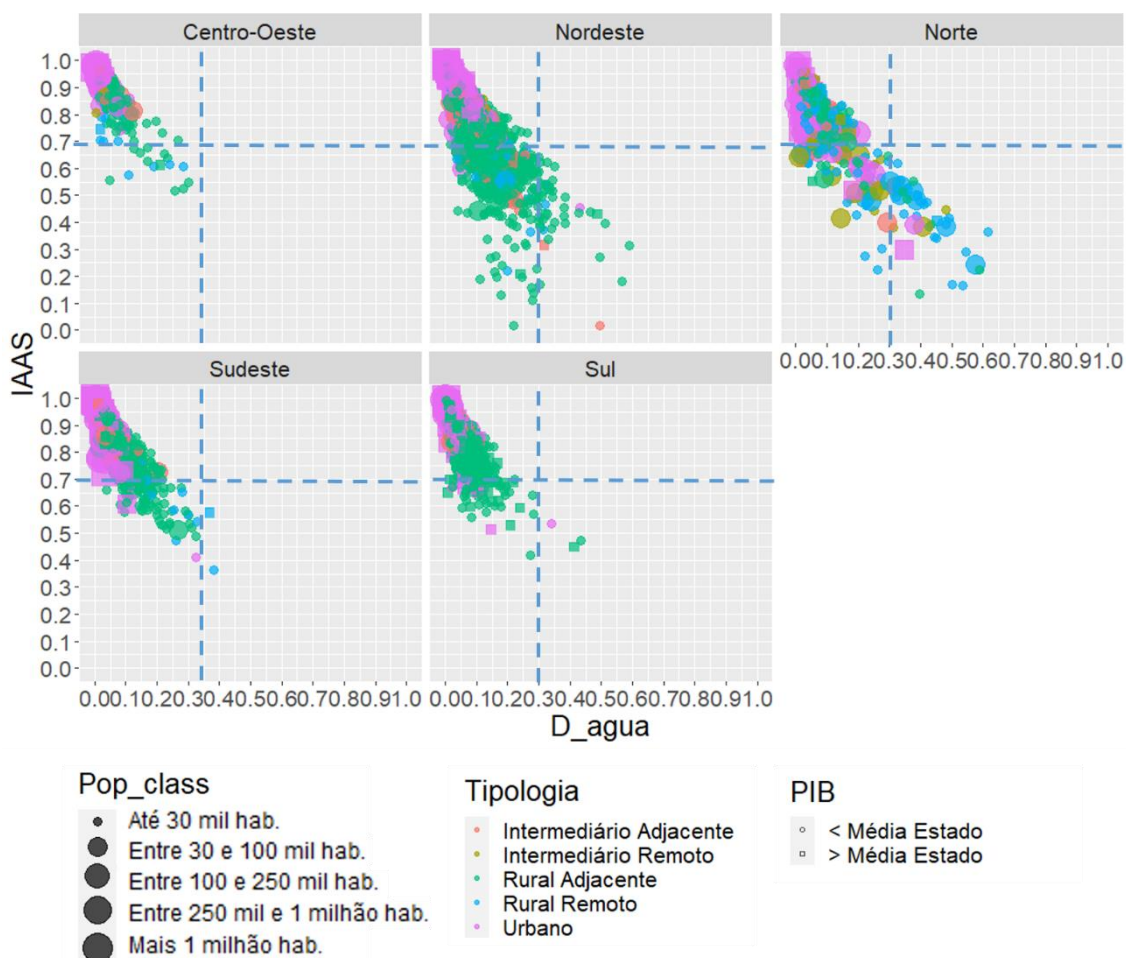
Figura 4.26 – Relações gráficas entre os resultados de D_{água} e IAAS dos municípios por Região do Brasil, considerando população, tipologia e PIB per capita .
