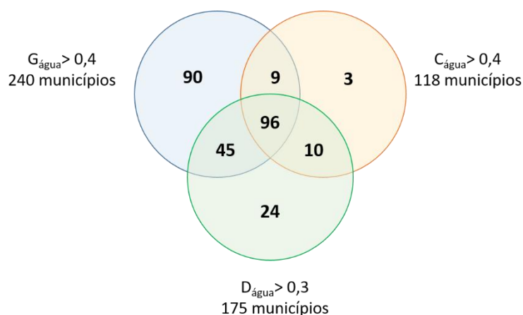
Figura 4.27 – Diagrama de Venn com sobreposição dos conjuntos de dados dos resultados de G_{água} , C_{água} e D_{água} considerados elevados conforme Tabelas 3.4 e 3.5.
