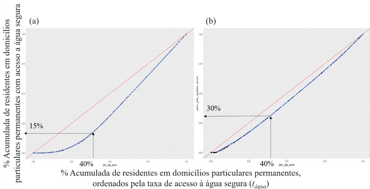
Figura 5.1 - Curvas de Lorenz de dois municípios com população de 102.033 e 99.075 habitantes, respectivamente, e com valores de IAAS de 72,8%.
