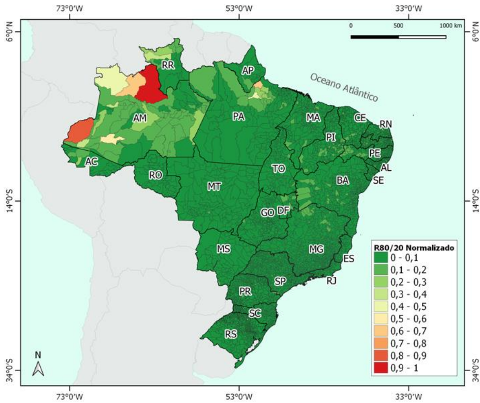
Figura 4.37 - Resultados de R_{80/20} normalizados.
