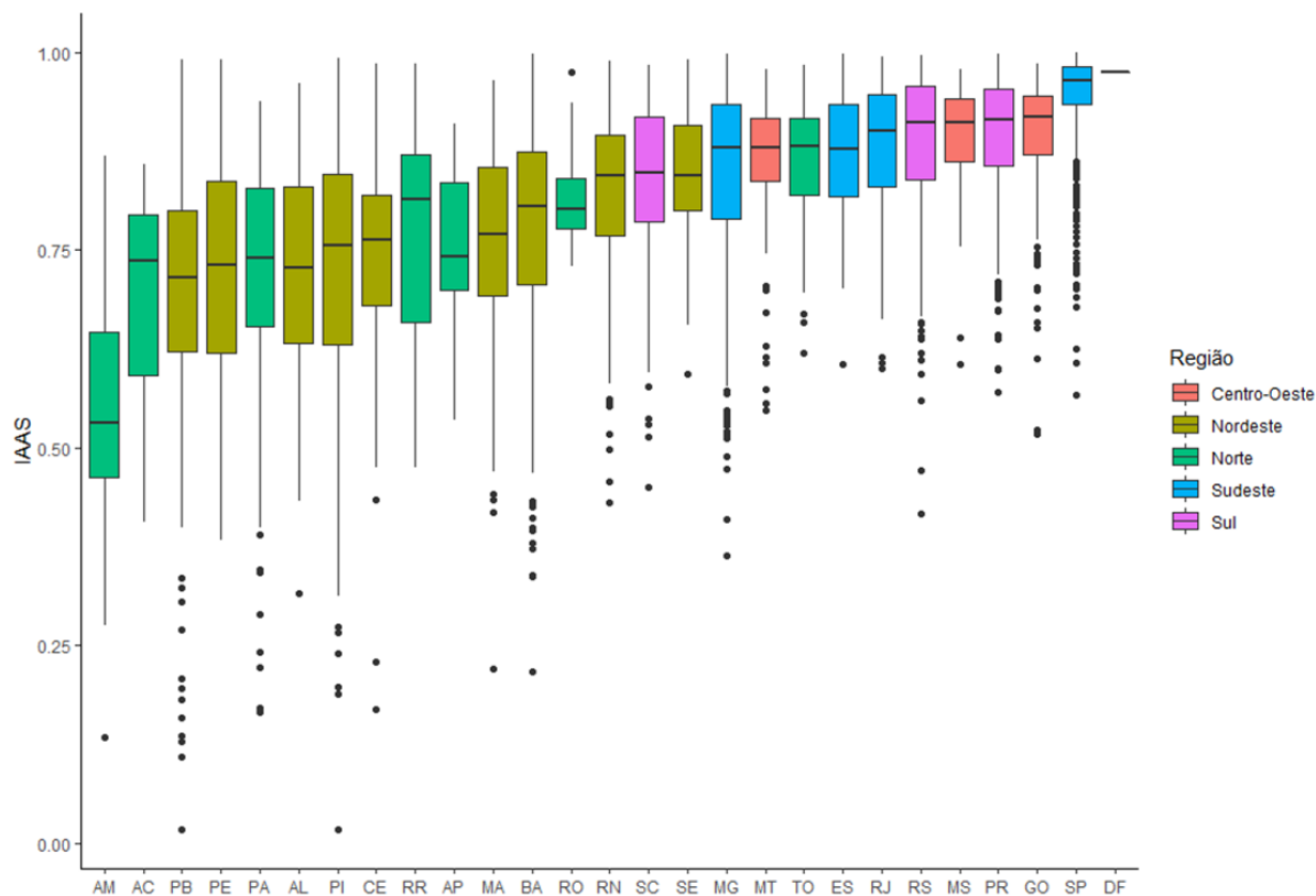
Figura 4.6 – Tabela com boxplots dos resultados de IAAS para os municípios discriminados por estados e Regiões.
