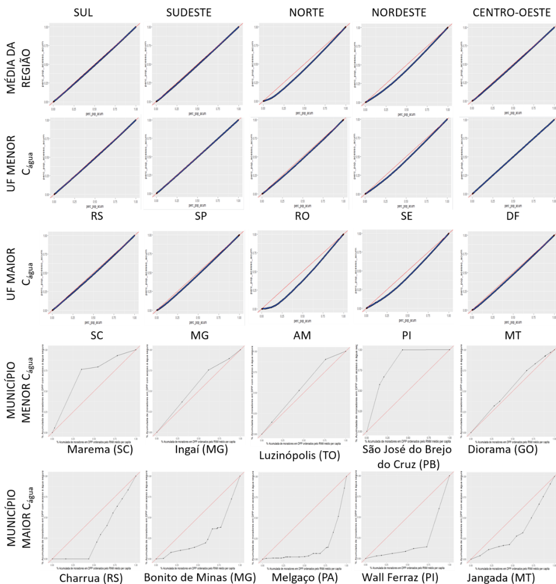
Figura 4.24 – Curvas de Concentração para as Regiões do Brasil, e respectivos estados e municípios do Brasil com menores e maiores resultados de C_{\text{água}} .
