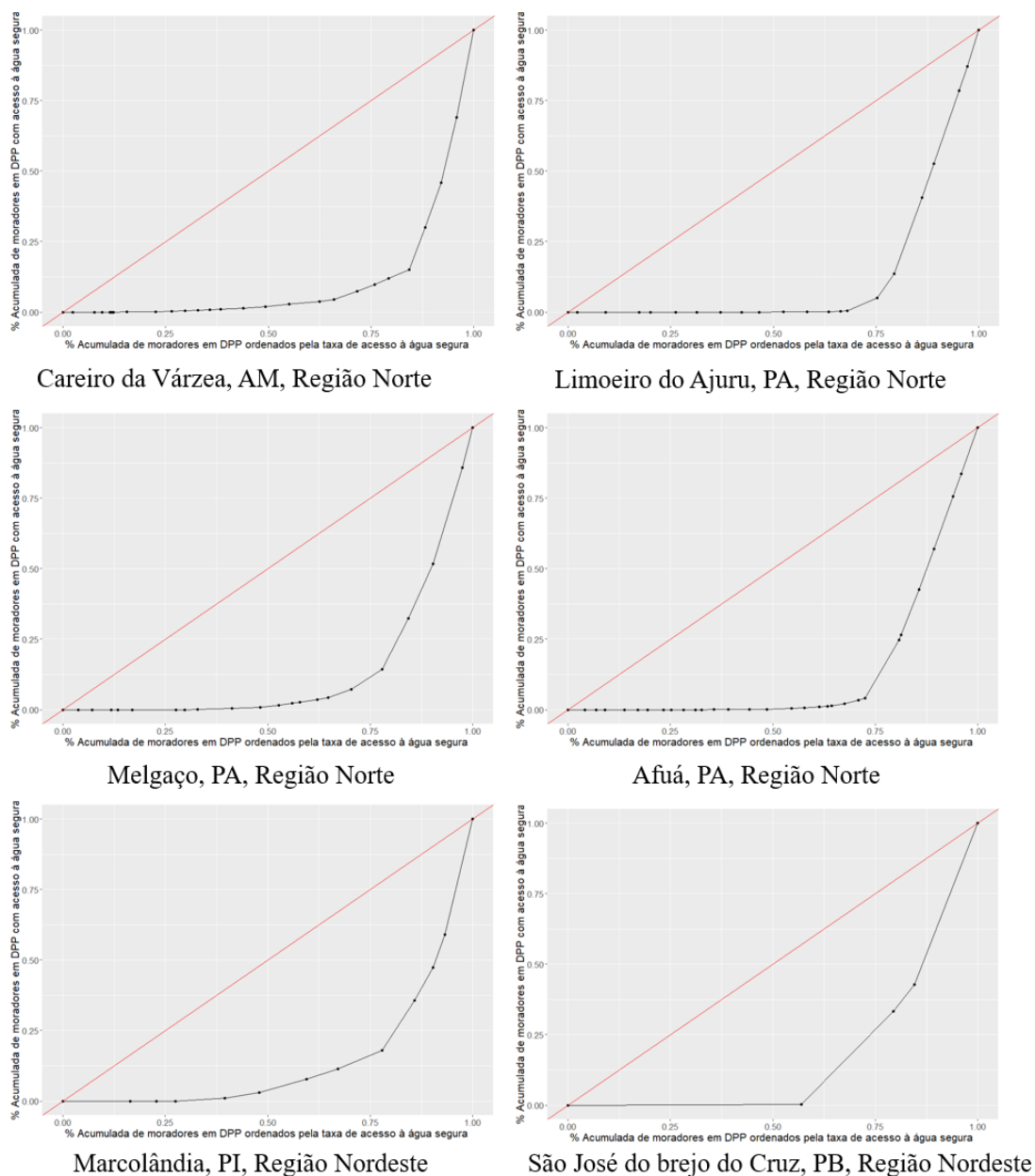
Figura 4.18 – Curvas de Lorenz dos municípios com maiores valores de G_{\text{água}} .
