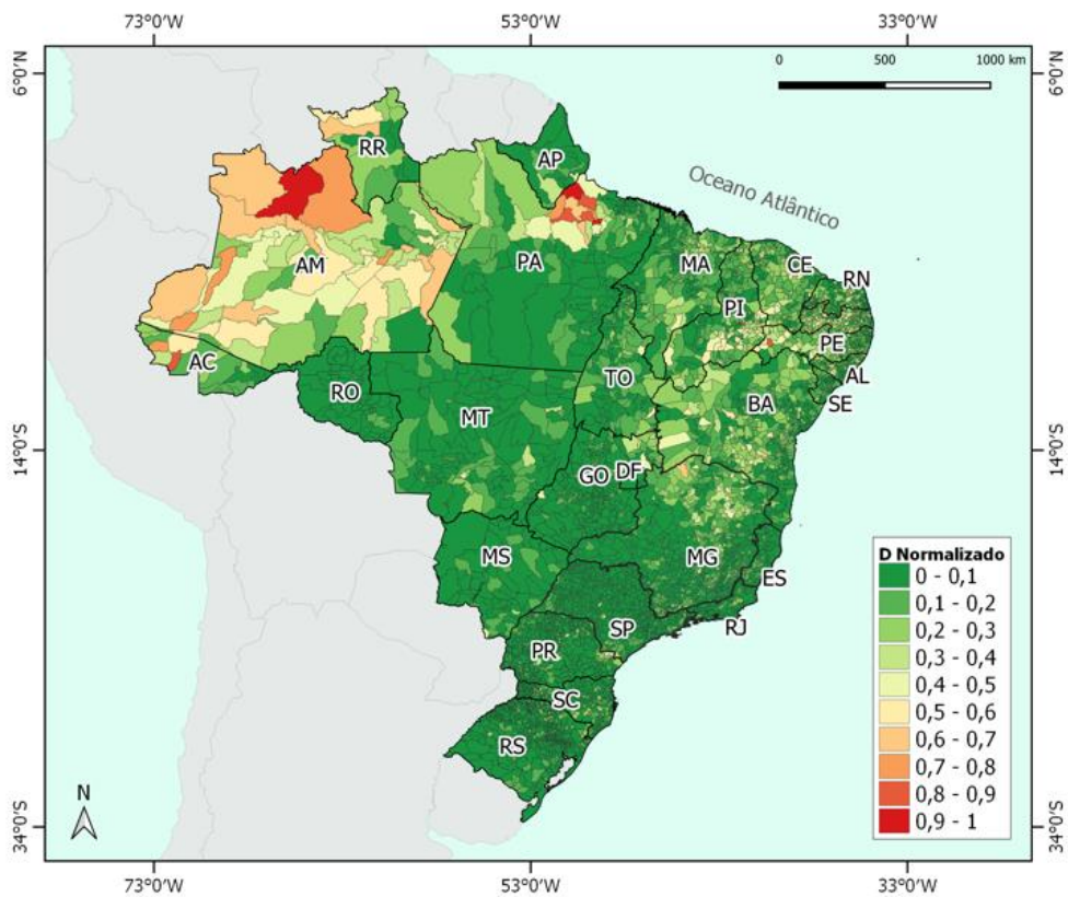
Figura 4.36 - Resultados de D_{\text{água}} normalizados.
