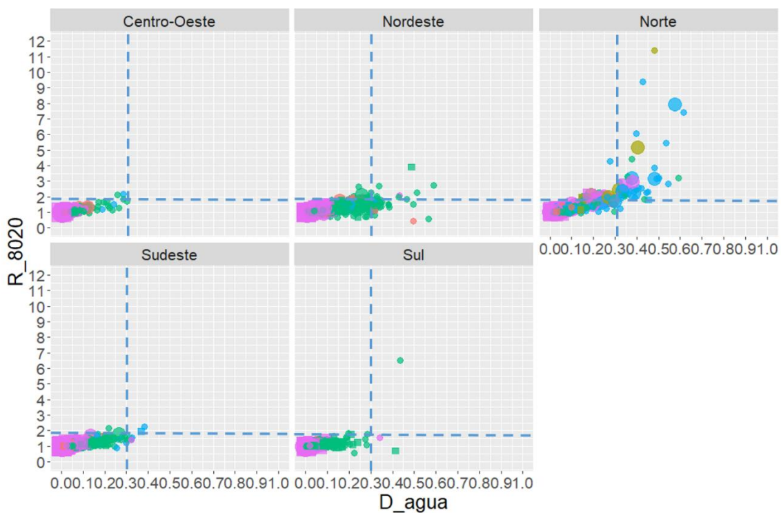
Figura 4.33 – Relações gráficas entre os resultados de D_{\text{água}} e R_{80/20} dos municípios por Região do Brasil, considerando população, tipologia e PIB per capita .
