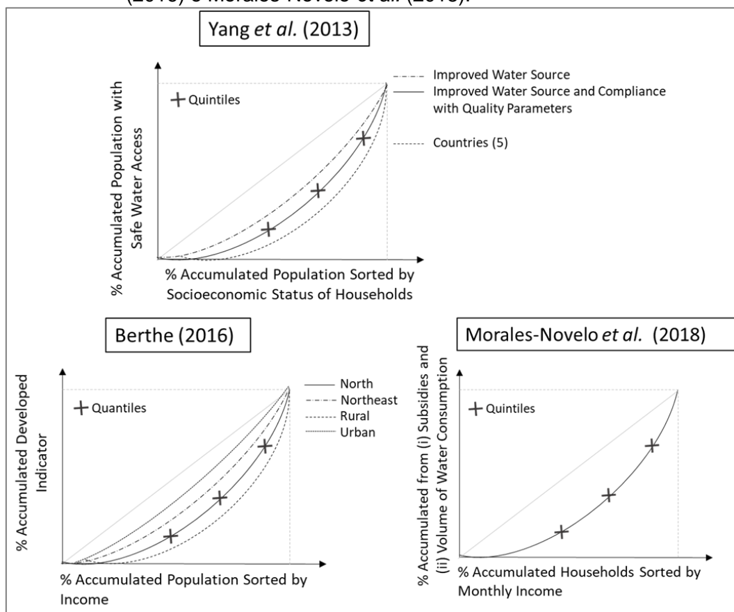
Figura 2.11 – Curvas de Concentração adaptadas por Yang et al. (2013), Berthe (2016) e Morales-Novelo et al. (2018).
