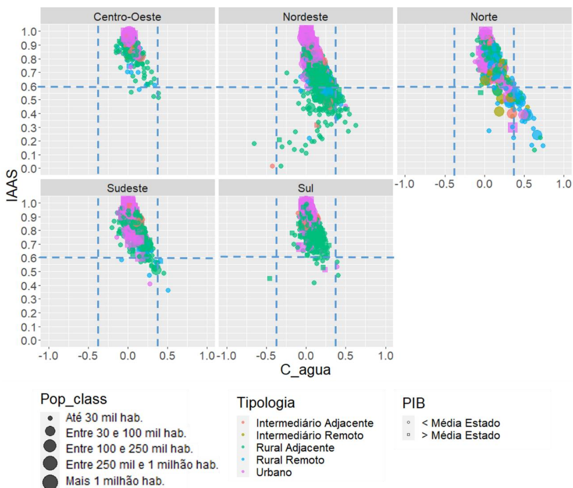
Figura 4.22 – Relações gráficas entre os resultados de C_{\text{água}} e IAAS dos municípios por Região do Brasil, considerando população, tipologia e PIB per capita .
