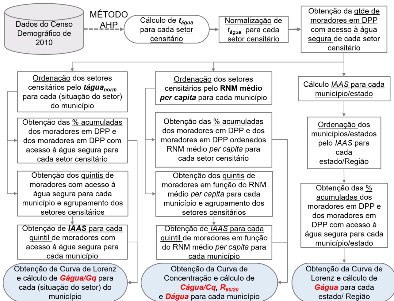
Figura 3.1 – Esquema com as etapas da pesquisa e os respectivos índices de desigualdades adaptados para acesso à água segura resultantes.
