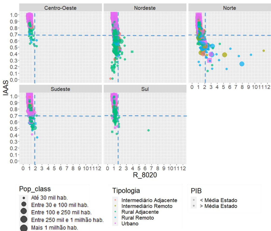
Figura 4.25 – Relações gráficas entre os resultados de R_{80/20} e IAAS dos municípios por Região do Brasil, considerando população, tipologia e PIB per capita .
