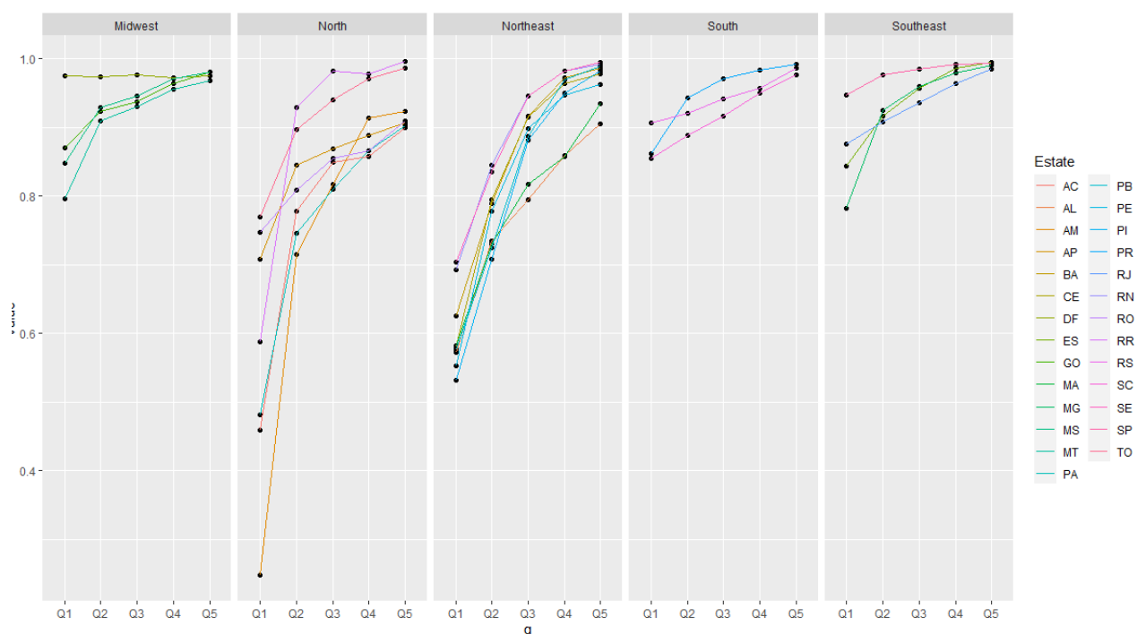
Figura 4.9 - Relação entre os valores de IAAS em função do quintil de RNM médio per capita para as Regiões do país.
