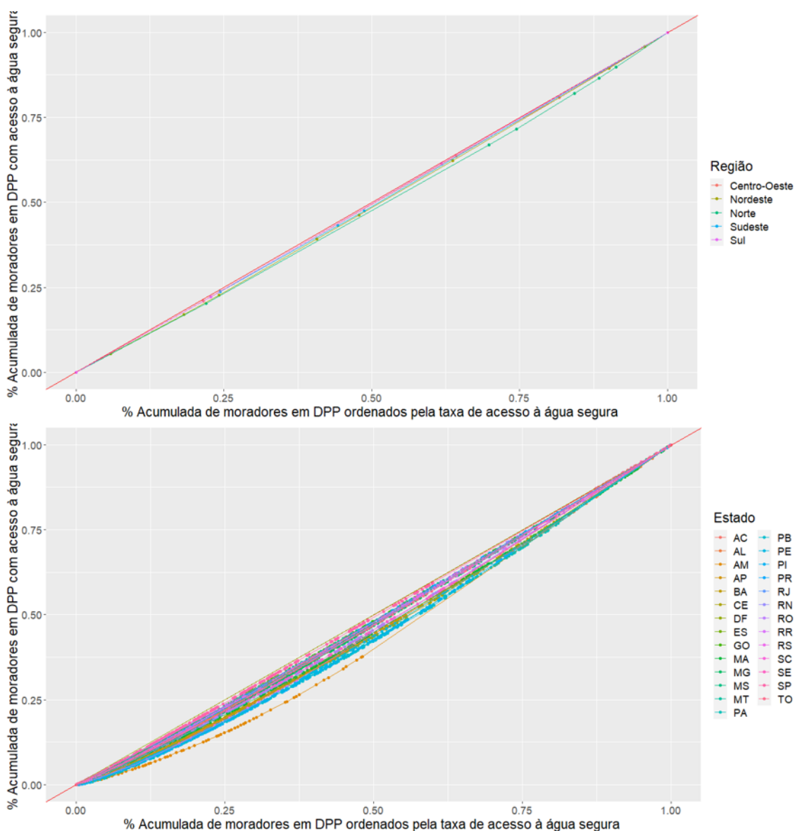
Figura 4.19 - Curvas de Lorenz para os estados e Regiões do país.
