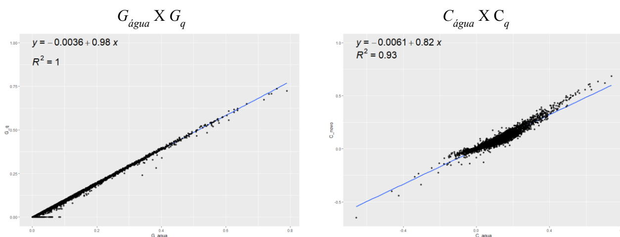
Figura 4.17 – Correlação entre G_{\text{água}} e G_q , e C_{\text{água}} e C_q , com linha de tendência linear, respectiva equação e R^2 .
