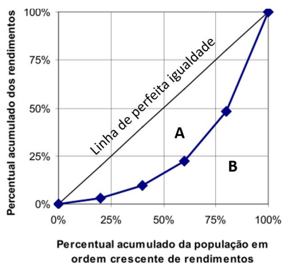
Figura 2.6 – Curva de Lorenz segundo rendimentos da população.
