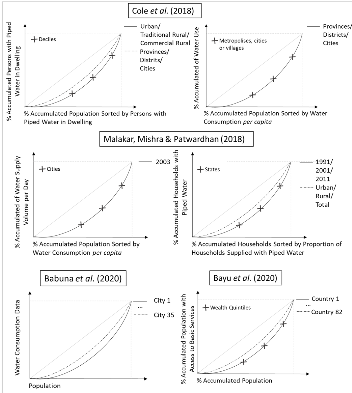
Figura 2.9 – Curvas de Lorenz adaptadas por Cole et al. (2018), Malakar, Mishra e Patwardhan (2018), Babuna et al. (2020) e Bayu et al. (2020).
