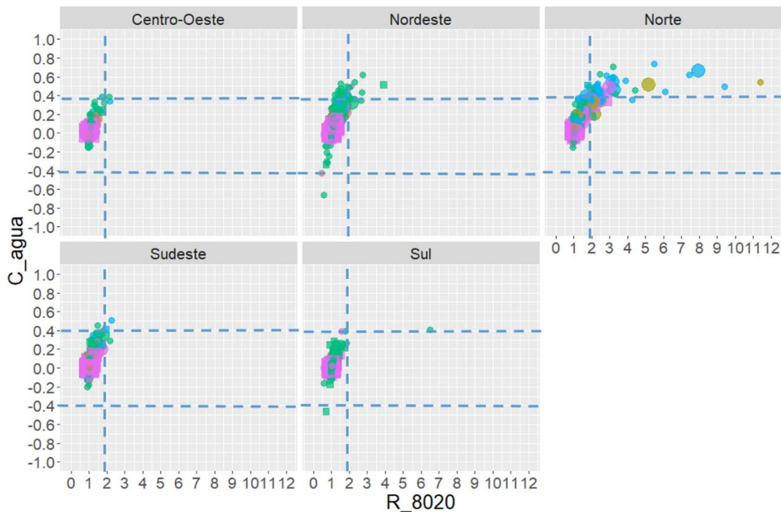
Figura 4.32 – Relações gráficas entre os resultados de C_{\text{água}} e R_{80/20} dos municípios por Região do Brasil, considerando população, tipologia e PIB per capita .
