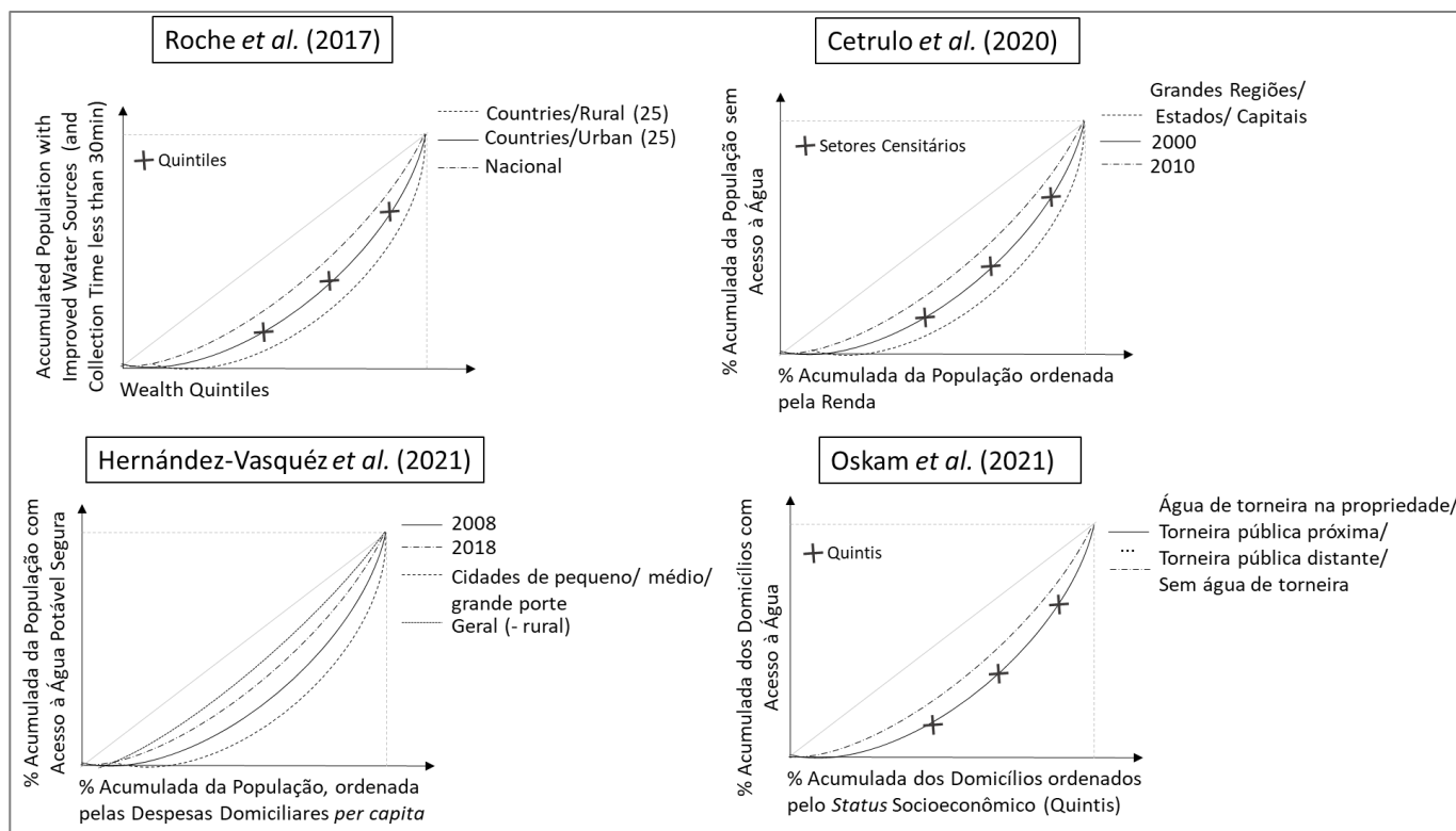
Figura 2.12 – Curvas de Concentração adaptadas por Roche et al. (2017), Cetrulo et al. (2020), Hernández-Vasqu ez et al. (2021) e Oskam et al. (2021).
