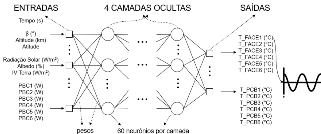
Figura 3.11 – Arquitetura da RNA.
