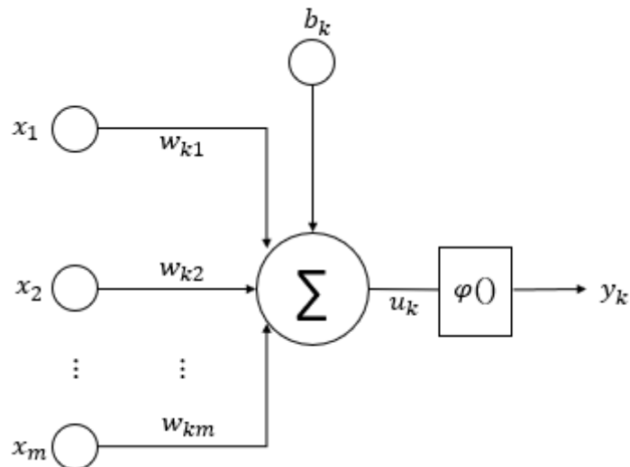
Figura 2.7. – Modelo não-linear de um neurônio.
