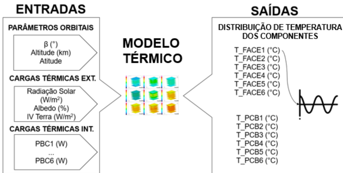
Figura 3.2 - Entradas e saídas do modelo térmico.
