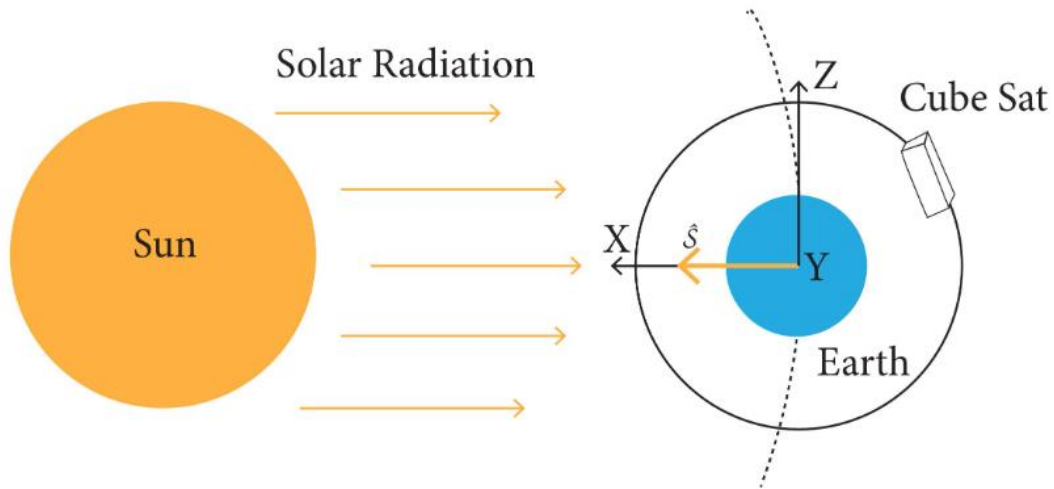
Figura 3.5 – Incidência da radiação solar sobre o CubeSat.
