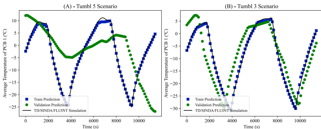
Figura 4.2 - Comparação entre as previsões de treinamento e validação da PCB 1 usando (A) cenário Tumbl 05 e (B) cenário Tumbl 03 para validação.
