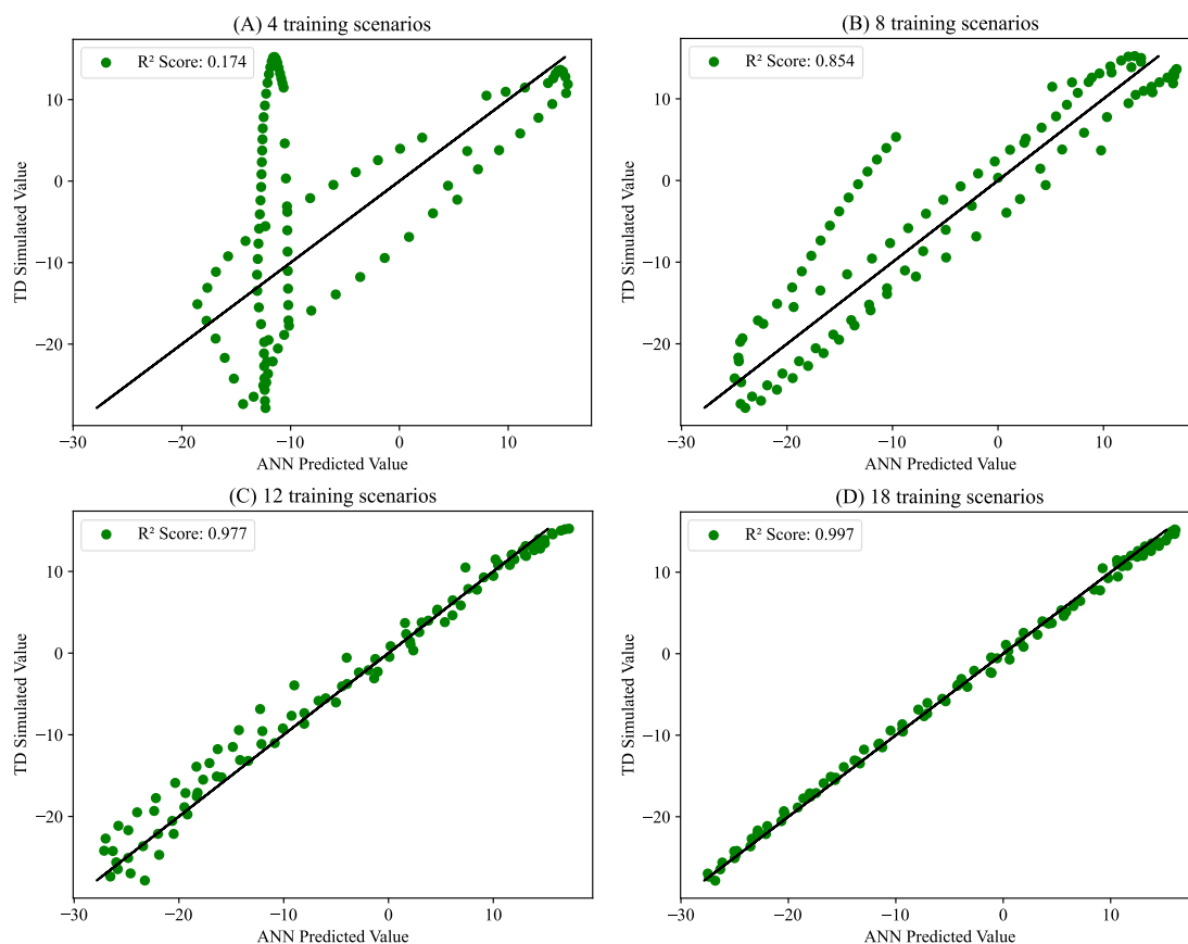
(A) 4 cenários utilizados para treinamento, (B) 8 cenários utilizados para treinamento, (C) 12 cenários utilizados para treinamento e (D) 18 cenários utilizados para treinamento.
