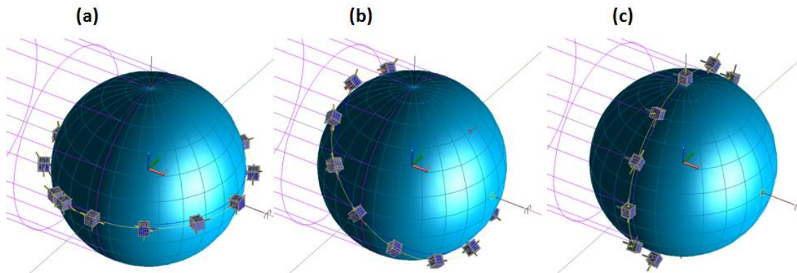
Figura 3.9 - Ilustração das órbitas com (a) \beta = 0^\circ , (b) \beta = 45^\circ , e (c) \beta = 90^\circ .
