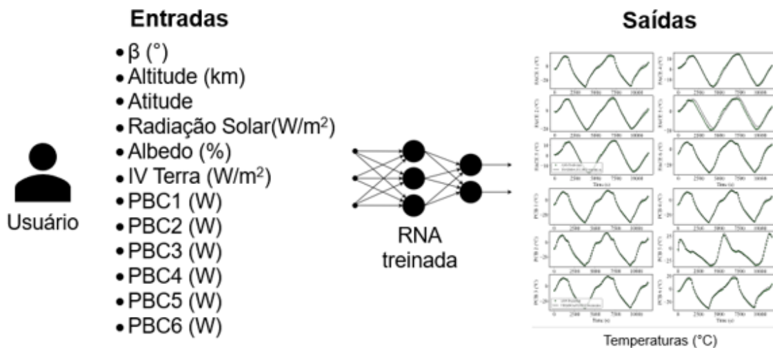
Figura 4.7 – Utilização da RNA treinada por um usuário para obtenção da distribuição de temperaturas do CubeSat.
