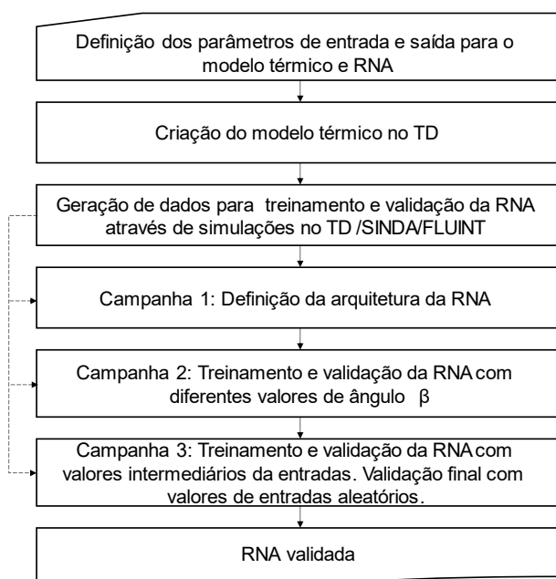
Figura 3.1 - Principais etapas do desenvolvimento da RNA.
