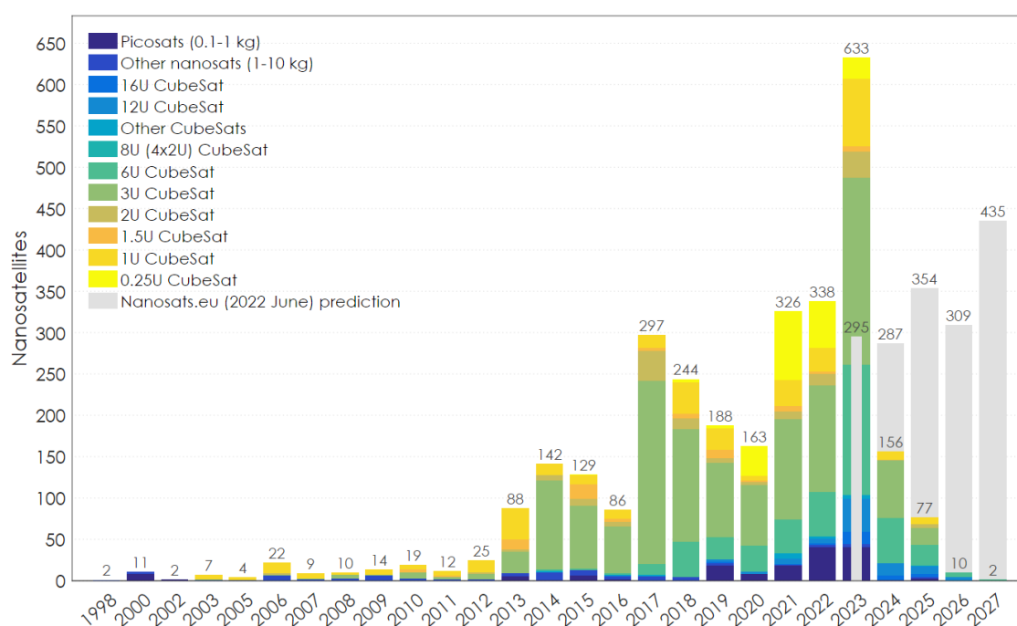
Figura 1.2. – Quantidade de nanosatélites lançados por tipo ao longo do tempo.
