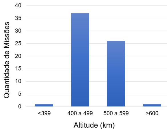
Figura 3.3 – Quantidade de missões de CubeSats 1U por faixa de altitude da órbita.
