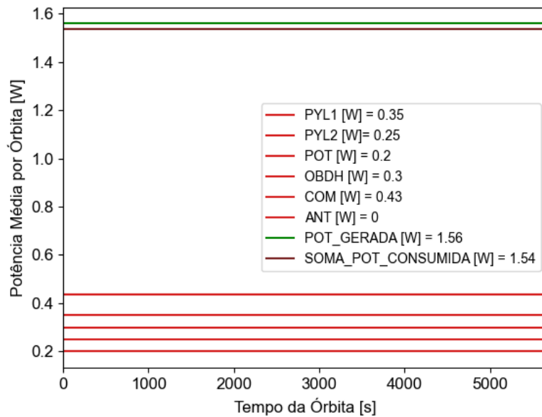
Figura 3.6 – Exemplo de consumo e geração de potência de um CubeSat 1U composto por 6 PCBs.
