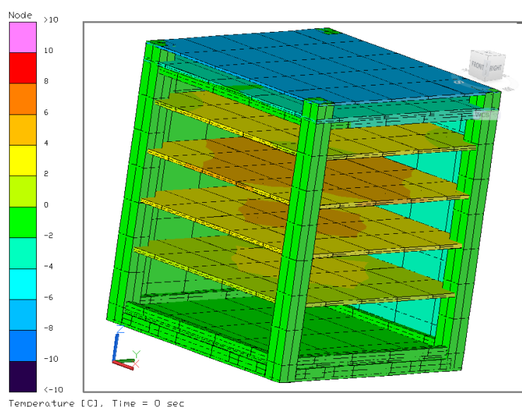
Figura 3.10 - Distribuição de temperatura no início da simulação transiente para o caso de estudo PassCon24 (ver Apêndice A para a descrição do caso). Faces Y- e X+ removidas para visualização das PCBs.
