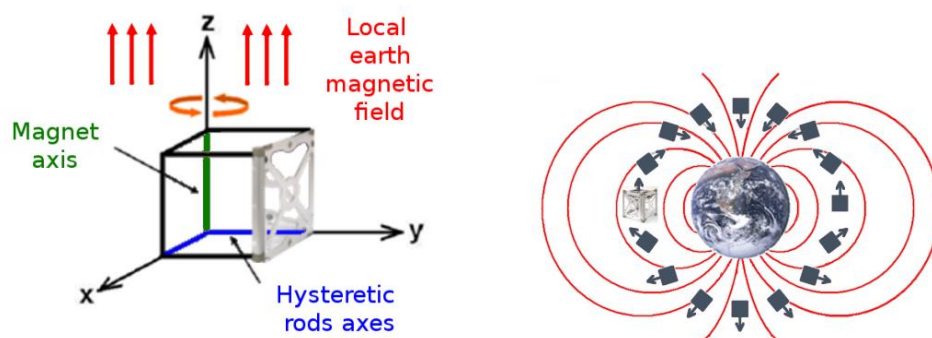
Figura 3.4 – Controle passivo de atitude em CubeSats. A orientação do satélite acompanha o campo magnético da Terra.
