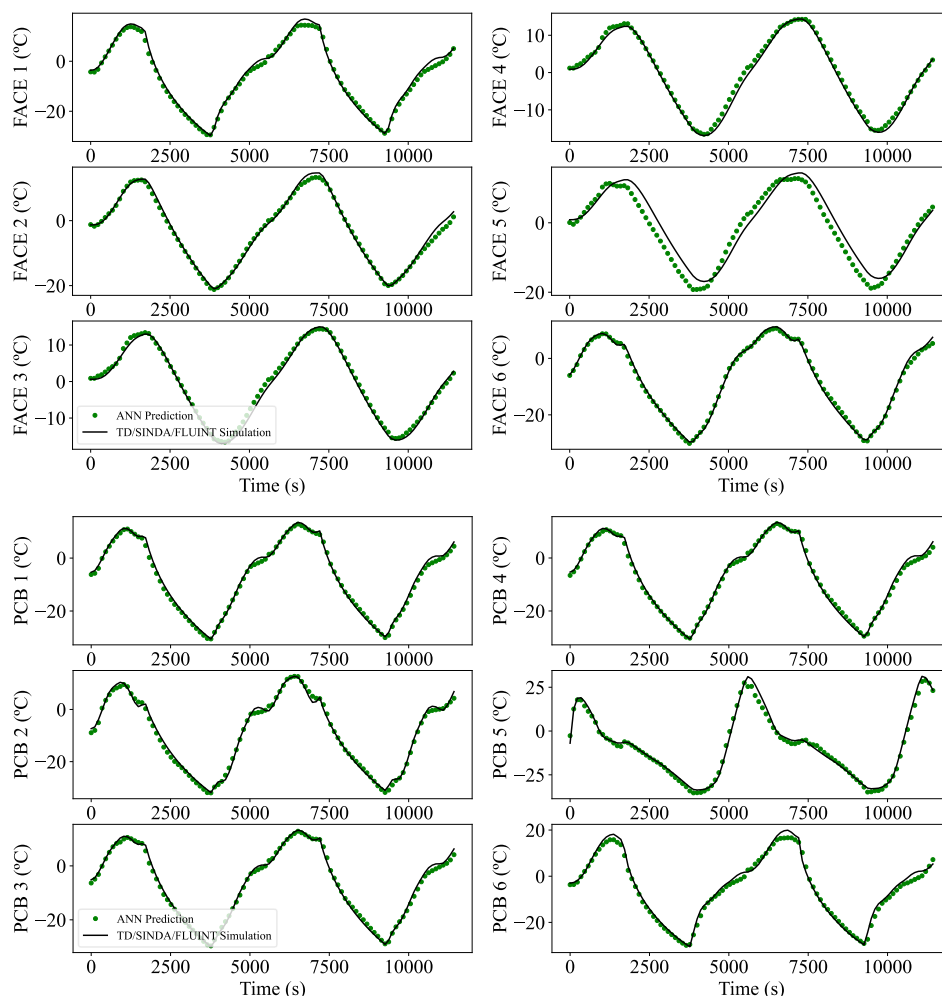
Figura 4.6 - Comparação entre o valor simulado e predito em um cenário de validação (PassCon39) com a RNA treinada.
