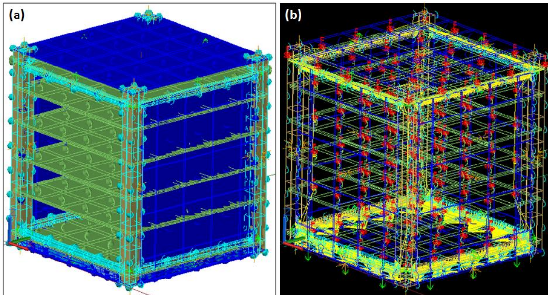
Figura 3.8 – Modelo térmico do CubeSat.
