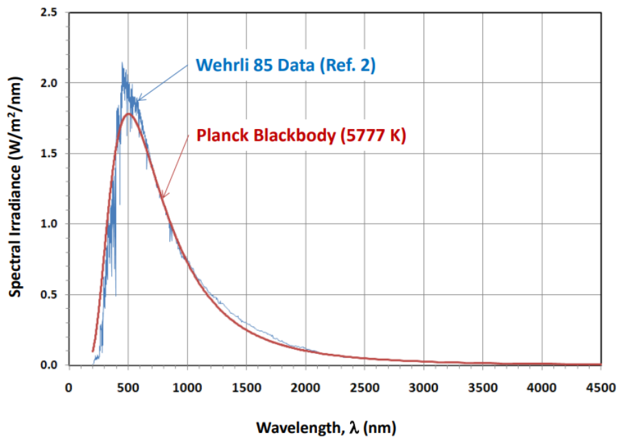
Figura 2.2. - Espectro da radiação solar.
