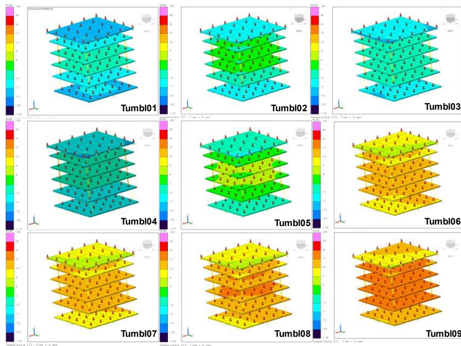
Figura 4.1 – Temperaturas dos nós do submodelo PCB após atingir regime permanente nos cenários da campanha 1.
