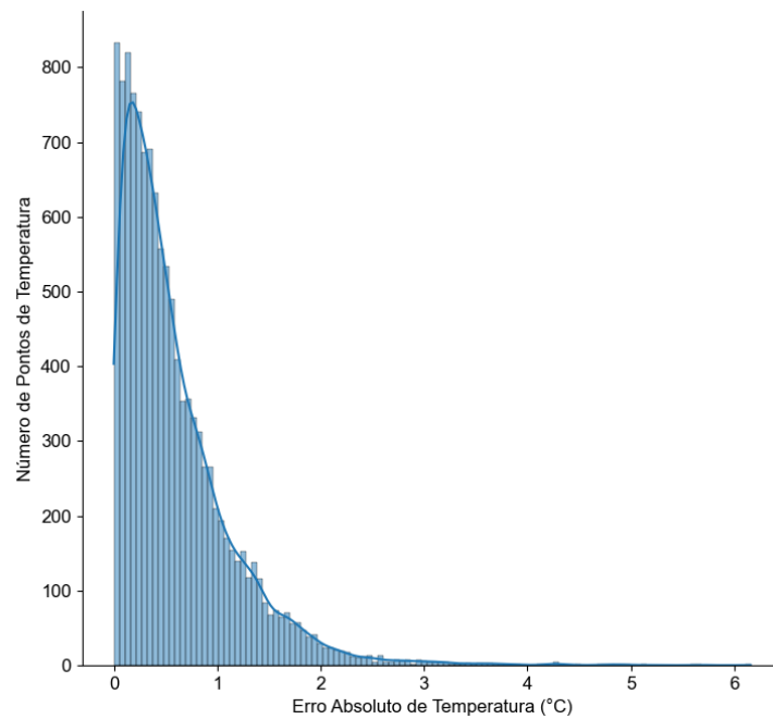
Figura 4.5 - Distribuição do erro absoluto para os dados de validação (12120 amostras).
