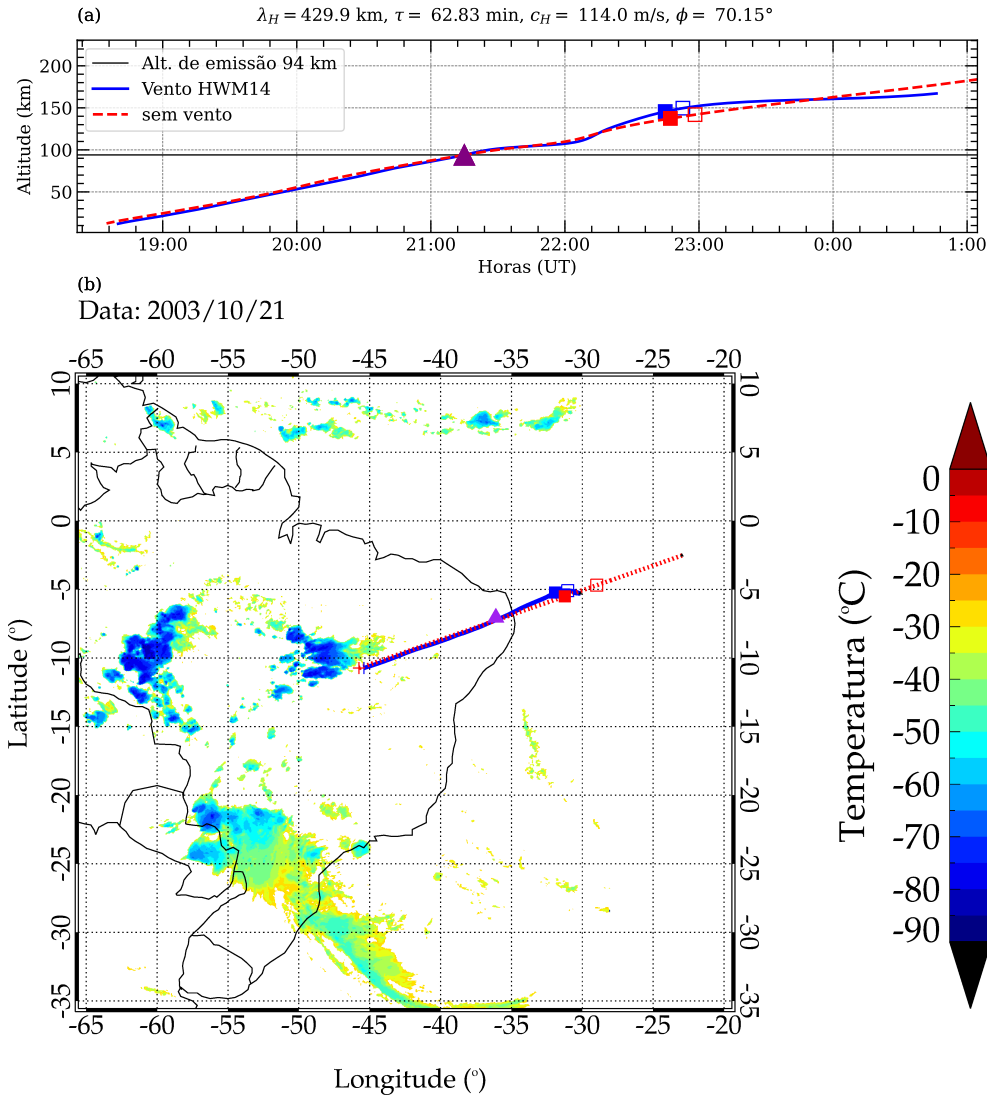
(a) Retrotrajetória da onda de gravidade de média escala em função do tempo. (b) Mapa do Brasil com a retrotrajetória da onda de gravidade e a sobreposição da temperatura de brilho do topo de nuvens, obtidos pelo satélite GOES-12 para o dia 21 de outubro de 2003. Aqui assumiu-se que a onda possui propagação de fase descendente, i.e., com origem na troposfera. Os quadrados preenchidos representam o fluxo de momentum máximo (azul com vento modelado e vermelho sem vento). Os quadrados vazios representam os locais onde o fluxo de momentum é menor do que 10% do fluxo máximo.
