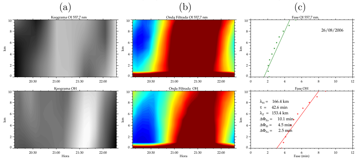
Figura A.23 - Onda de gravidade de média escala observada nas emissões do OI 557,7 nm e OH, na noite de 26/08/2006, em São João do Cariri (PB).
