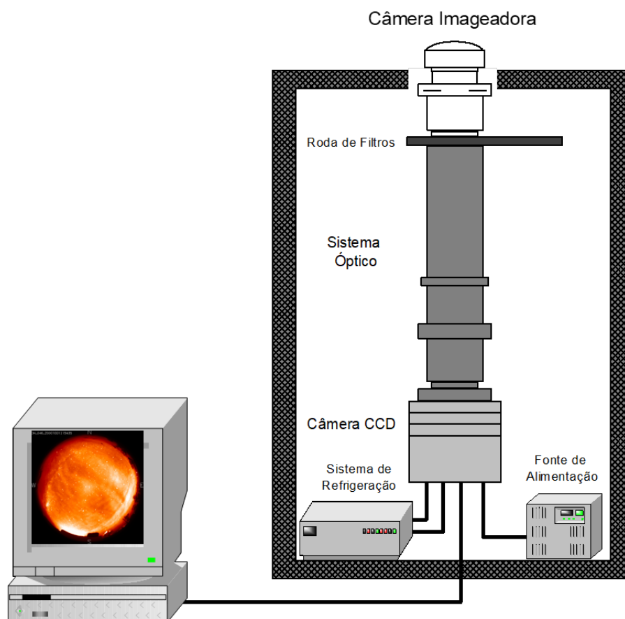
Figura 3.1 - Representação esquemática dos imageadores utilizados no presente trabalho para observar as emissões da aeroluminescência noturna.
