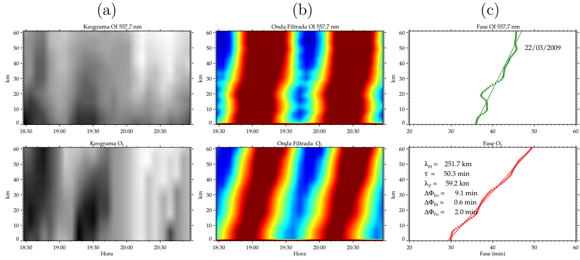
Figura A.32 - Onda de gravidade de média escala observada nas emissões do OI 557,7 nm e O 2 , na noite de 22/03/2009, em São João do Cariri (PB).
