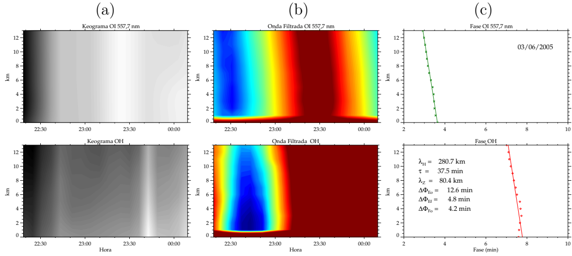
Figura A.20 - Onda de gravidade de média escala observada nas emissões do OI 557,7 nm e OH, na noite de 03/06/2005, em São João do Cariri (PB).
