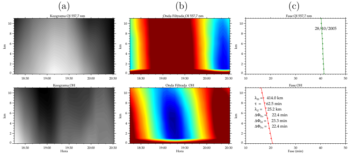
Figura A.21 - Onda de gravidade de média escala observada nas emissões do OI 557,7 nm e OH, na noite de 28/10/2005, em São João do Cariri (PB).
