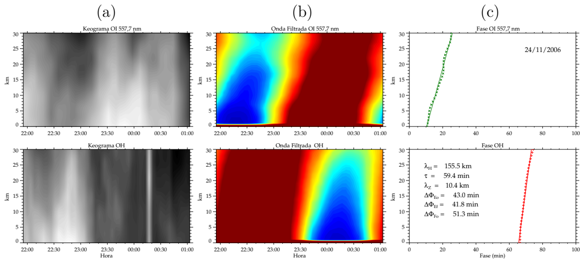
Figura 4.16 - Representação da fase da onda de gravidade de média escala observada na noite de 24 de novembro de 2006.
