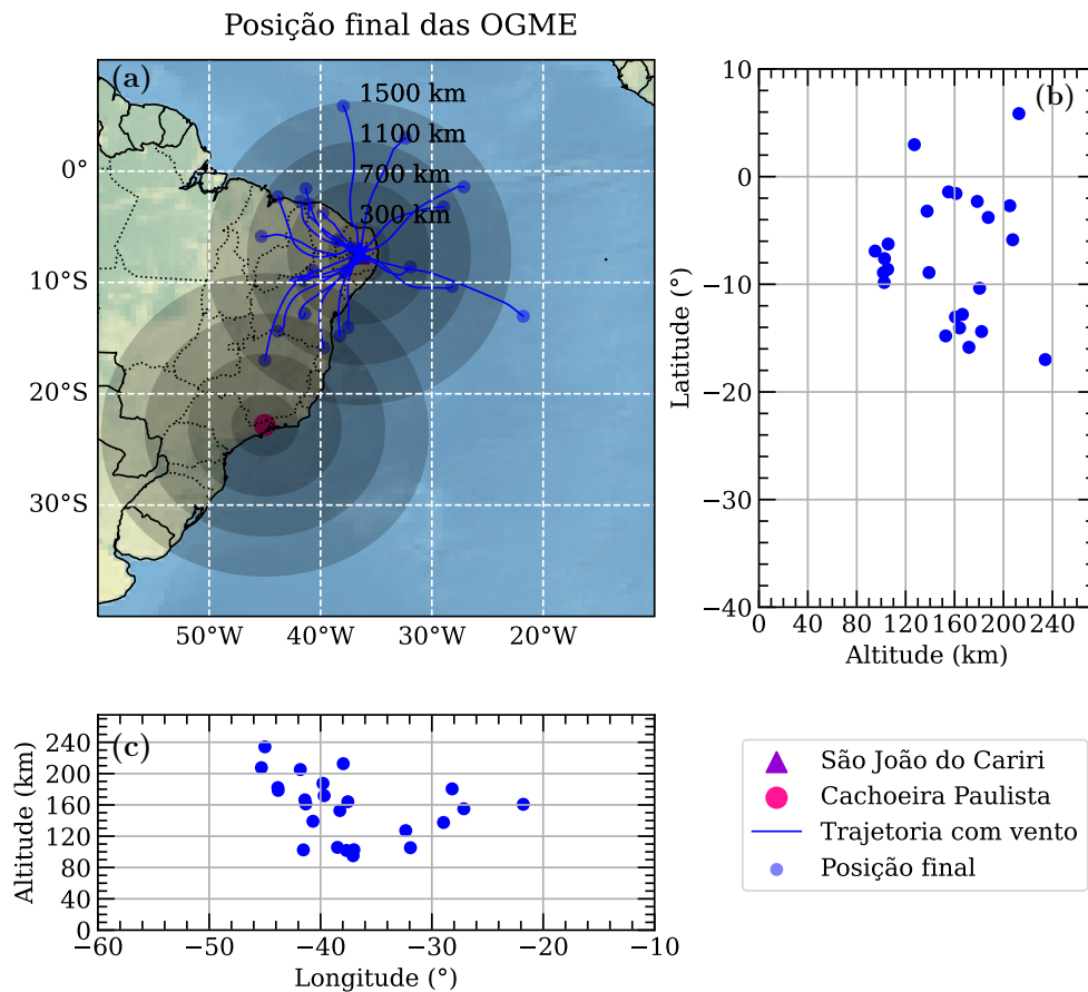
Figura 4.7 - Distribuição das posições finais das ondas de gravidade de média escala com propagação de fase ascendente.
