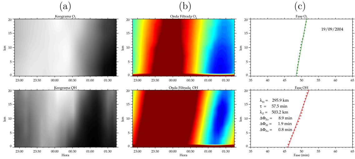
Figura A.18 - Onda de gravidade de média escala observada nas emissões do O 2 e OH, na noite de 19/09/2004, em São João do Cariri (PB).
