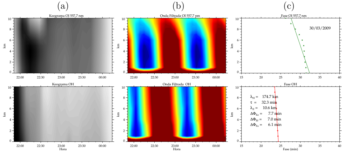
Figura A.33 - Onda de gravidade de média escala observada nas emissões do OI 557,7 nm e OH, na noite de 30/03/2009, em São João do Cariri (PB).
