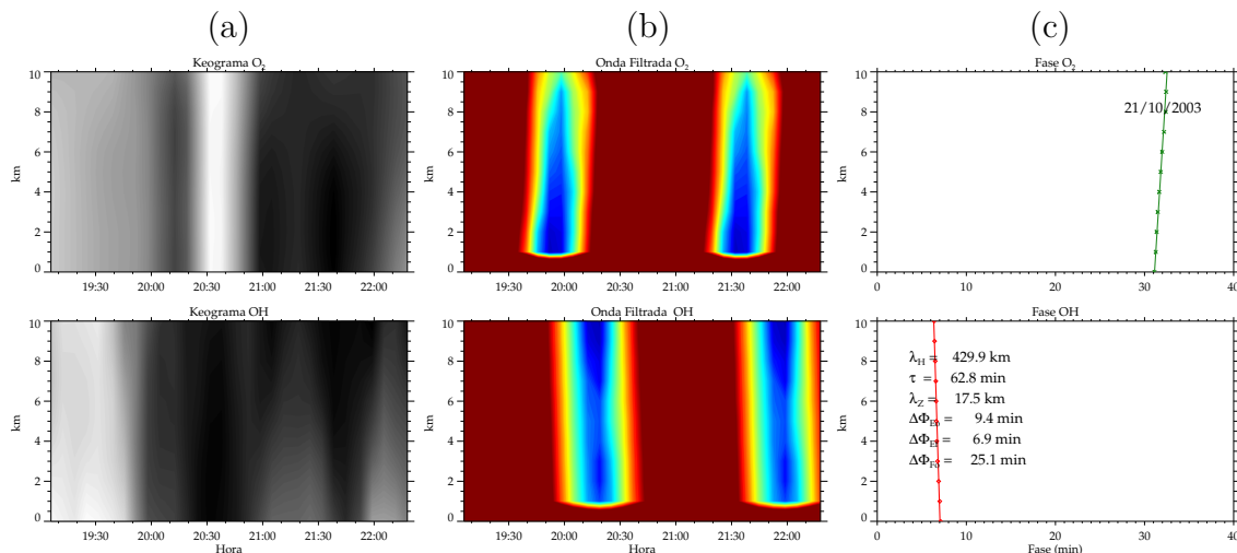
Figura 4.10 - Representação da fase da onda de gravidade de média escala observada na noite de 21 de outubro de 2003.
