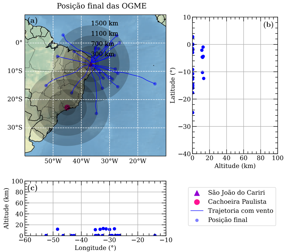
Figura 4.6 - Distribuição das trajetórias das ondas de gravidade de média escala com propagação de fase ascendente.
