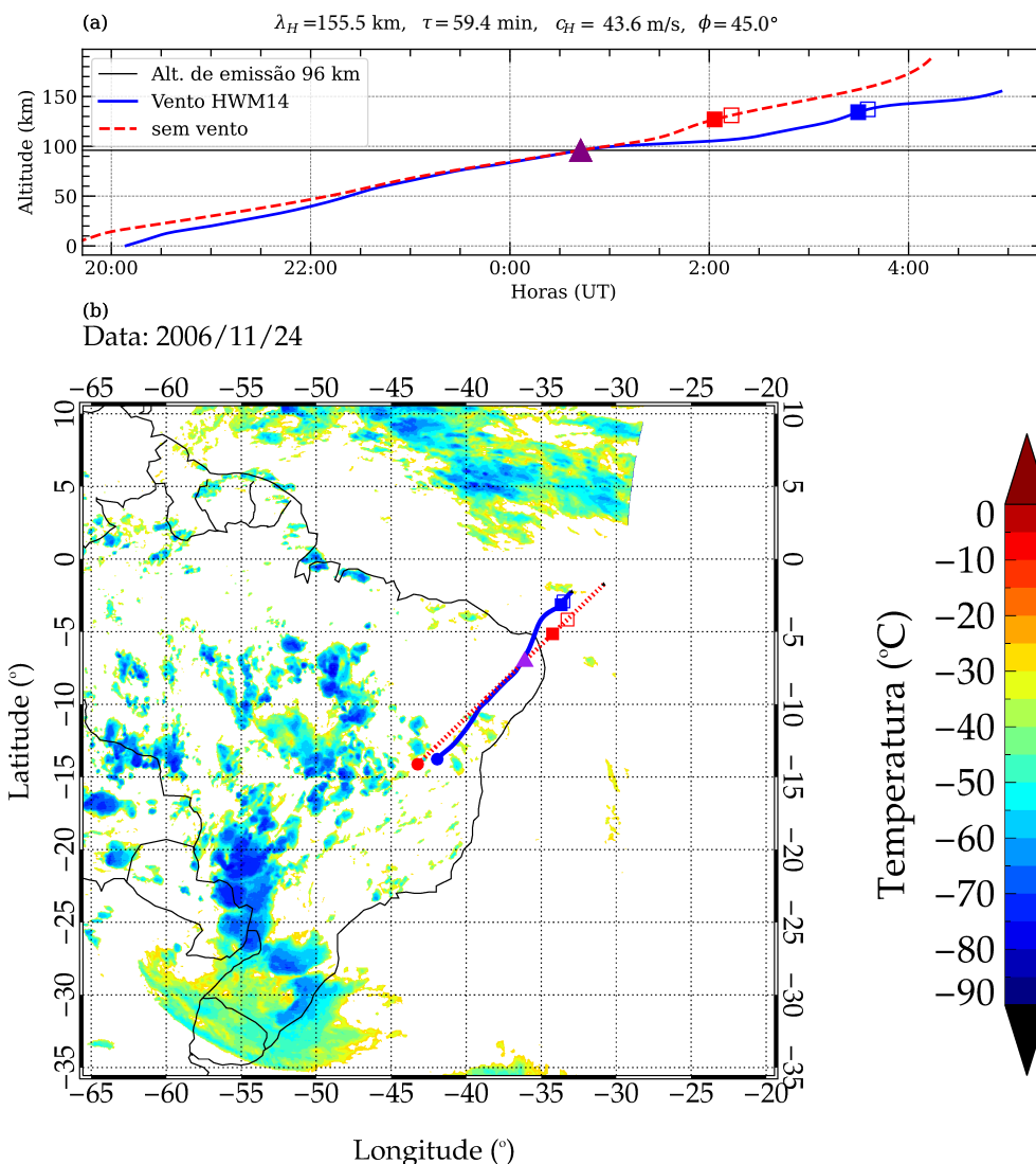
Figura 4.17 - Retrotrajetória da onda de gravidade de média escala, com propagação de fase descendente, em função do tempo, e sobre o mapa da temperatura de brilho do topo de nuvens às 19 h 30 min.
