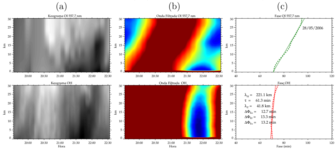
Figura A.22 - Onda de gravidade de média escala observada nas emissões do OI 557,7 nm e OH, na noite de 28/05/2006, em São João do Cariri (PB).
