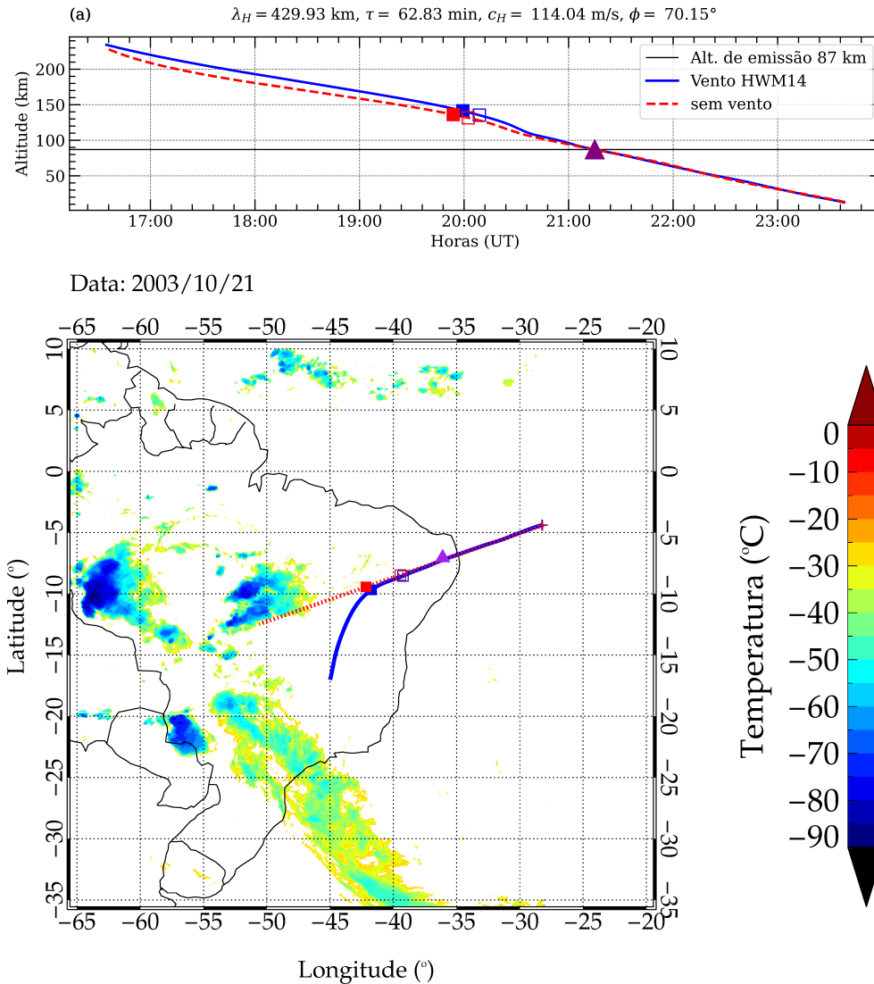
(a) Trajetória da onda de gravidade de média escala, com propagação de fase ascendente, em função do tempo. (b) Mapa do Brasil com a trajetória da onda de gravidade e a sobreposição da temperatura de brilho do topo de nuvens, obtidos pelo satélite GOES-12, para o dia 21 de outubro de 2003, às 23 h 30 min. Os quadrados preenchidos representam o fluxo de momentum máximo da onda (azul com vento modelado e vermelho sem vento). Os quadrados vazios representam os pontos da trajetória onde o fluxo de momentum é menor do que 10% do fluxo máximo.
