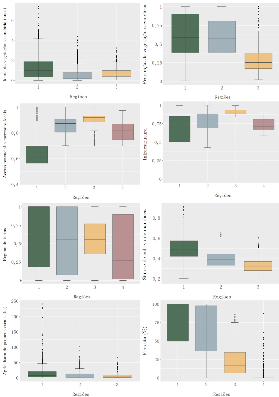
Figura 5.15 - Boxplot: indicadores e AGPE por região.
