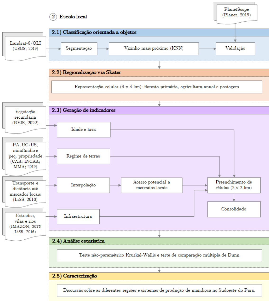
Figura 4.2 - Fluxograma: escala local.
