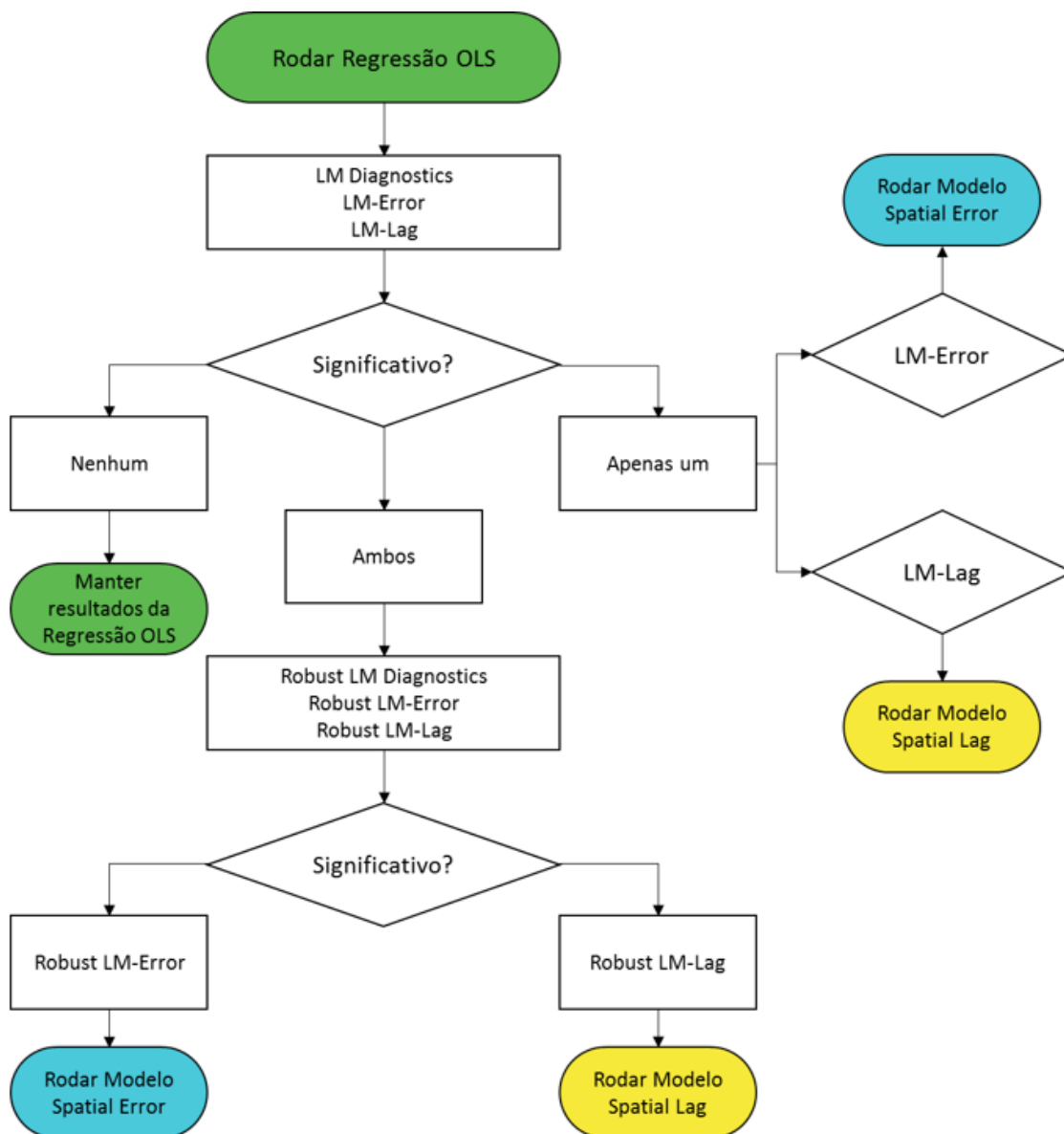
Figura 2.3 - Chave de decisão para escolha de modelo de regressão.
