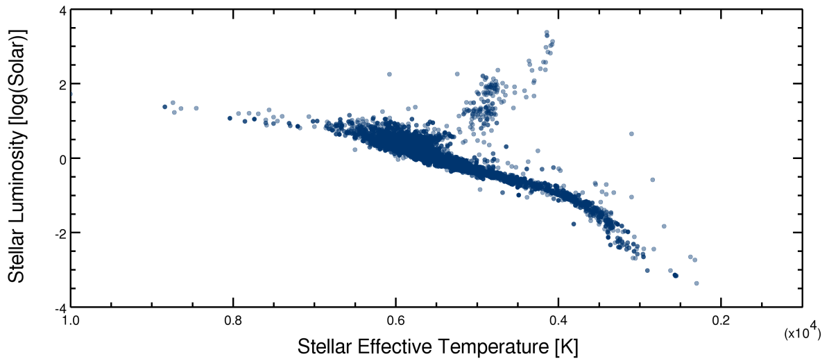
Figura 5.1 - Diagrama H-R das estrelas hospedeiras de planetas.
