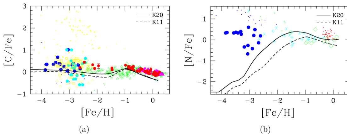
Figura 2.5 - [C/Fe] e [N/Fe] versus [Fe/H] para a vizinhança solar.
