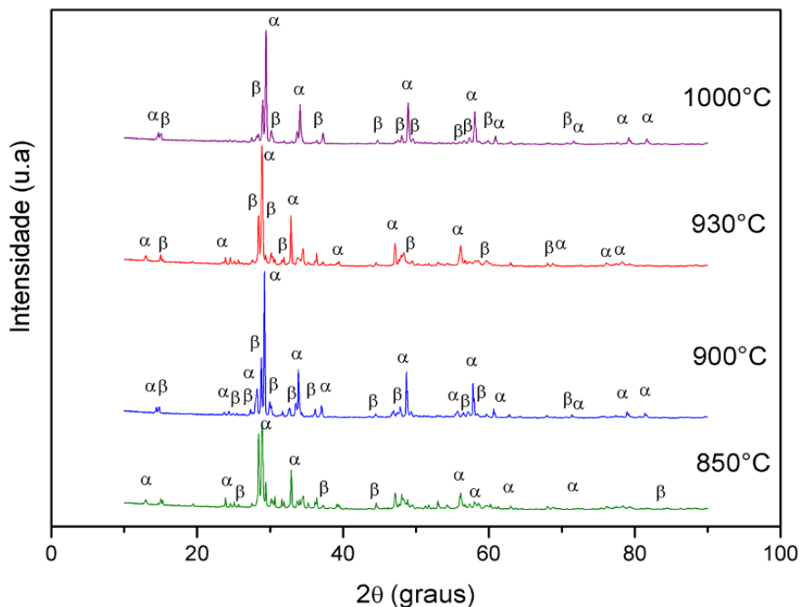
Figura 4.6 - Difratogramas do pó \alpha -BZN calcinados após 3h.
