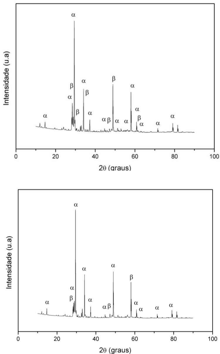
Figura 4.9 - Difratometria das amostras calcinadas por 3h a 1050°C: \alpha -BZN (a) 850°C; \alpha -BZN (b) 930°C.
