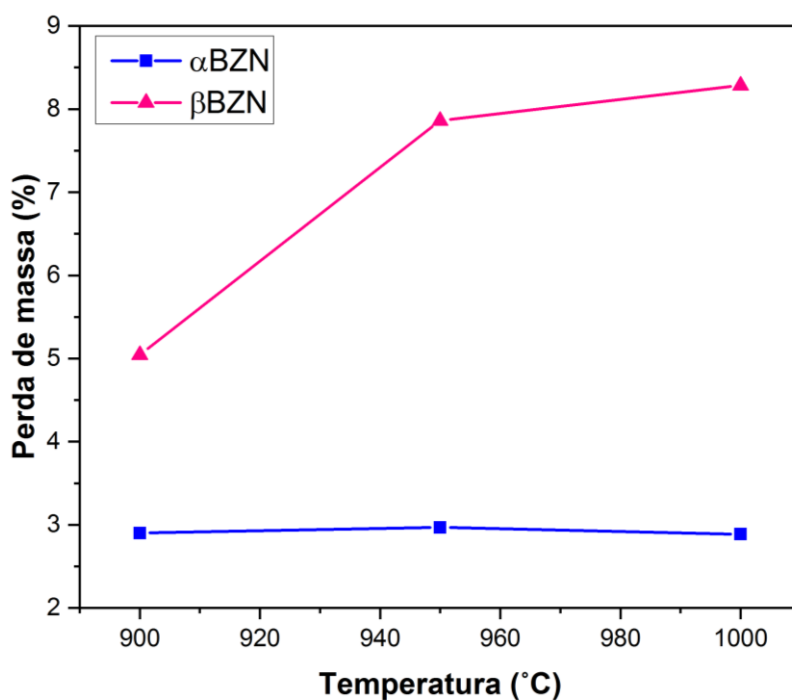
Figura 4.1 - Gráfico da perda de massa dos pós \beta e \alpha BZN em função da temperatura de calcinação.
