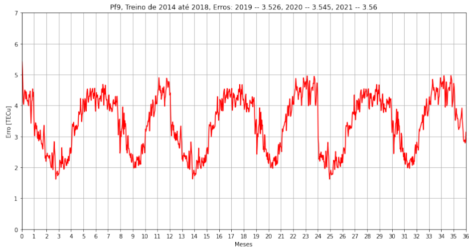
Figura 2.7 - RMSE para modelo linear treinado com dados de PF_9 de 2014-2018 e testado de 2019-2021.
