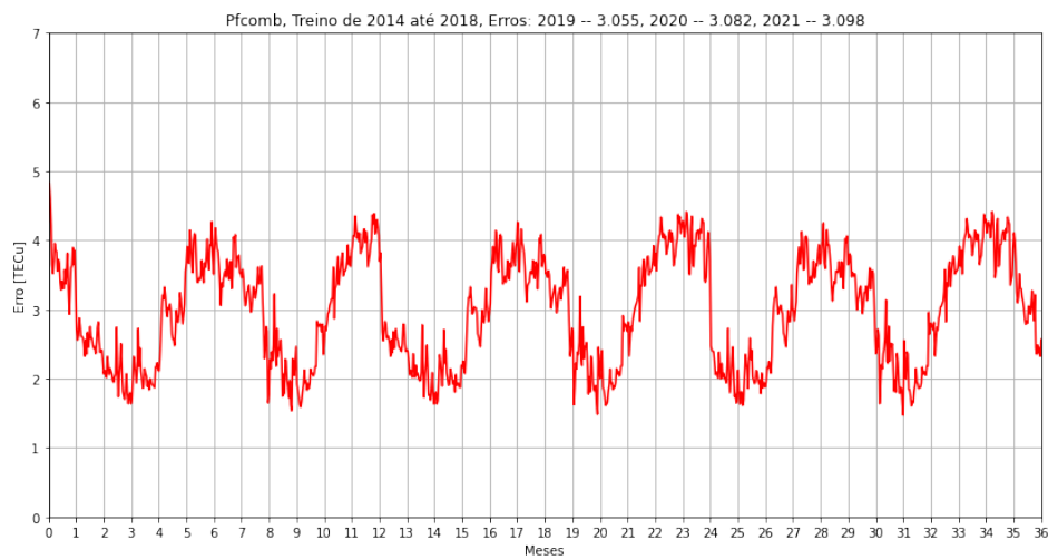
Figura 2.8 - RMSE para modelo linear treinado com dados de PF_{comb} de 2014-2018 e testado de 2019-2021.
