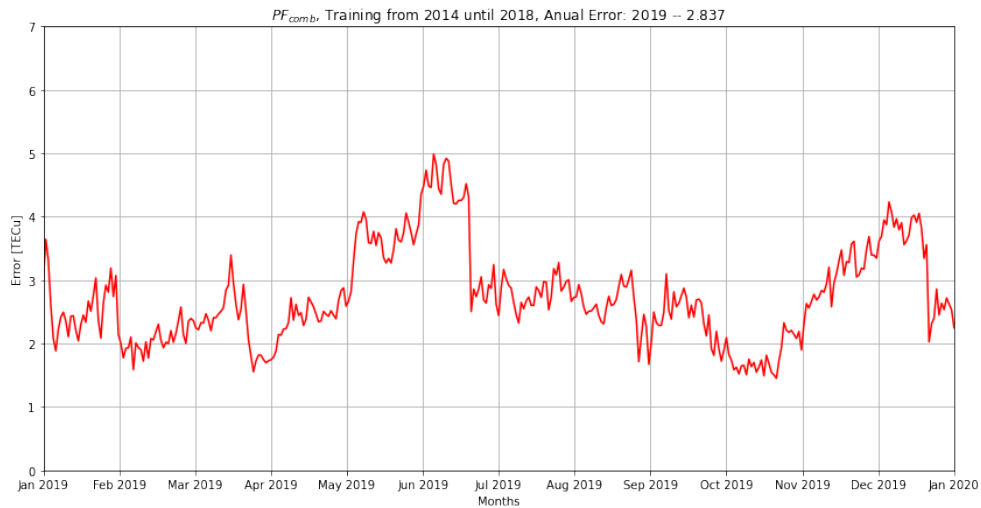
Figura 3.9 - Variação durante o ano de 2019 do RMSE para regressão linear, treino de 2014-2018 com PF_{comb} e divisão sazonal.
