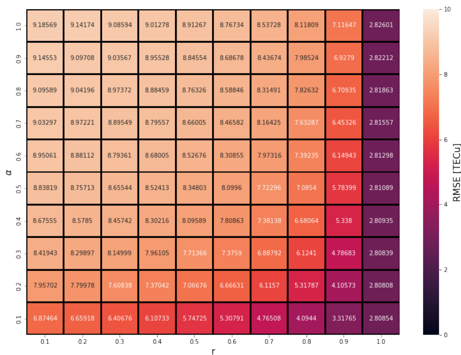
Figura 3.2 - Mapa de calor dos coeficientes de regularização do modelo linear para RSN, testado em 2021.
