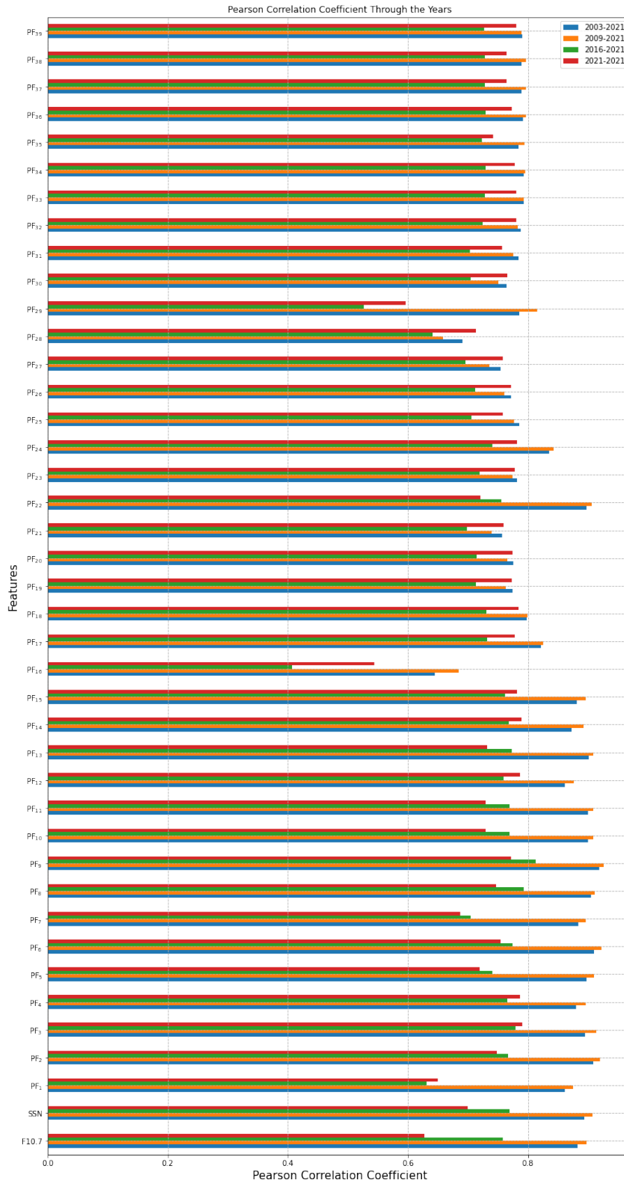
Figura 2.5 - Correlação entre o TEC médio diário e todas as features para diferentes períodos de tempo.
