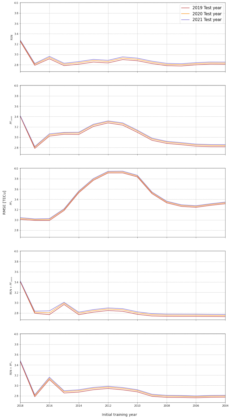
Figura 3.11 - Comparação entre RMSE para diferentes anos de teste, treino e conjuntos de features.
