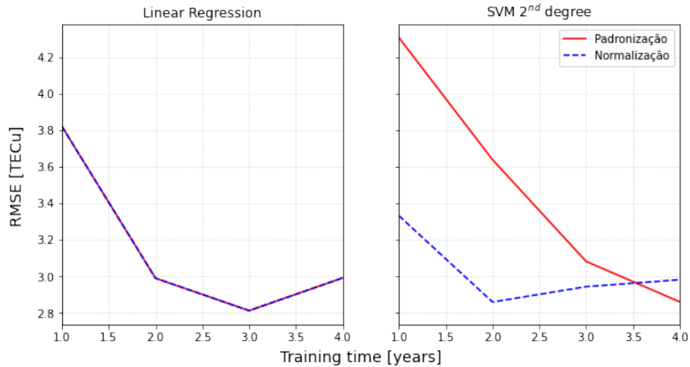
Figura 2.10 - Comparação do efeito da normalização e padronização no RMSE anual.
