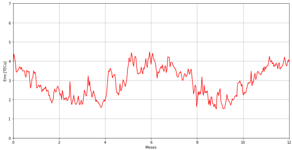
Figura 3.4 - Variação durante o ano do RMSE para modelo treino de 2014-2018 com RSN, F10.7 e PF_1 - PF_3 .
