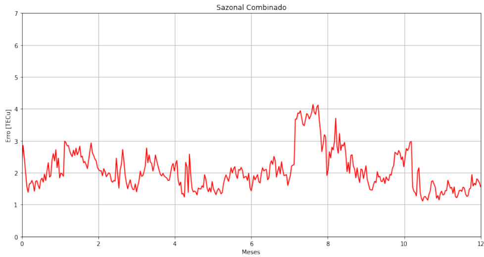
Figura 3.8 - Variação durante o ano de 2019 do RMSE para treino de 2014-2018 com RSN, F10.7 e PF_1 - PF_3 e divisão sazonal.
