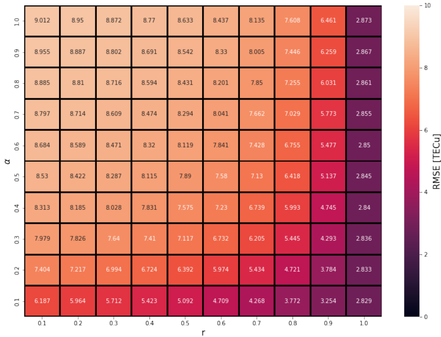
Figura 3.3 - Mapa de calor dos coeficientes de regularização do modelo linear para RSN e PF_{comb} , testado em 2021.
