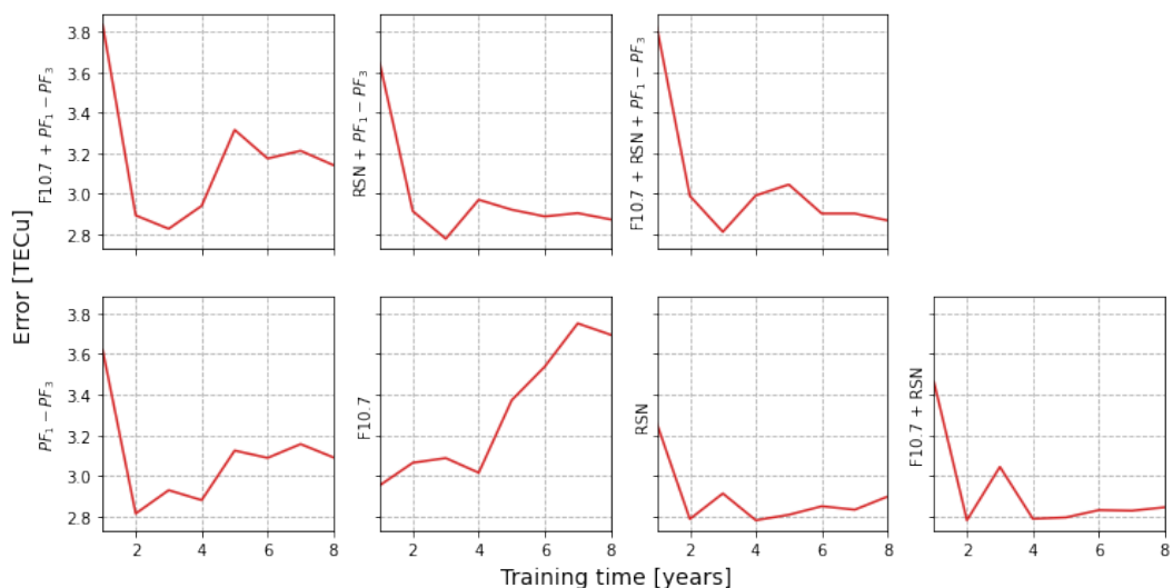
Figura 3.1 - Variação do RMSE conforme se aumenta o número de anos de treino começando em 2018, sendo o treino sempre em 2019.
