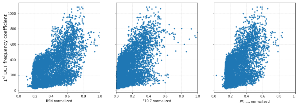
Figura 2.9 - Primeiro coeficiente de frequência após aplicação da DCT.
