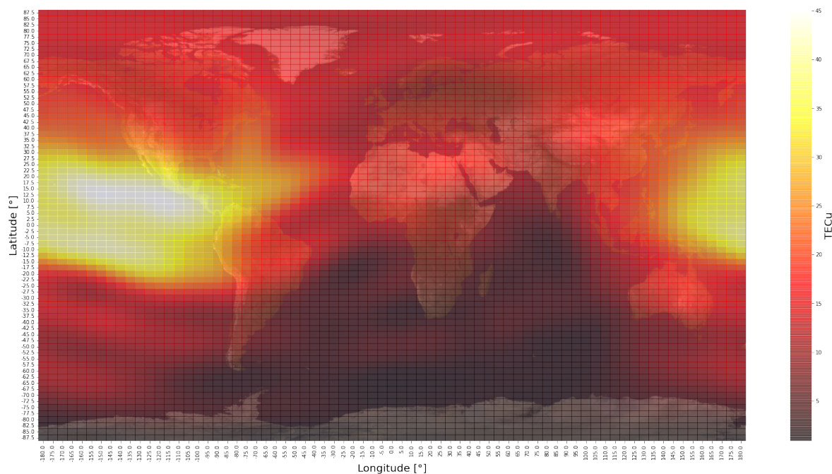
Figura 1.1 - Mapa de TEC para o dia 200 de 2009 às 08:00 UTC.
