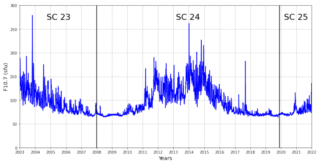
Figura 2.2 - Conjunto de dados de F10.7 obtidos para análise.
