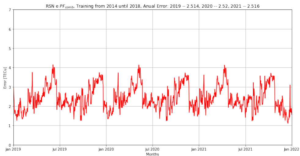
Figura 3.10 - Variação durante o ano de 2019, 2020 e 2021 do RMSE para regressão linear, treino de 2014-2018 com PF_{comb} e RSN e divisão sazonal.
