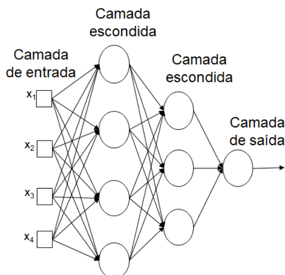
Figura 1 - Arquitetura de uma rede neural
