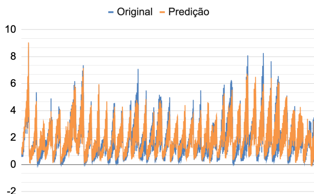
Figura 17 - Gráfico de Previsão x Alvo (Estratégia 2)
