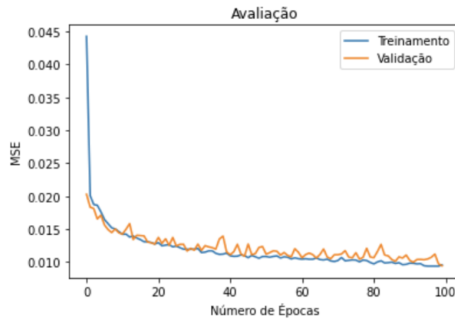
Figura 11 - Avaliação do modelo de previsão (Estratégia 1)
