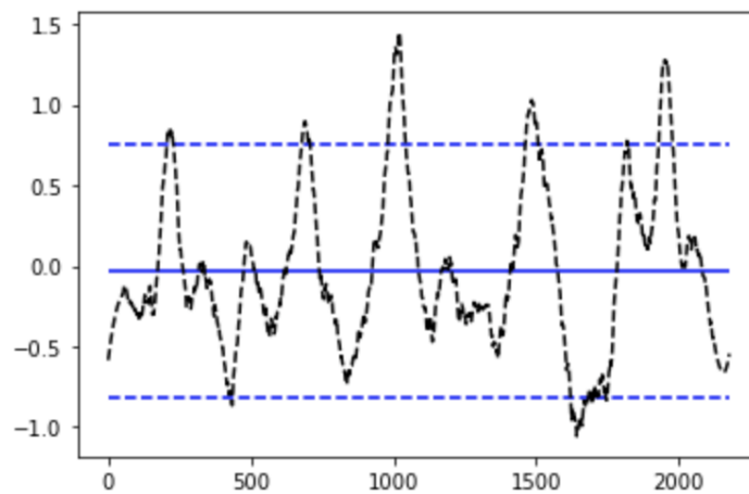
Figura 12 - Erro de saída esperada x previsão (Estratégia 1)
