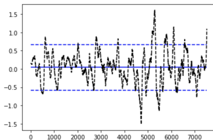
Figura 16 - Erro de saída esperada x previsão (Estratégia 2)
