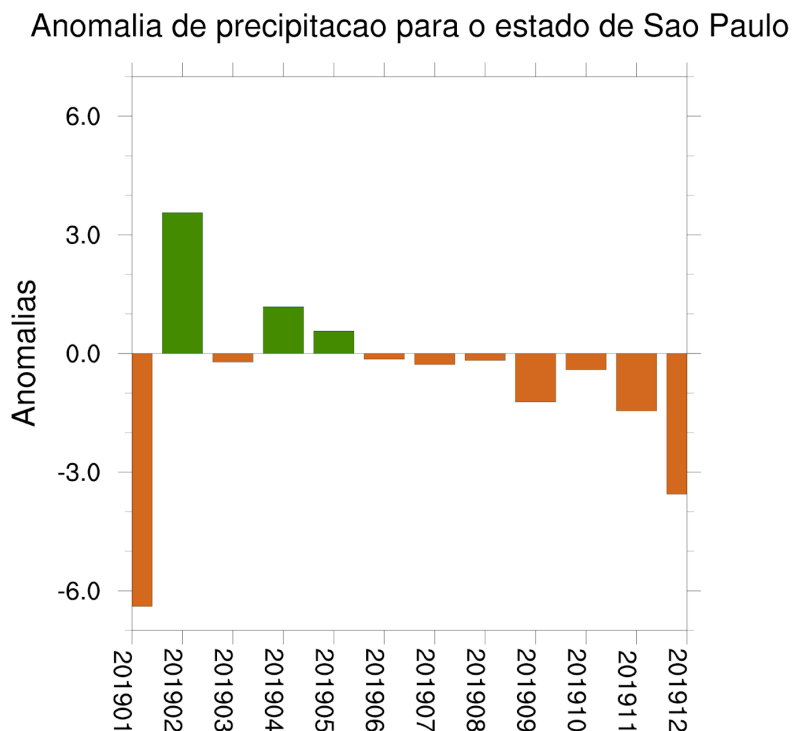
Figura 10 - Anomalia de precipitação (mm/dia) do ano de 2019 para o estado de São Paulo
