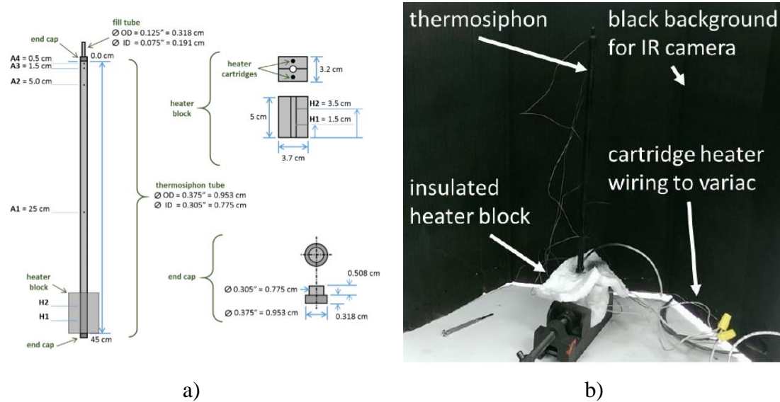
Figura 5- Termosifões: a) Desenho esquemático; b) imagem do sistema real,
