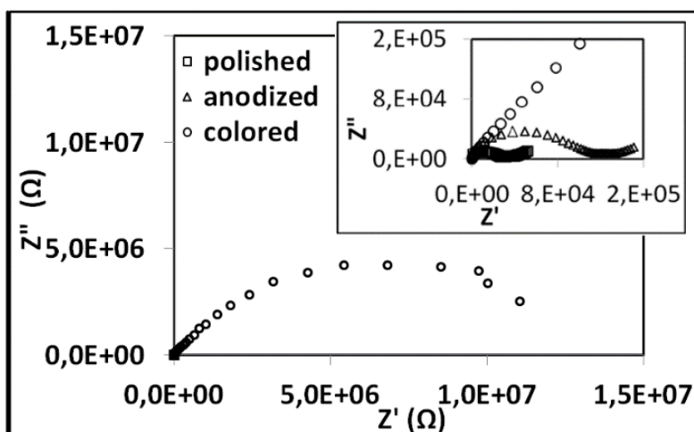
Figura 20- Resultados de impedância eletroquímica da amostra em alumínio 6061 anodizada em ácido sulfúrico a 90g/l por 40min e colorida.
