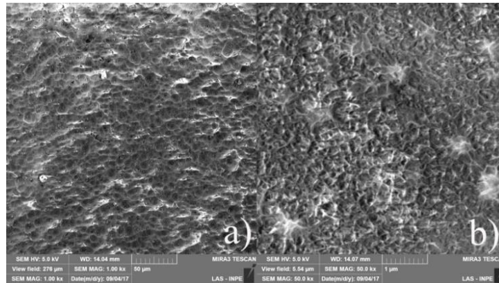
Figura 24 : Camada anodizada e colorida observada por MEV.
