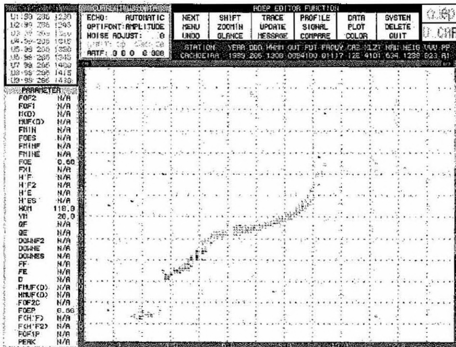
FIGURA 2.1 - Ionograma
