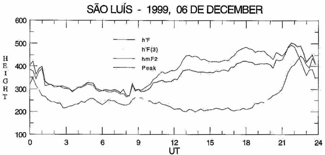
FIGURA 2.2 - Gráfico dos parâmetros h'F, h'F(3), hmF2, Peak.
