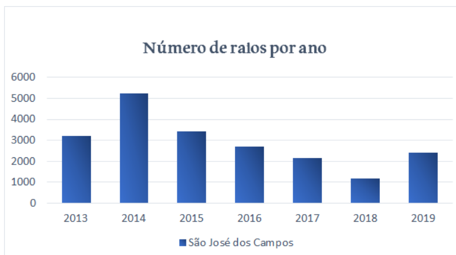
Figura 6 - Quantidade de descargas atmosféricas anuais no município de São José dos Campos.
