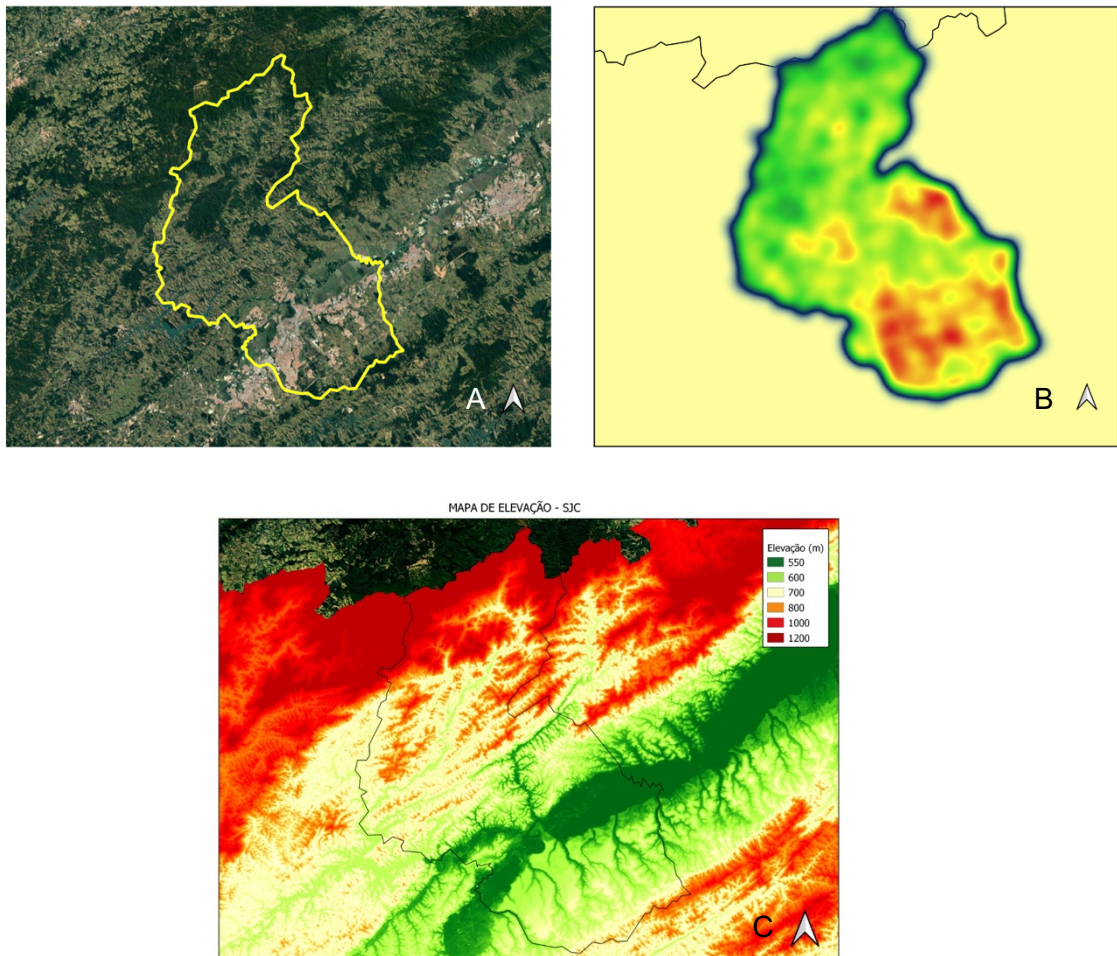
Figura 8- a) Mapa de áreas impermeáveis no município de São José dos Campos. b) Mapa da concentração de descargas atmosféricas no município de São José dos Campos. c) Mapa de elevação no município de São José dos Campos.
