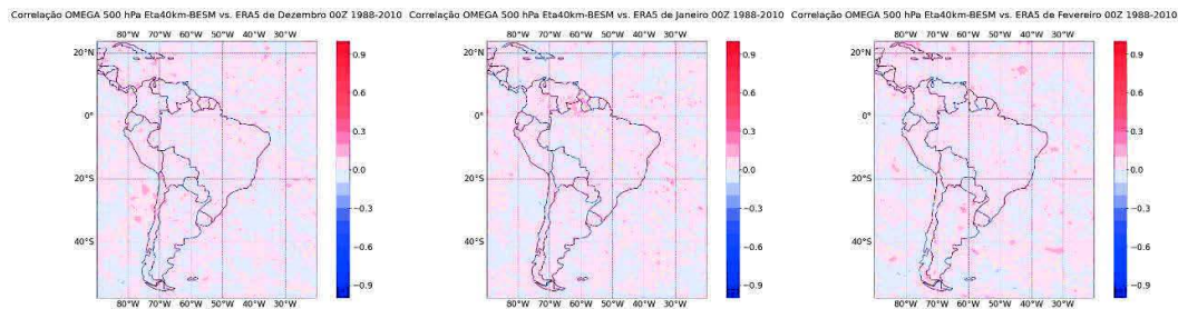
Figura 4.24 - Coeficientes de correlação entre as previsões de movimento vertical a 500 hPa do Eta40km-BESM e valores observados pelo ERA5, para os meses de dezembro, janeiro e fevereiro do período de 1988-2010.
