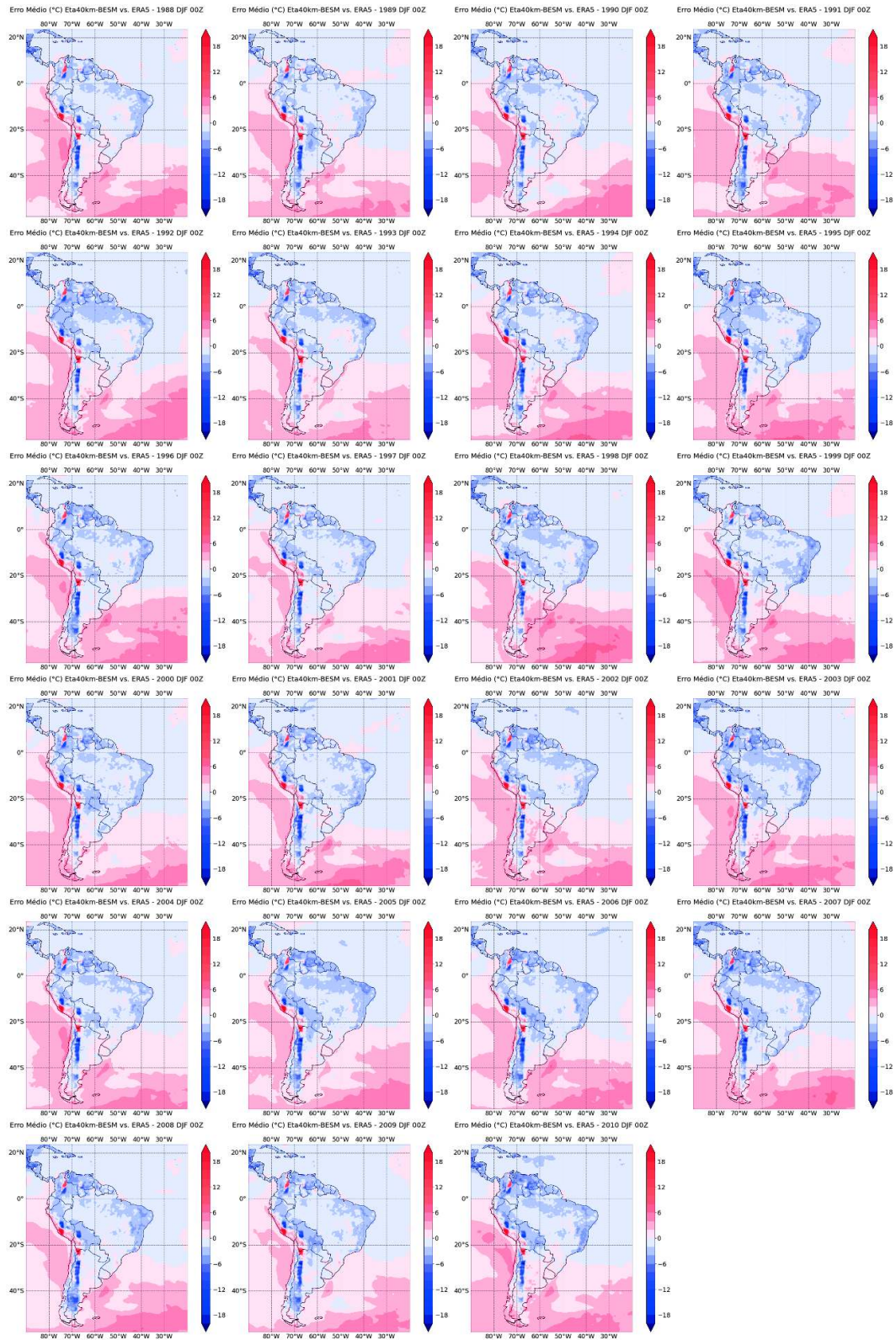
Figura 4.8 – Erro médio de temperatura do ar a 2m (°C) das previsões do Eta40km-BESM, para o período de dezembro, janeiro e fevereiro (DJF) dos anos de 1988 até 2010.
