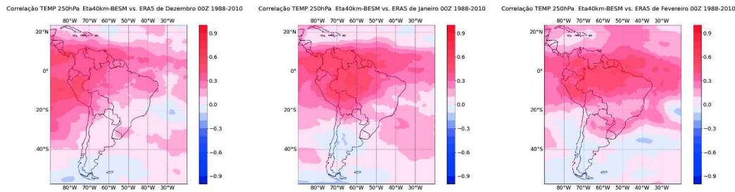
Figura 4.18 - Coeficientes de correlação entre as previsões de temperatura do ar a 250 hPa do Eta40km-BESM e valores observados pelo ERA5, para os meses de dezembro, janeiro e fevereiro do período de 1988-2010, exceto 1991 e 2010.
