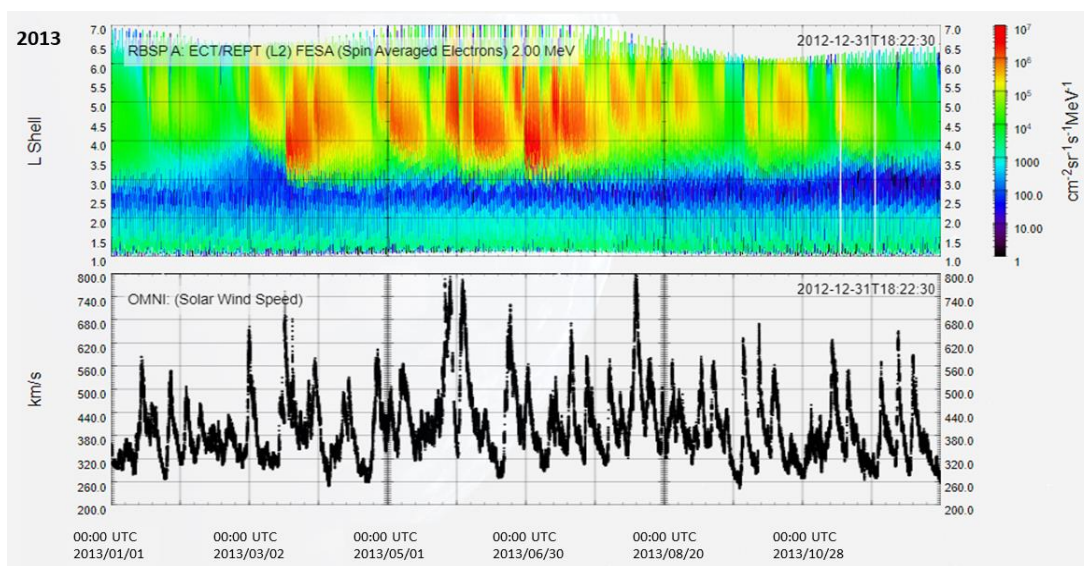
Figura 4.28 - Medida de fluxo de elétrons com energia de 2,00 MeV e medida de velocidade do vento solar em 2013.
