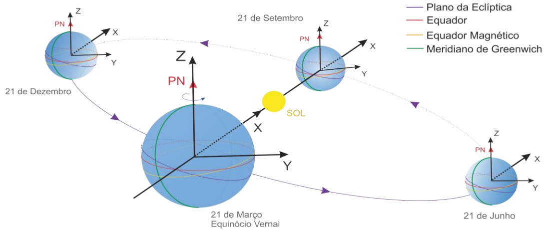
Figura 2.13 - Representação do Sistema de coordenadas GEI.
