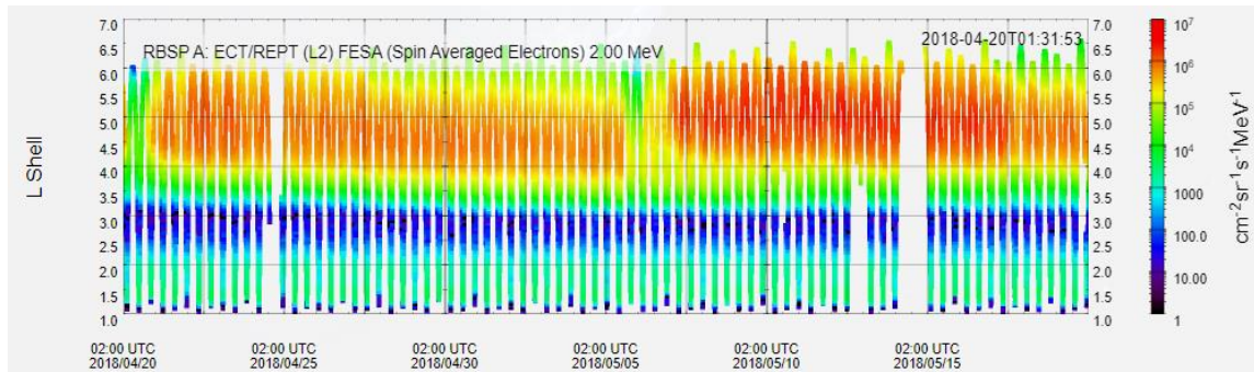
Figura 2.12 - Medida de fluxo de elétrons com energia de 2,00 MeV durante 1 mês. No eixo Y é mostrado a localização da partícula a partir do L-Shell, no eixo x indica a data e a legenda no lado direito indica a intensidade do fluxo.
