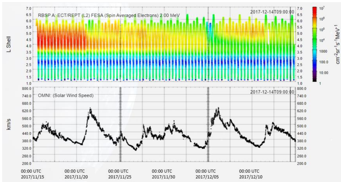
Figura 4.27 - Medida de fluxo de elétrons com energia de 2,00 MeV e medida de velocidade do vento solar entre 15/11/2017 e 15/12/2017.
