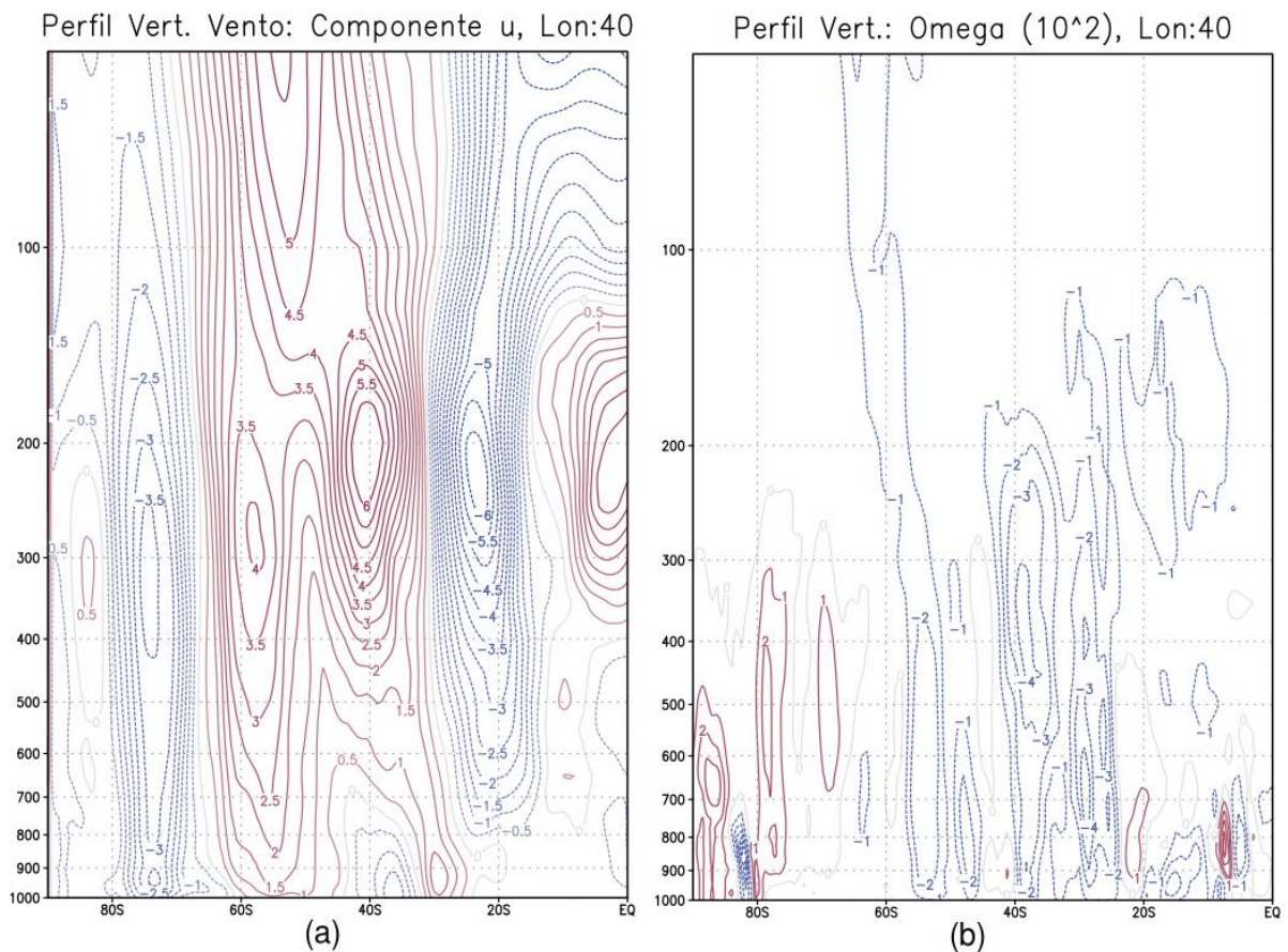
Figura 4.15: Composto de Perfil Vertical para SAM positivo, La Niña - Máxima extensão de gelo marinho no MBA: a) anomalia do vento zonal ( m.s^{-1} ); b) ômega ( 10^2 Pa.s^{-1} ).
