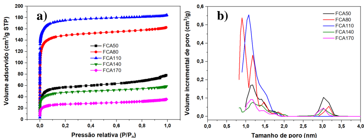
Figura 6.1 – a) Isotermas de N 2 a 77K e b) distribuição de tamanhos de poro por NLDFT.
