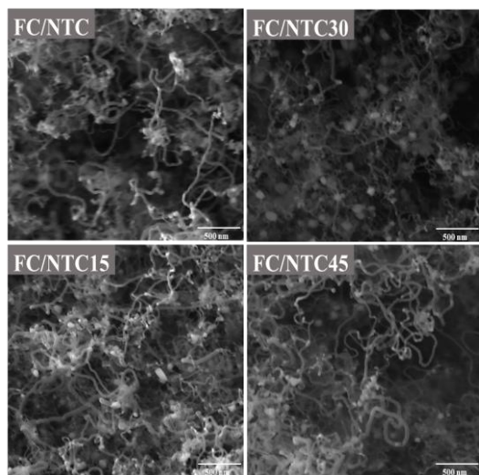
Fig. 1 – Micrografia das amostras antes e após os processos oxidativos.
