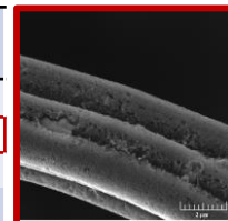
Fig. 3 – Superfície exposta de um monofilamento da FC após tratamento de ativação da amostra FC/NTC15.
