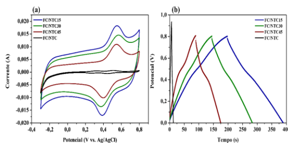
Fig. 2 – (a) Voltamogramas e (b) curvas de carga e descarga das amostras FC/NTC antes e após o processo oxidativo.
