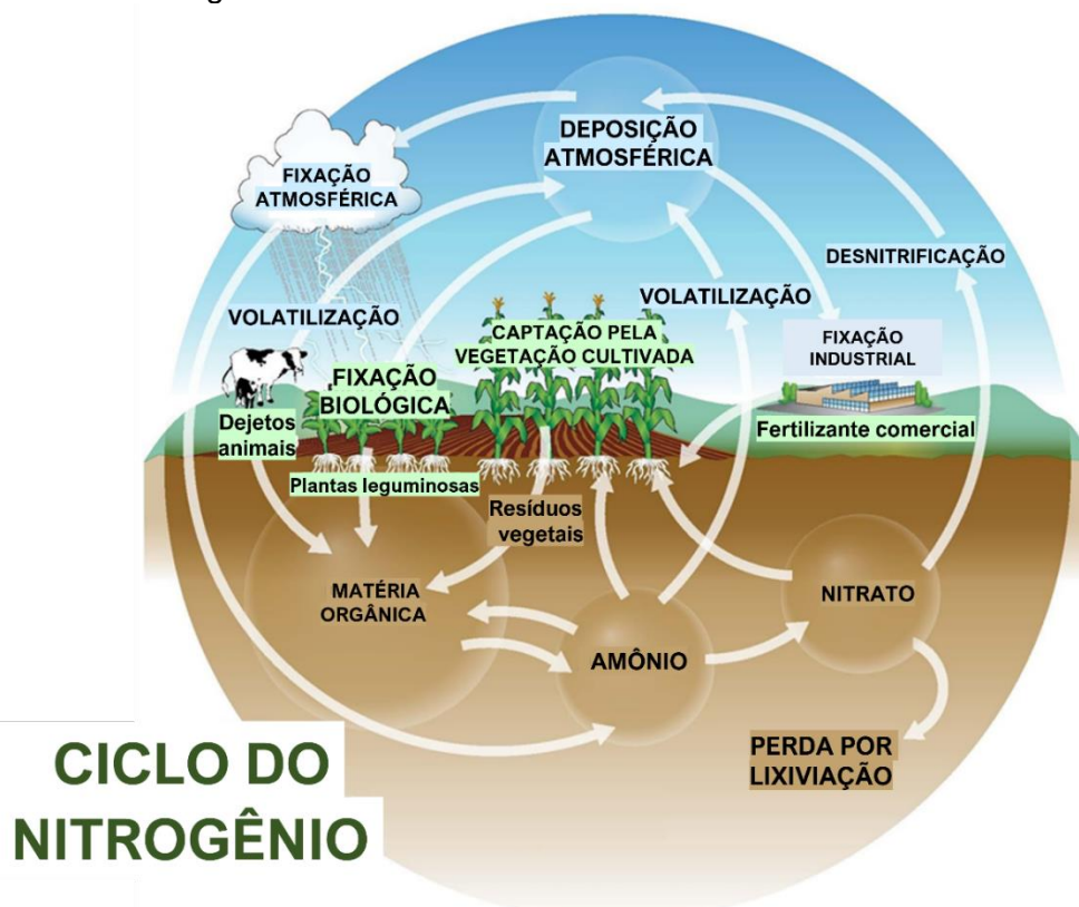
Figura 2.1 - Esquema simplificado dos principais processos que governam a ciclagem do nitrogênio.
