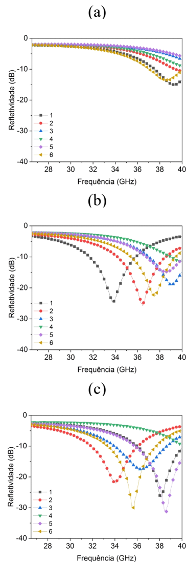
Fig. 10. Refletividade das amostras com concentrações de FC de (a) 50%, (b) 60% e (c) 70% para a banda Ka.
