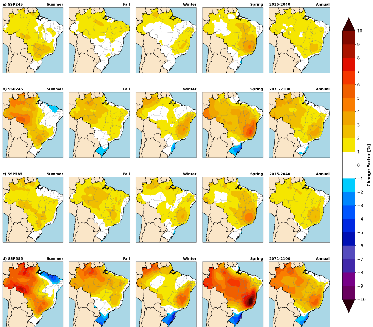
Figura 5 - O fator de mudança na SSR sazonal previsto pelo SME no SSP2-4.5 (primeiras duas linhas) e SSP5-8.5 (últimas duas linhas) para os períodos de 2015-2040 (linhas ímpares) e 2071-2100 (linhas pares). As estações do ano estão apresentadas sequencialmente da esquerda para a direita: verão, outono, inverno e primavera. A coluna mais à direita apresenta a média anual do CCF.
