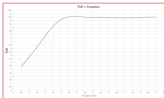
Figura 2: Permissividade efetiva em função da frequência utilizada
