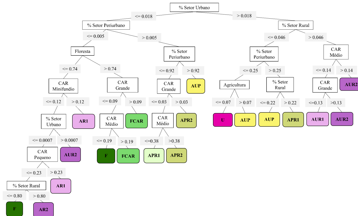
Figura B. 1 – Exemplo de uma das árvores de decisão com menor ocorrência de erro na avaliação dos dados de teste.
