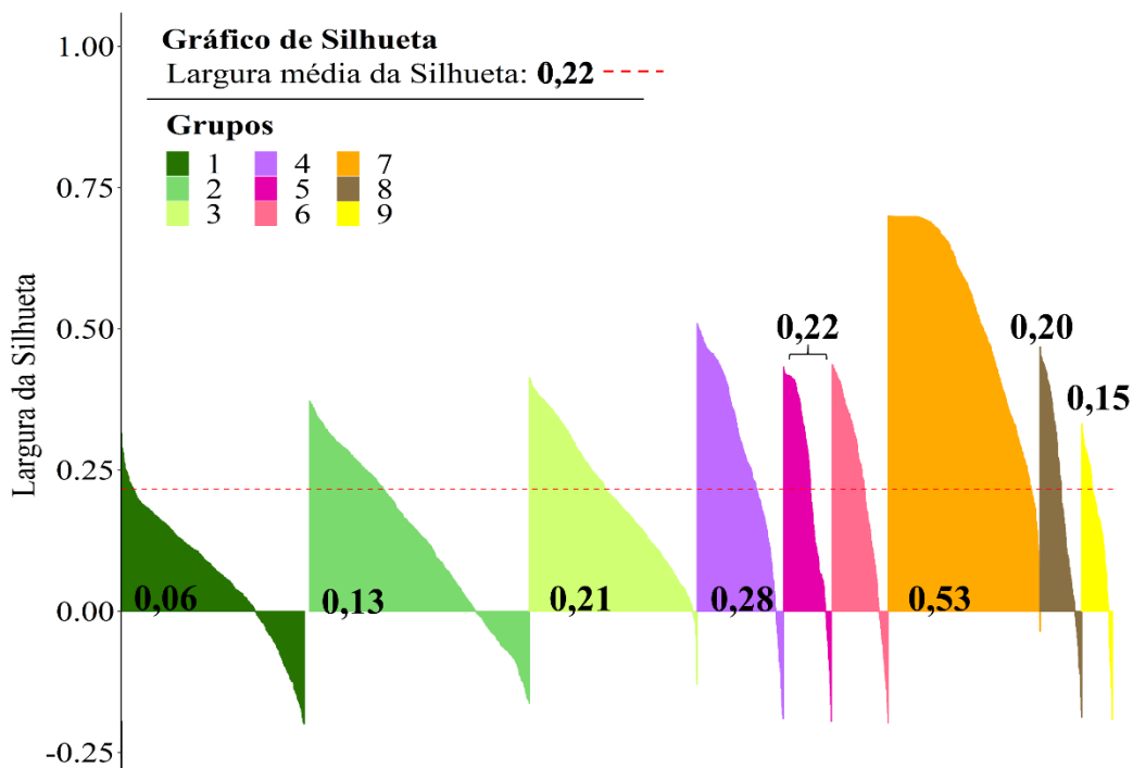
Figura 4.2 - Gráfico de silhueta - Avaliação dos grupos formados.
