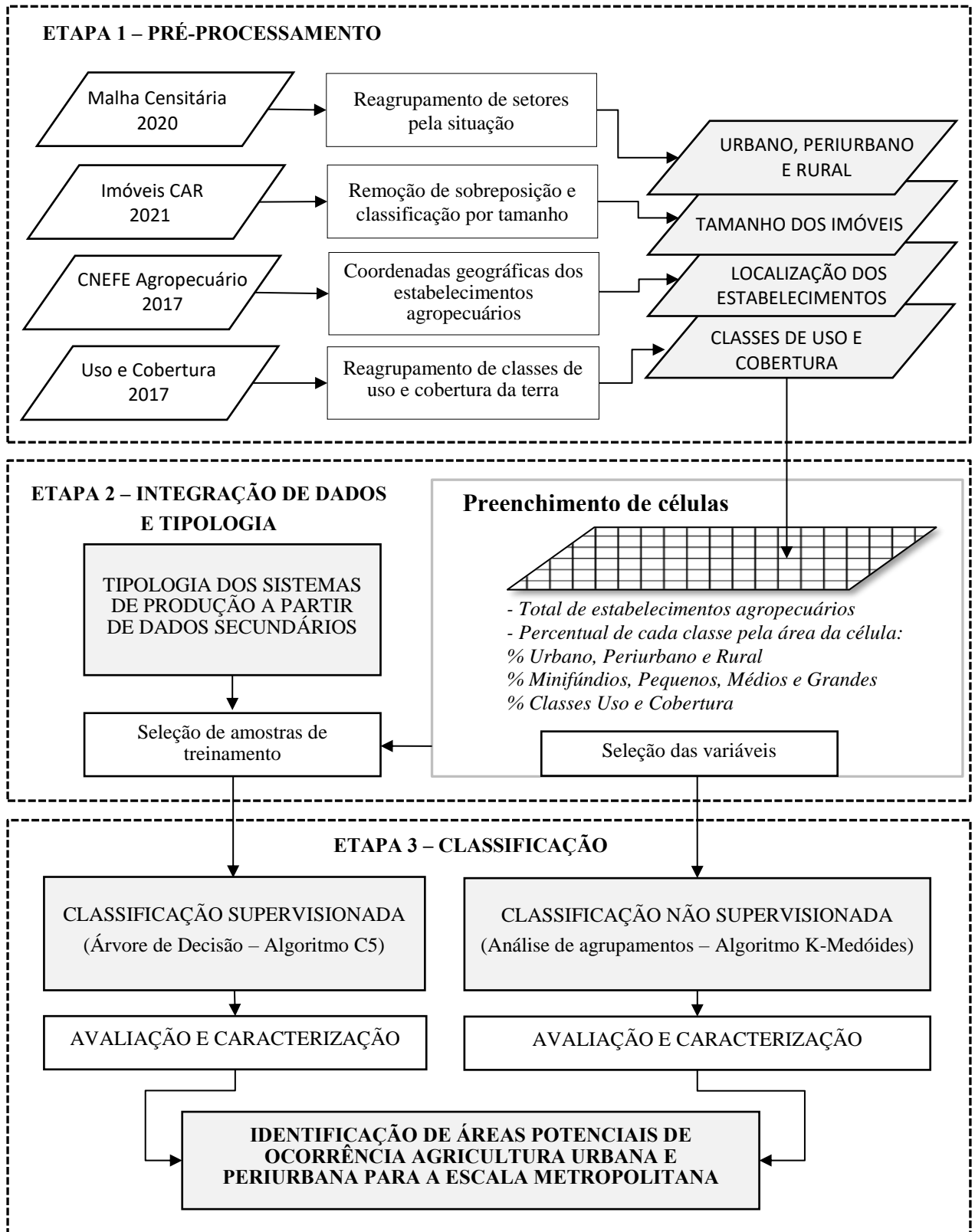
Figura 3.3 - Diagrama metodológico geral com as etapas da pesquisa.
