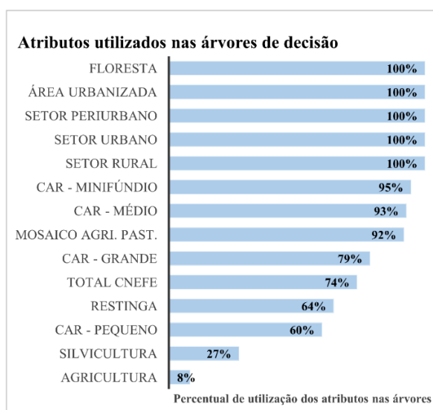
Figura 4.3 - Atributos utilizados nas árvores de decisão.
