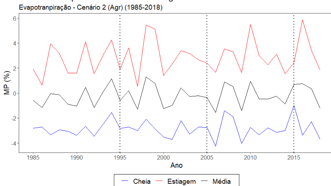
Figura H.3 – Mudança percentual para o cenário 2 para a evapotranspiração médias e em períodos de cheia e estiagem.
