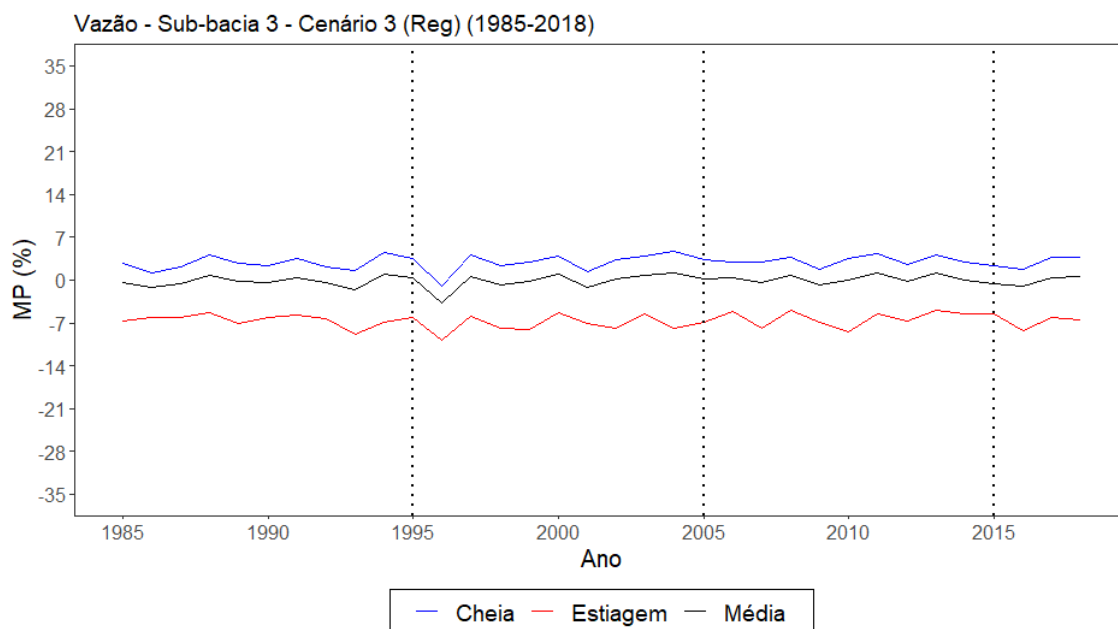
Figura G.15 – Mudança percentual para cenário 3 para as vazões médias, máximas e mínimas da sub-bacia 3.
