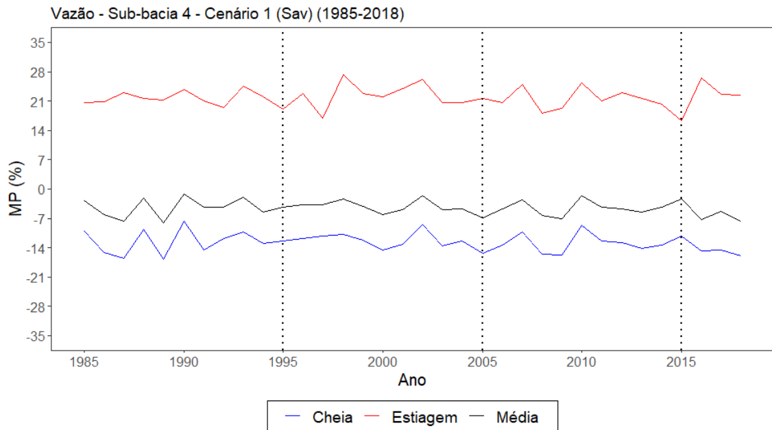
Figura G.8 – Mudança percentual para cenário 1 para as vazões médias, máximas e mínimas da sub-bacia 4.
