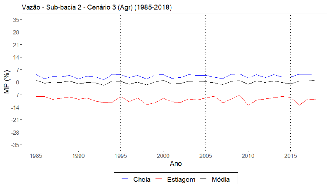
Figura G.14 – Mudança percentual para cenário 3 para as vazões médias, máximas e mínimas da sub-bacia 2.
