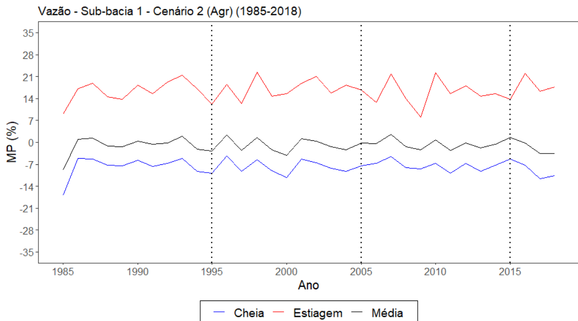
Figura G.9 – Mudança percentual para cenário 2 para as vazões médias, máximas e mínimas da sub-bacia 1.
