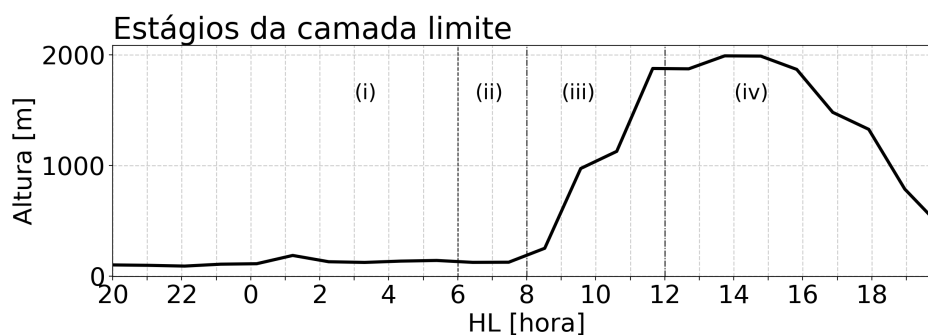
Figura 3.9 - Evolução horária da altura da Camada Limite Atmosférica estimada pelo ceilometer para um dia com pouca cobertura de nuvens (23/08/2015). As fases referem-se ao (i) estágio estável da CLA noturna ; (ii) estágio de transição matutina; (iii) o estágio de rápido crescimento da CLA convectiva; (iv) o estágio da camada de mistura com nuvens convectivas.
