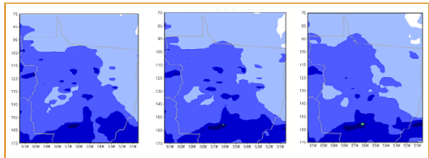
Figura 3.3: (a) fumaça ( \mu\text{g}/\text{m}^2 ), (b) PM2.5 ( \mu\text{g}/\text{m}^3 ) e (c) AOT no Estado de Roraima referente ao dia 28 de janeiro de 2018. As variáveis são estimadas pelo modelo regional BRAMS.
