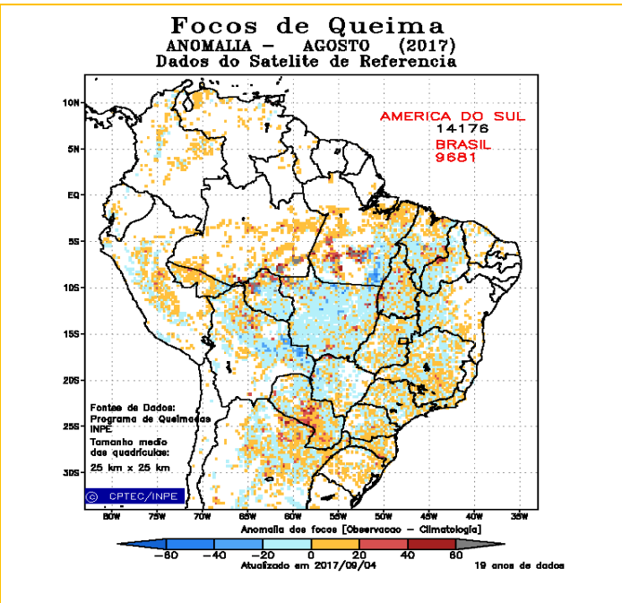
Mapa 2.2 – Anomalia de detecções registradas em Agosto/2017 segundo o satélite referência.
